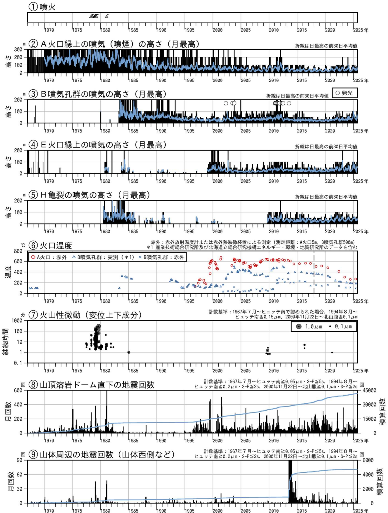
図1 樽前山 火山活動経過図（1967年1月～2025年9月）
