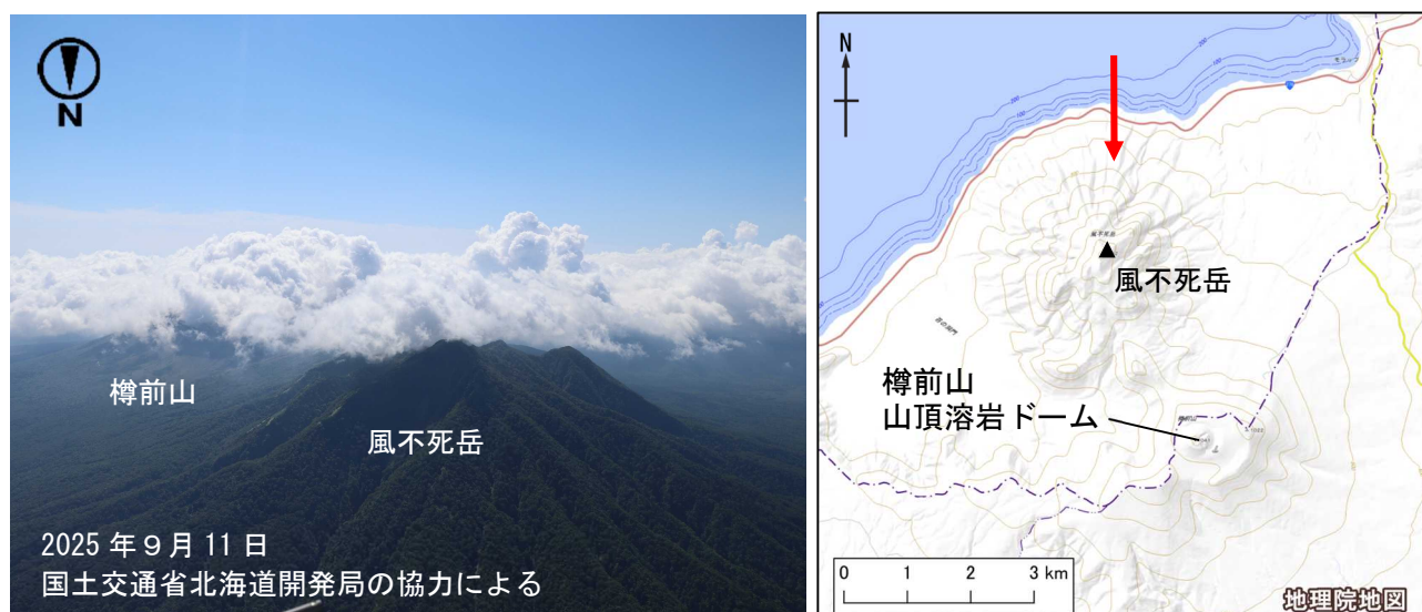
図3 樽前山 北側上空からの風不死岳付近の状況（右図の赤矢印方向から撮影）
