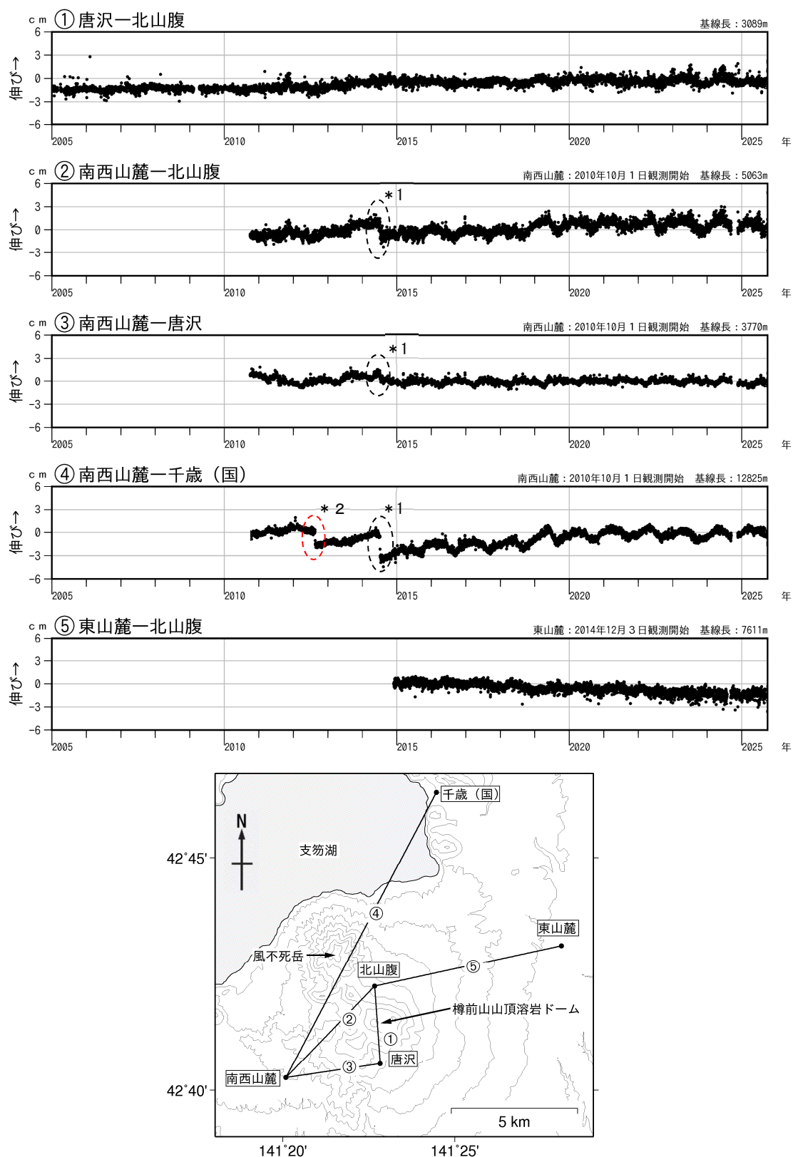
図5 樽前山 GNSS連続観測による基線長変化（2005年1月～2025年9月）及び観測点配置図 グラフ①～⑤は観測点配置図の基線①～⑤に対応しています。
