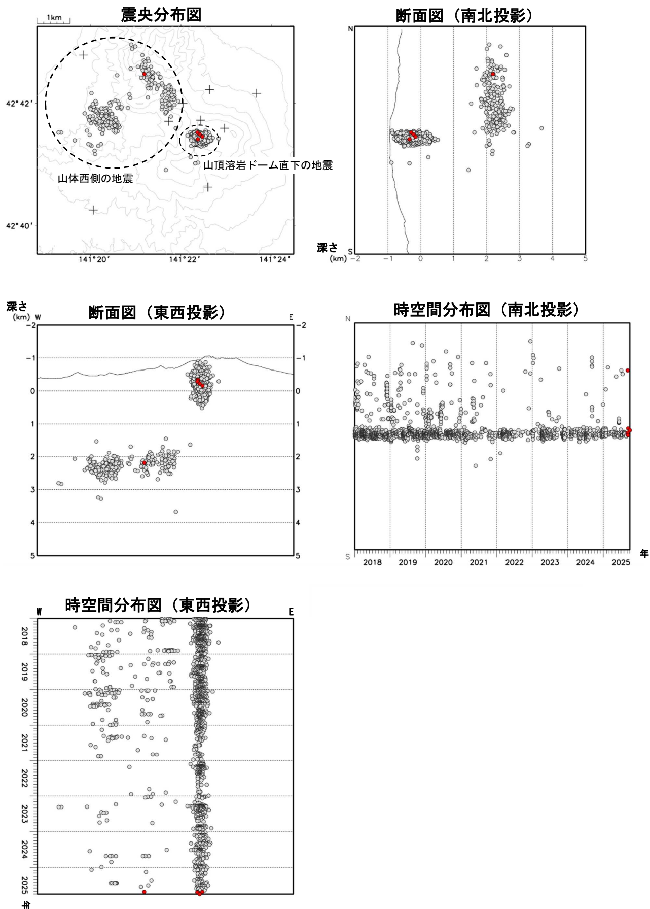
図4 樽前山 火山性地震の震源分布（2018年1月～2025年9月）
