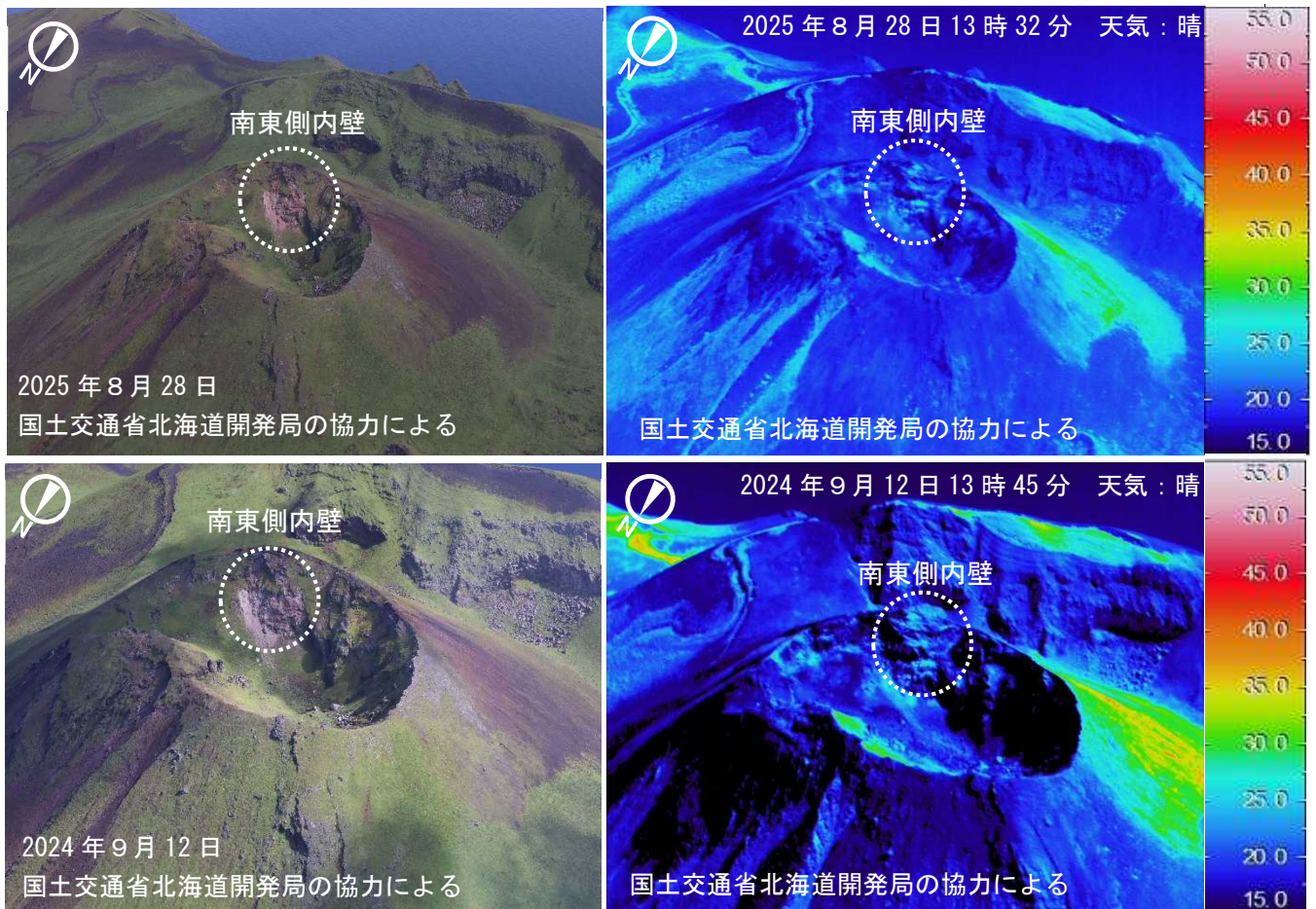
図3 渡島大島 赤外熱映像装置による寛保岳火口内の地表面温度分布
