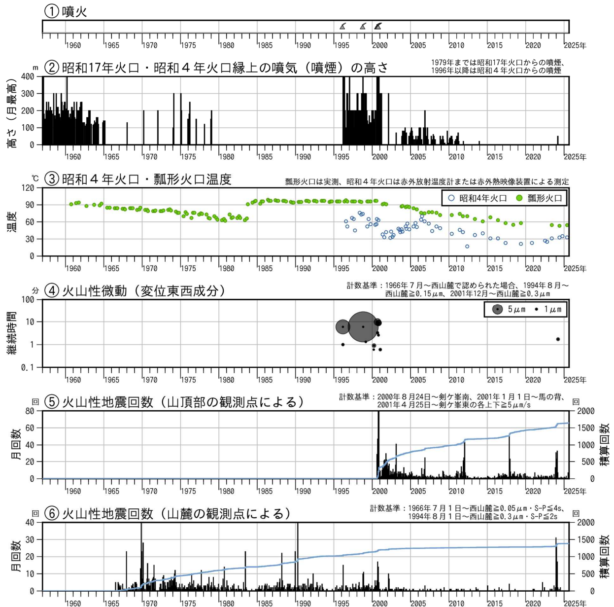
図1 北海道駒ヶ岳 火山活動経過図（1957年1月～2025年8月） 各火口の位置は図10を参照してください。
