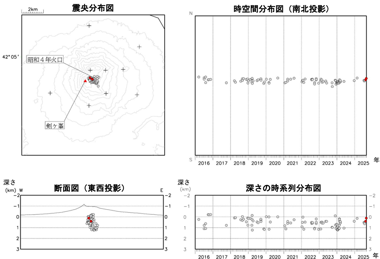
図6 北海道駒ヶ岳 火山性地震の震源分布（2016年1月～2025年8月）
