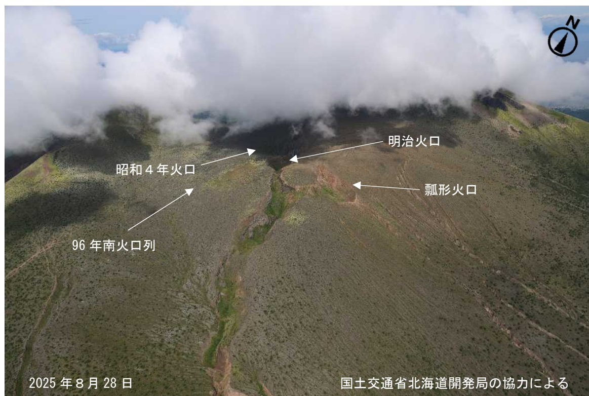
図4 北海道駒ヶ岳 山頂火口原の状況（図3の①から撮影）
