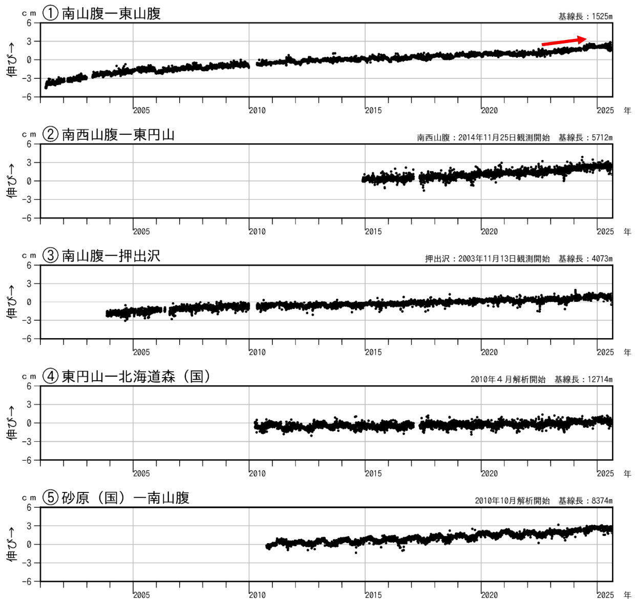
図7 北海道駒ヶ岳 GNSS連続観測による基線長変化（2001年4月～2025年8月）
