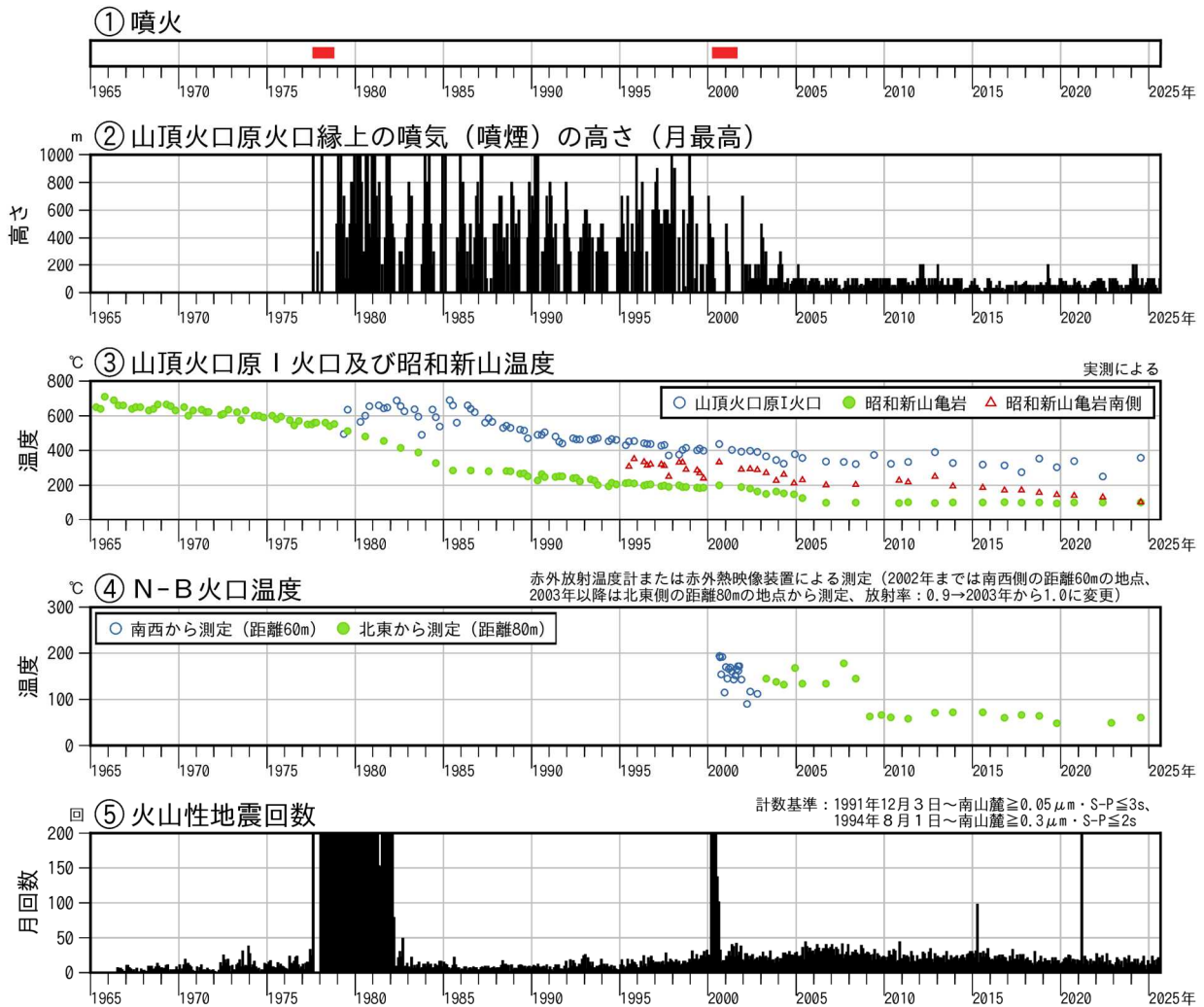
図1 有珠山 火山活動経過図（1965年1月～2025年8月）
