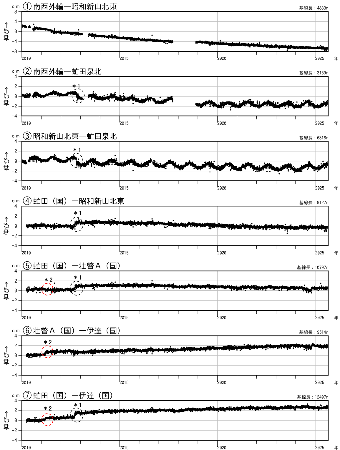
図4 有珠山 GNSS連続観測による基線長変化（2010年1月～2025年8月）
