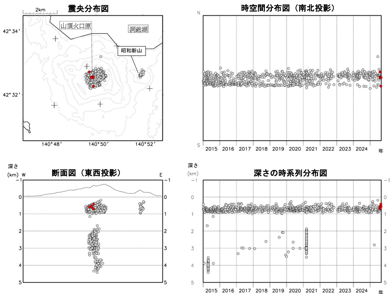
図3 有珠山 火山性地震の震源分布（2015年1月～2025年8月）
