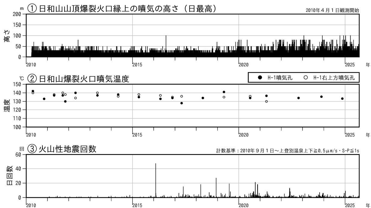
図 2 倶多楽 火山活動経過図（2010年 1 月～2025年 8 月）
