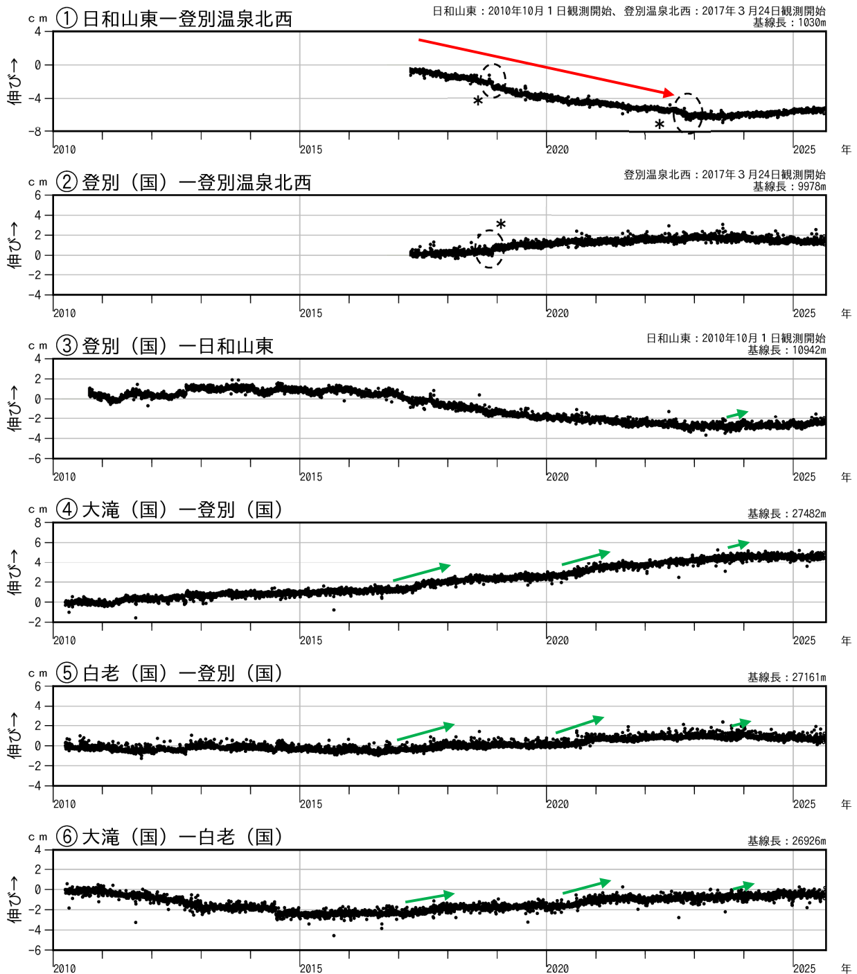
図3 倶多楽 GNSS連続観測による基線長変化（2010年4月～2025年8月）
