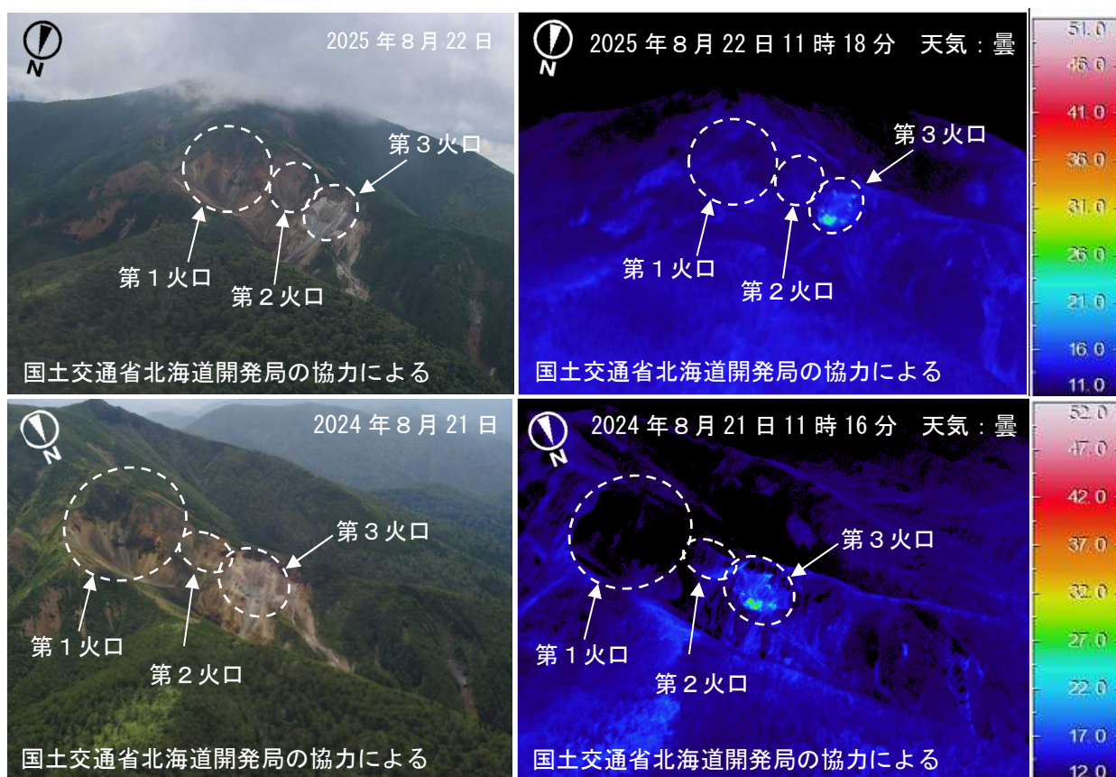
図3 丸山 赤外熱映像装置による山頂付近及び北側の火口列の地表面温度分布
