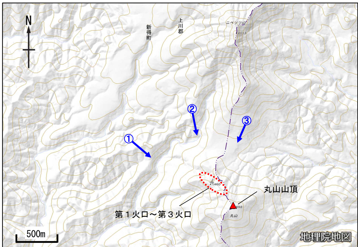
図1 丸山 赤外熱映像及び写真の撮影方向（青矢印）
