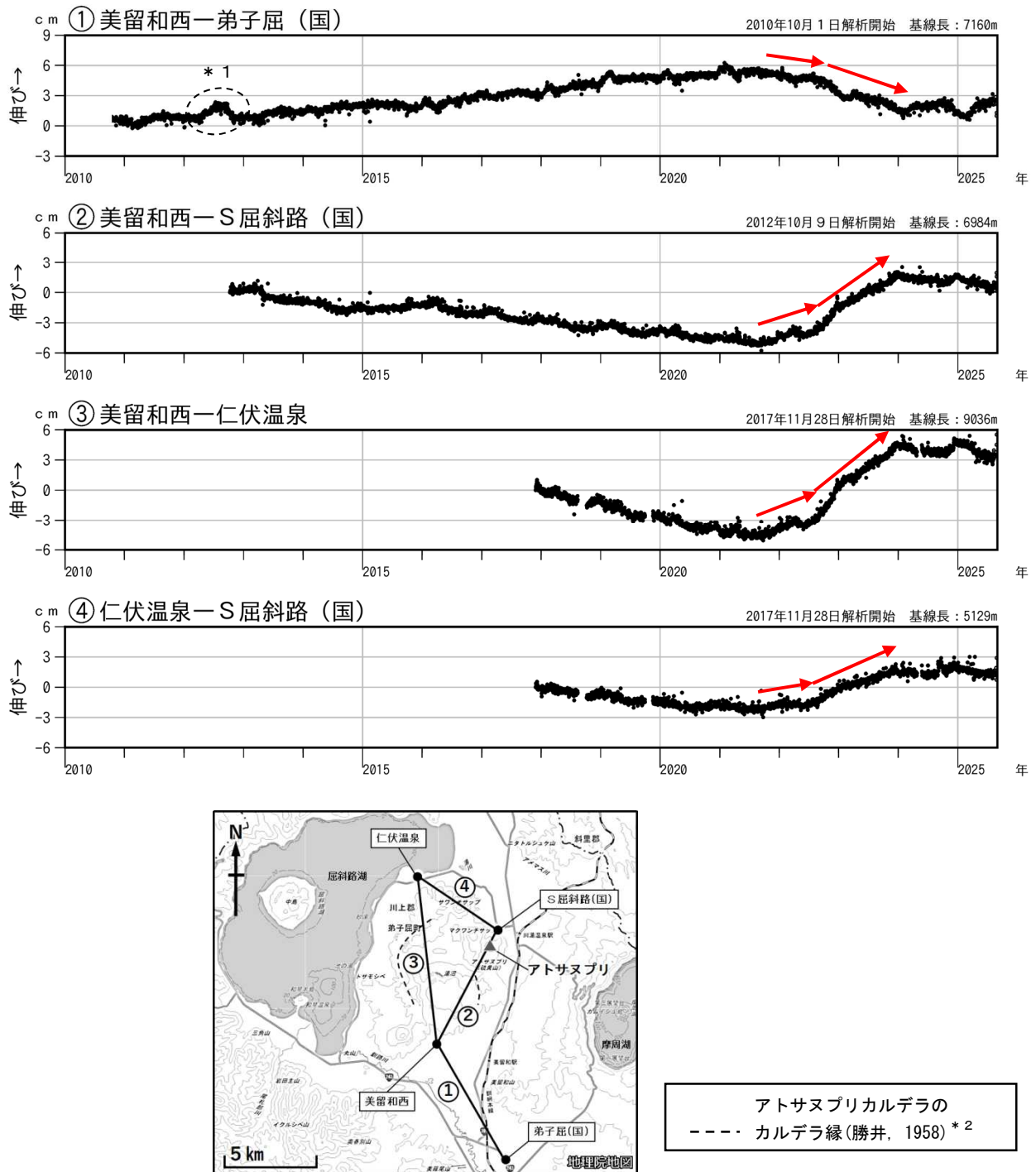
図 4 アトサヌプリ GNSS連続観測による基線長変化（2010年10月～2025年8月）及び観測点配置図
