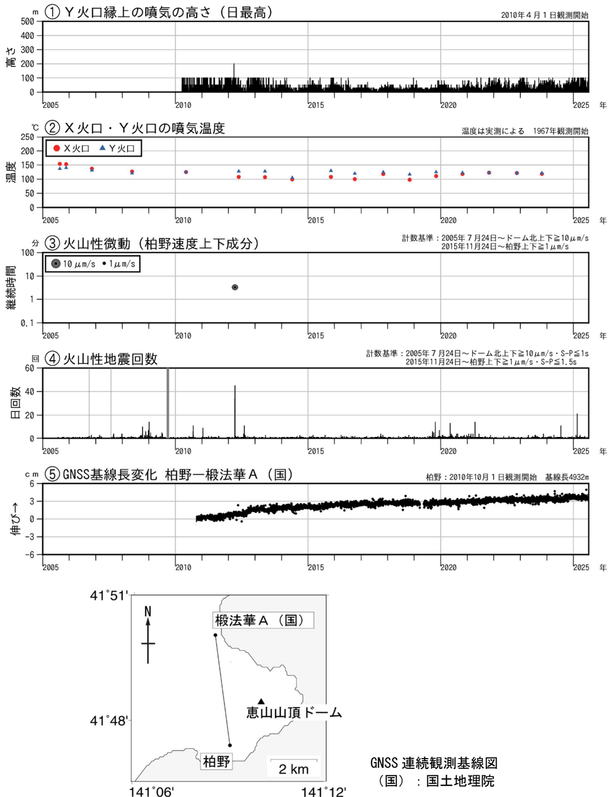
図 2 恵山 火山活動経過図（2005 年 7 月～2025 年 7 月） ④の灰色部分は機器障害による欠測期間を示します。 ⑤のグラフは上図の基線に対応しています。 ⑤のグラフの空白部分は欠測を示します。
