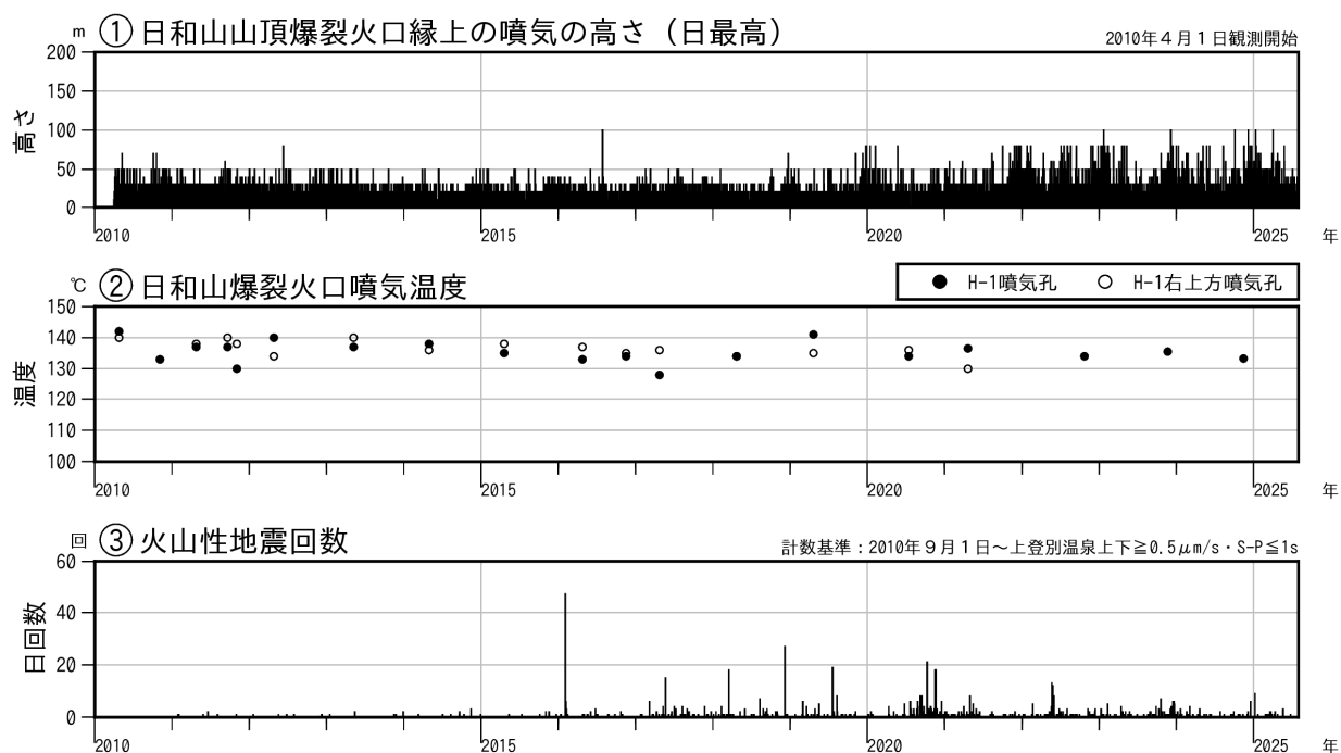
図2 倶多楽 火山活動経過図（2010年1月～2025年7月）
