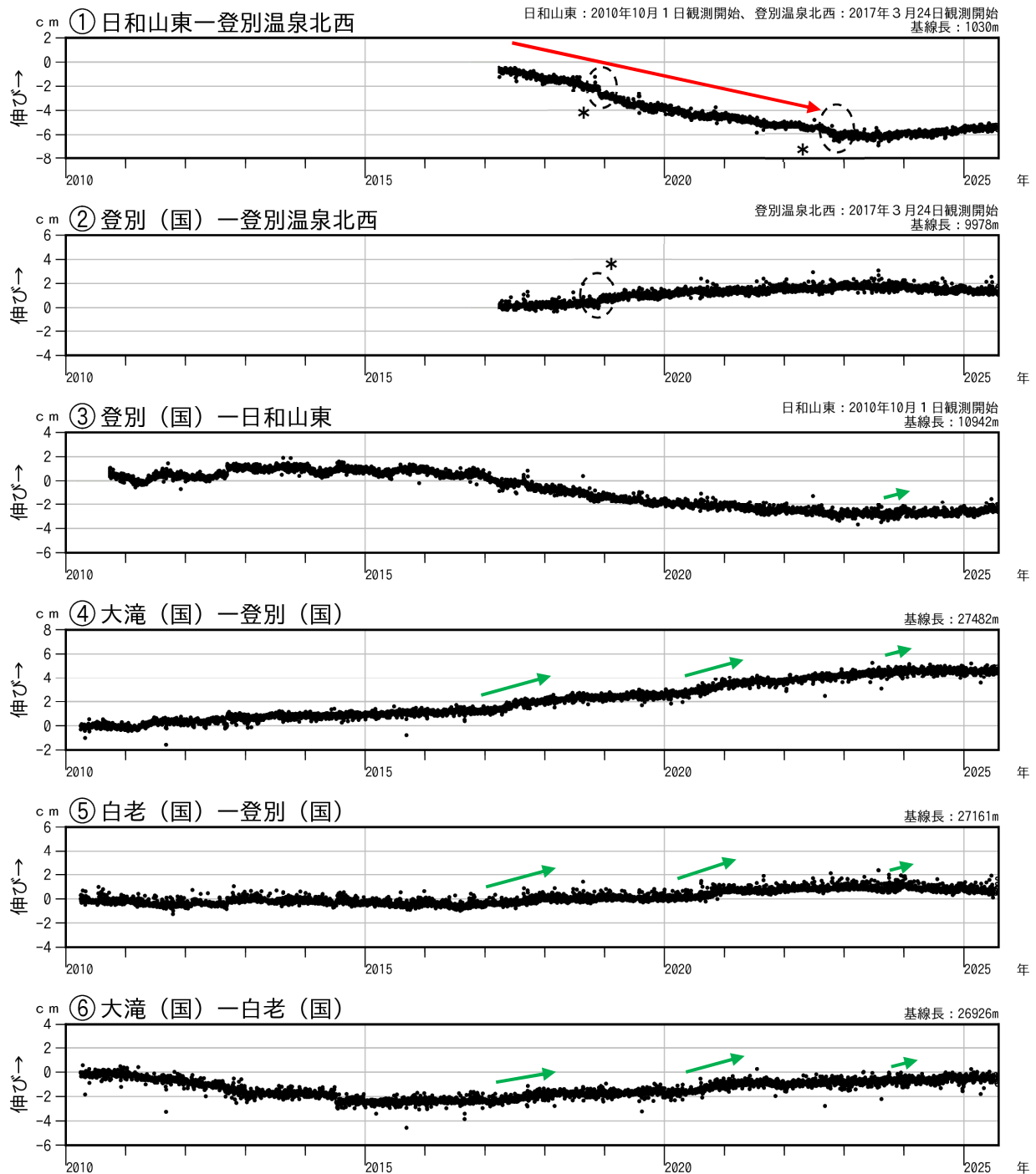
図3 倶多楽 GNSS連続観測による基線長変化（2010年4月～2025年7月）
