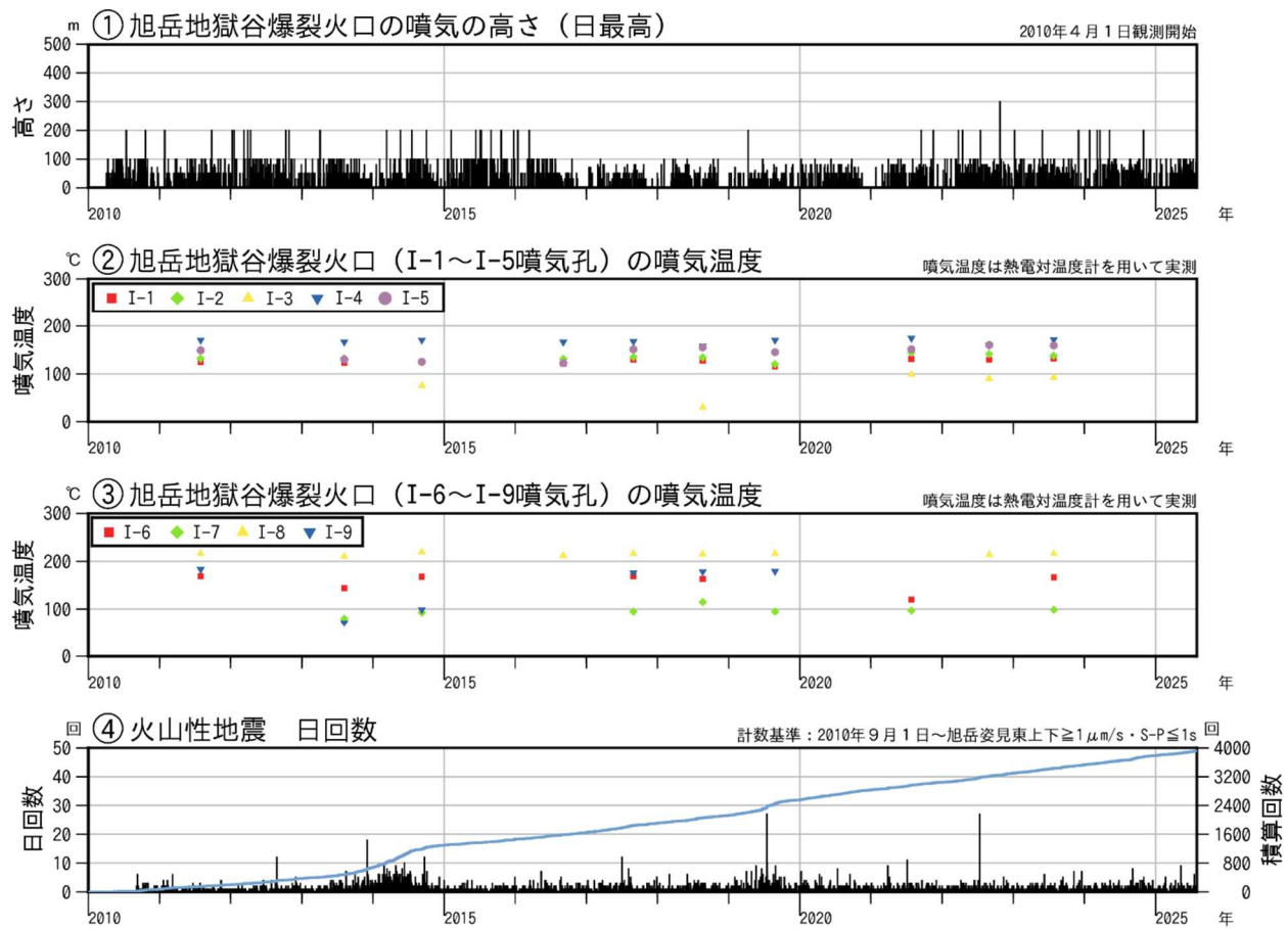
図2 大雪山 火山活動経過図（2010年4月～2025年7月）
