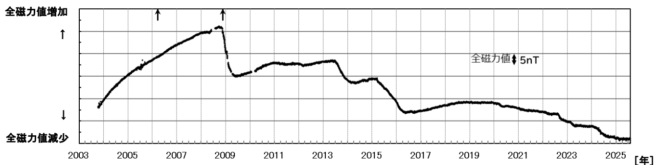
図8 雌阿寒岳 ポンマチネシリ96-1火口の噴気（噴煙）の長さとお磁力値の経過及び全磁力観測点配置図（2003年～2025年7月）
