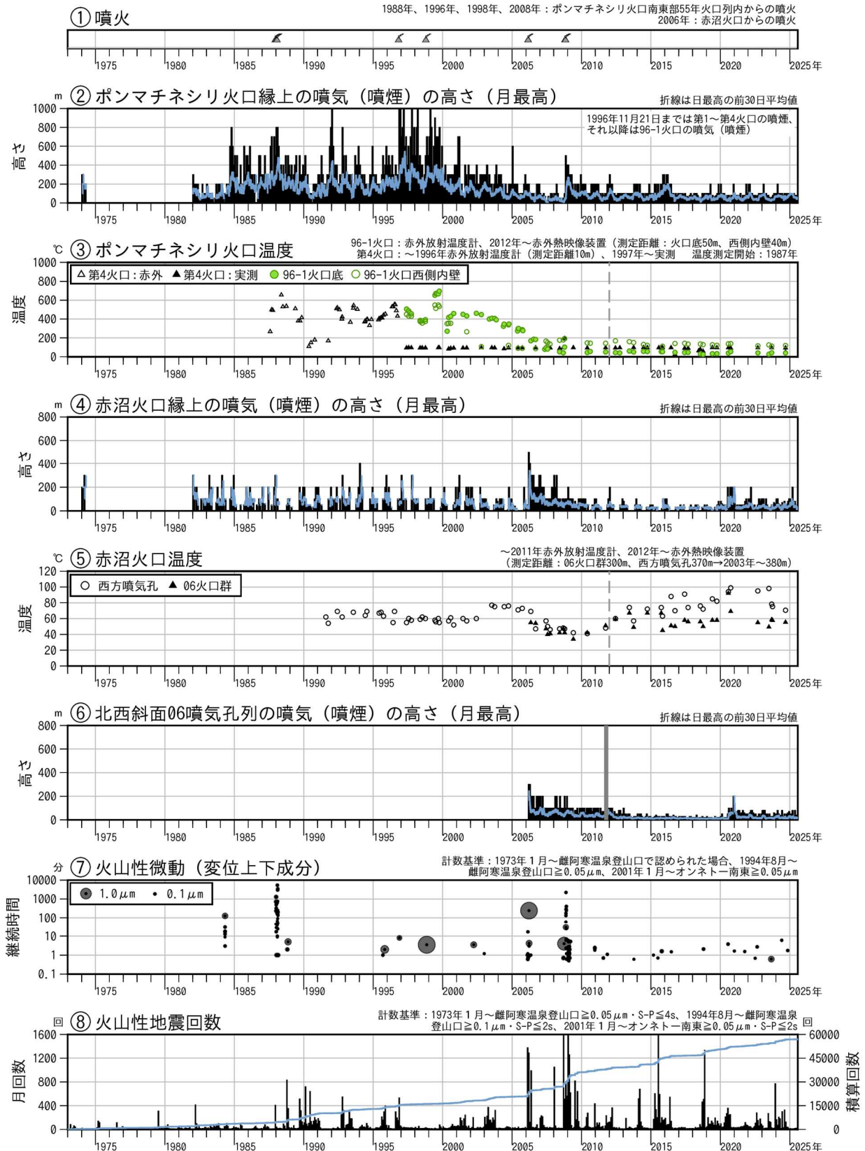
図6 雌阿寒岳 火山活動経過図（1973年1月～2025年7月）
