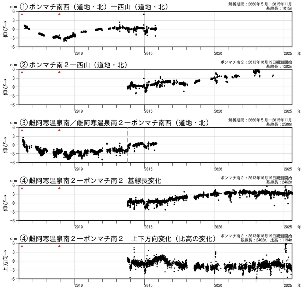
図10-1 雌阿寒岳 GNSS連続観測による基線長及び比高の変化（2006年4月～2025年7月）
