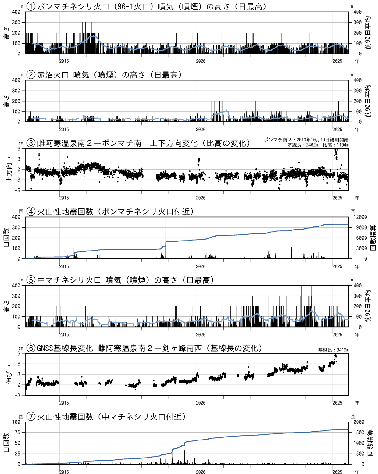
図7 雌阿寒岳 火口別の活動経過図（2013年10月～2025年7月）
