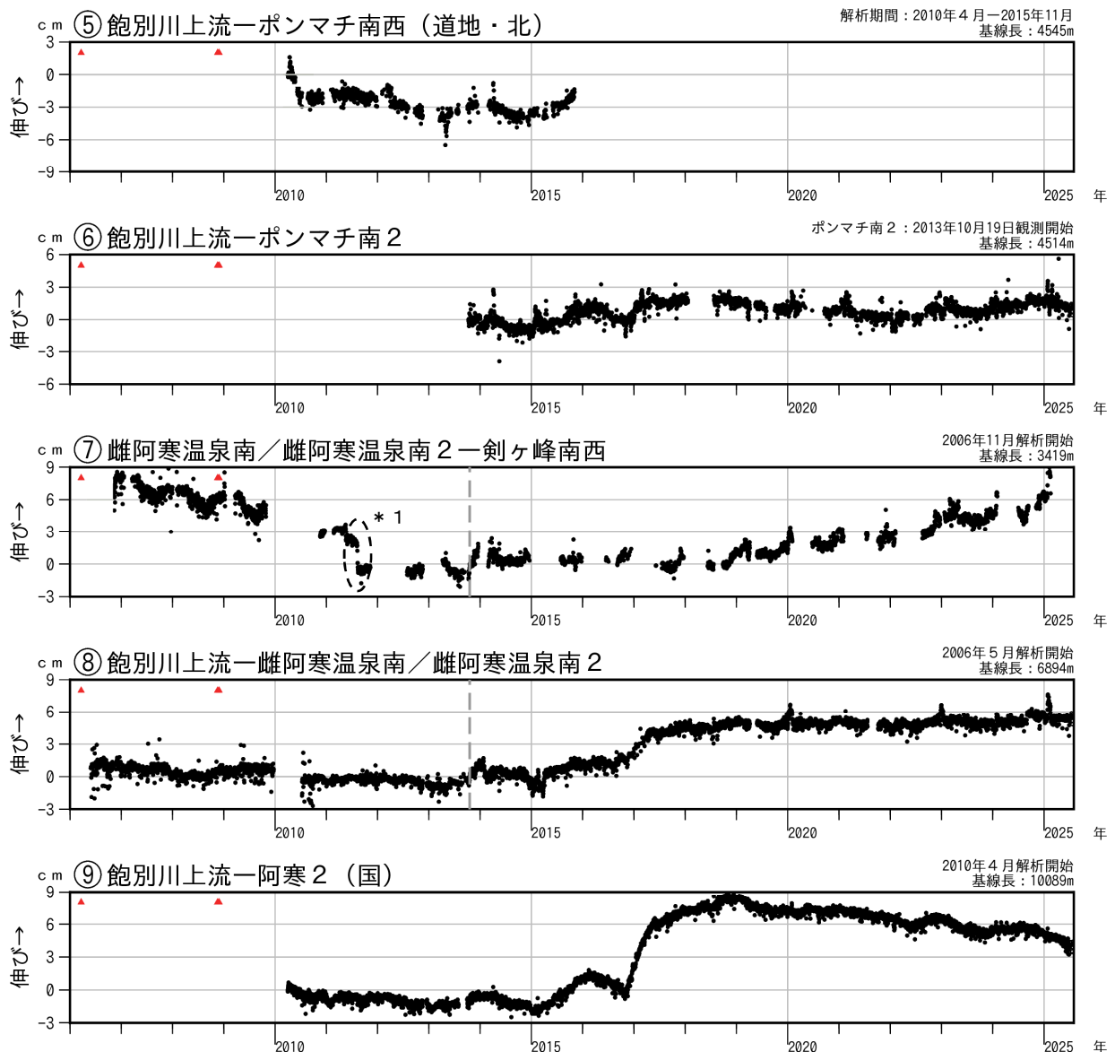
図10-2 雌阿寒岳 GNSS連続観測による基線長の変化（2006年4月～2025年7月）
