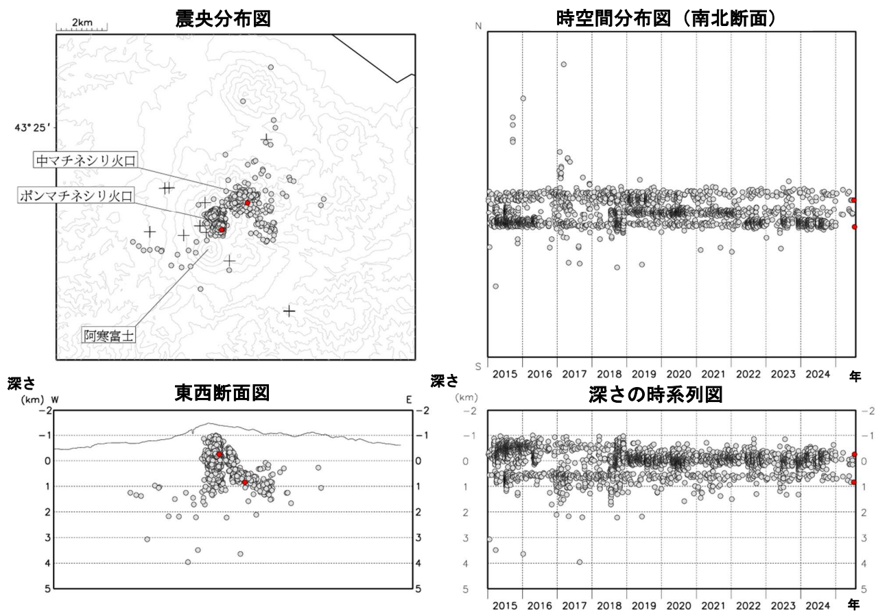
図9 雌阿寒岳 火山性地震の震源分布（2015年1月～2025年7月）
