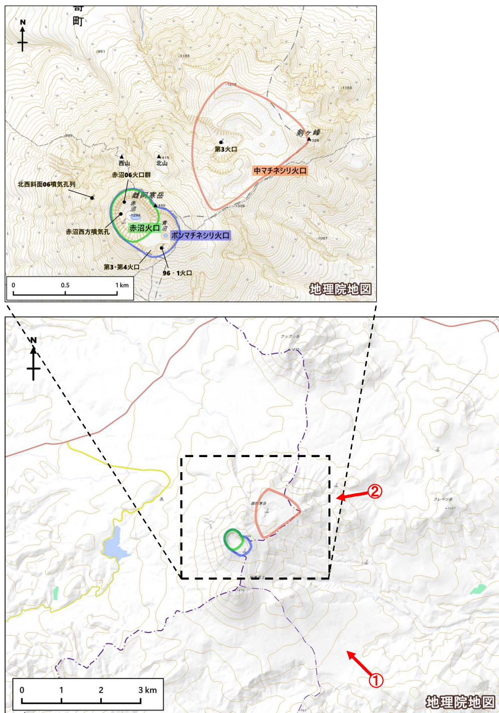
図1 雌阿寒岳 火口及び噴気孔の位置図と写真の撮影方向（矢印） 各火口の火口縁は、概ねの範囲を示すものです
