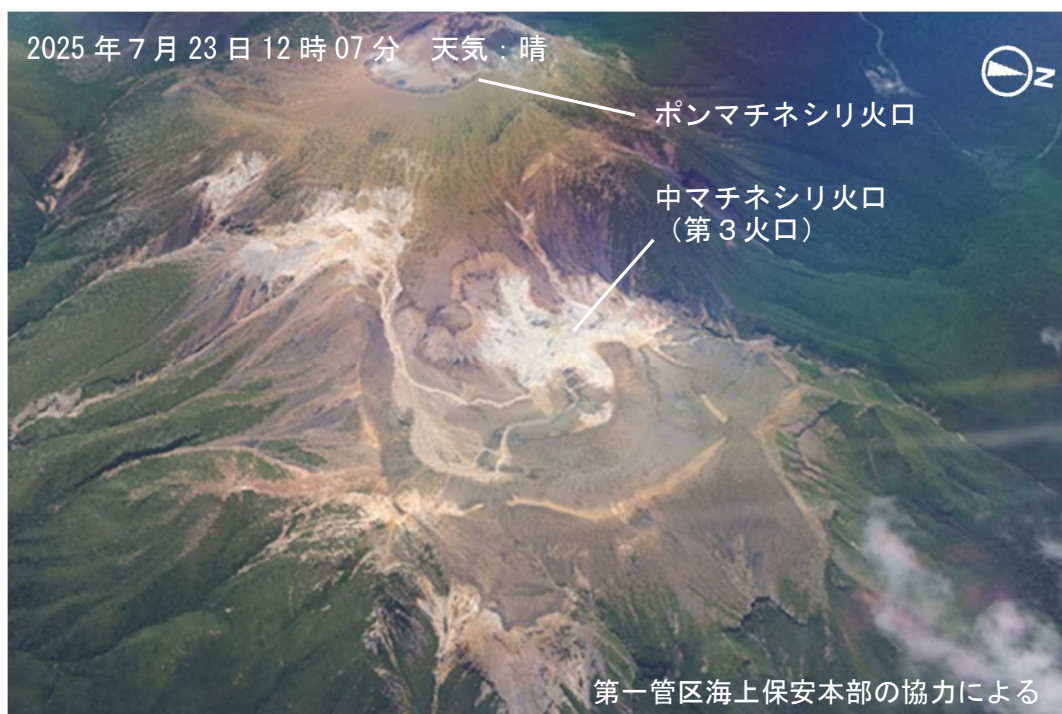
図5 雌阿寒岳 中マチネシリ火口付近の状況 東側上空（図1の②）から撮影 ・中マチネシリ火口内の噴気活動は引き続き低調で、特段の変化は認められませんでした。
