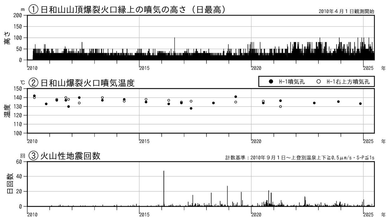
図2 倶多楽 火山活動経過図（2010年1月～2025年6月）
