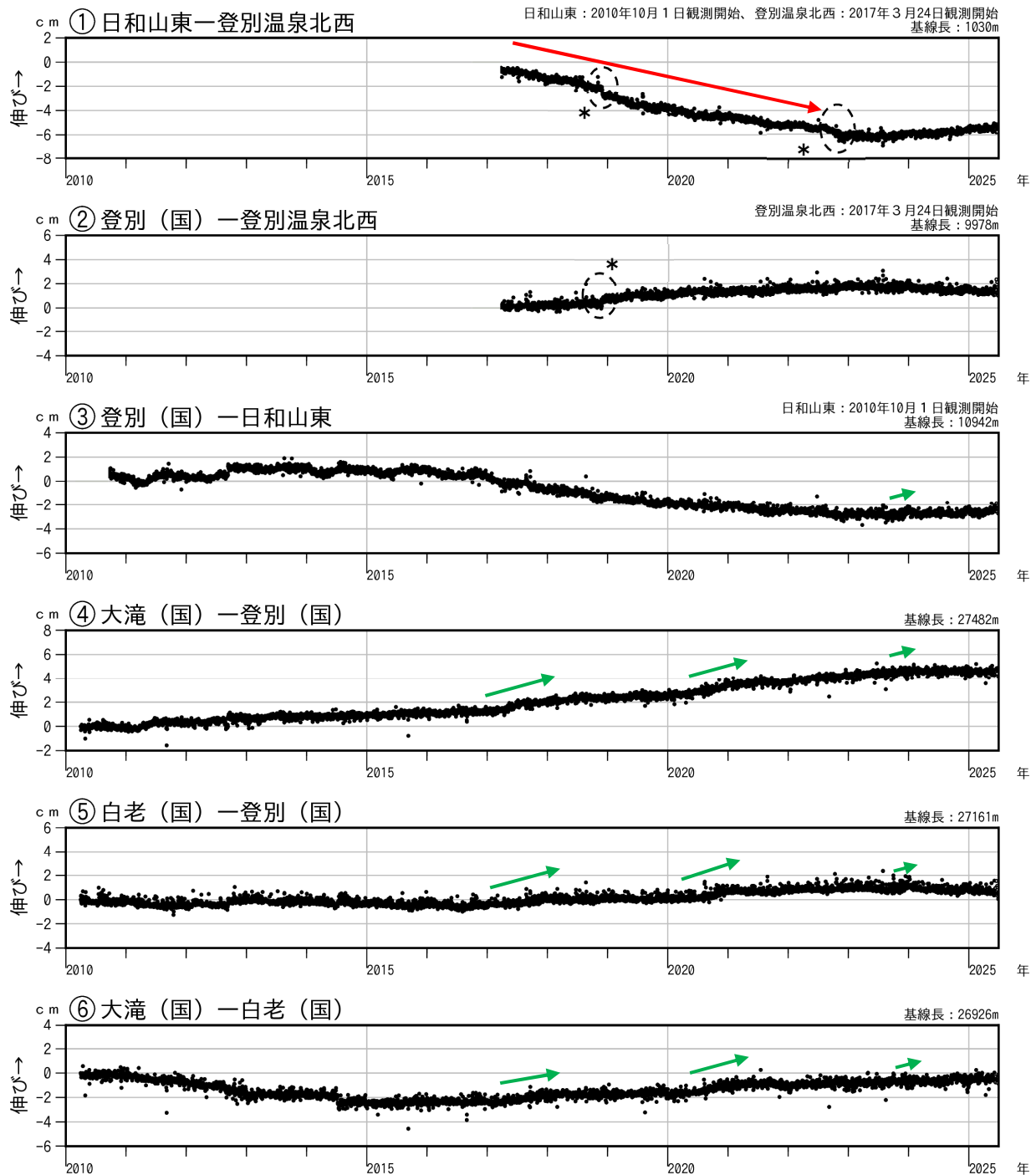
図3 倶多楽 GNSS連続観測による基線長変化（2010年4月～2025年6月）
