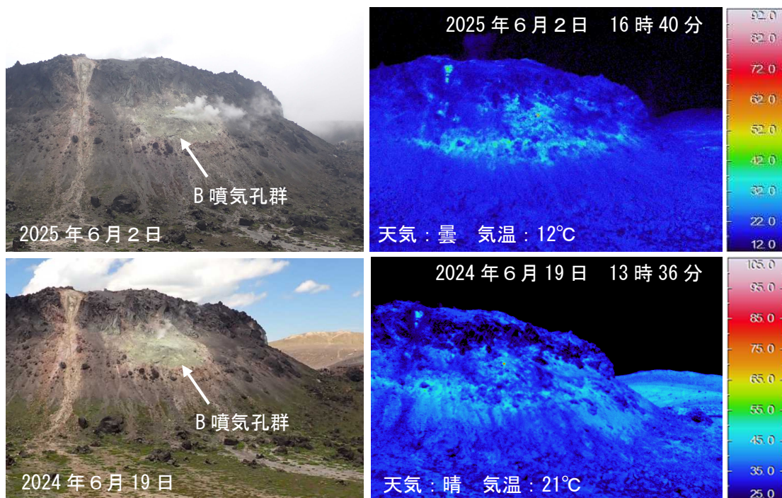
図6 樽前山 赤外熱映像装置によるB噴気孔群の地表面温度分布の比較
