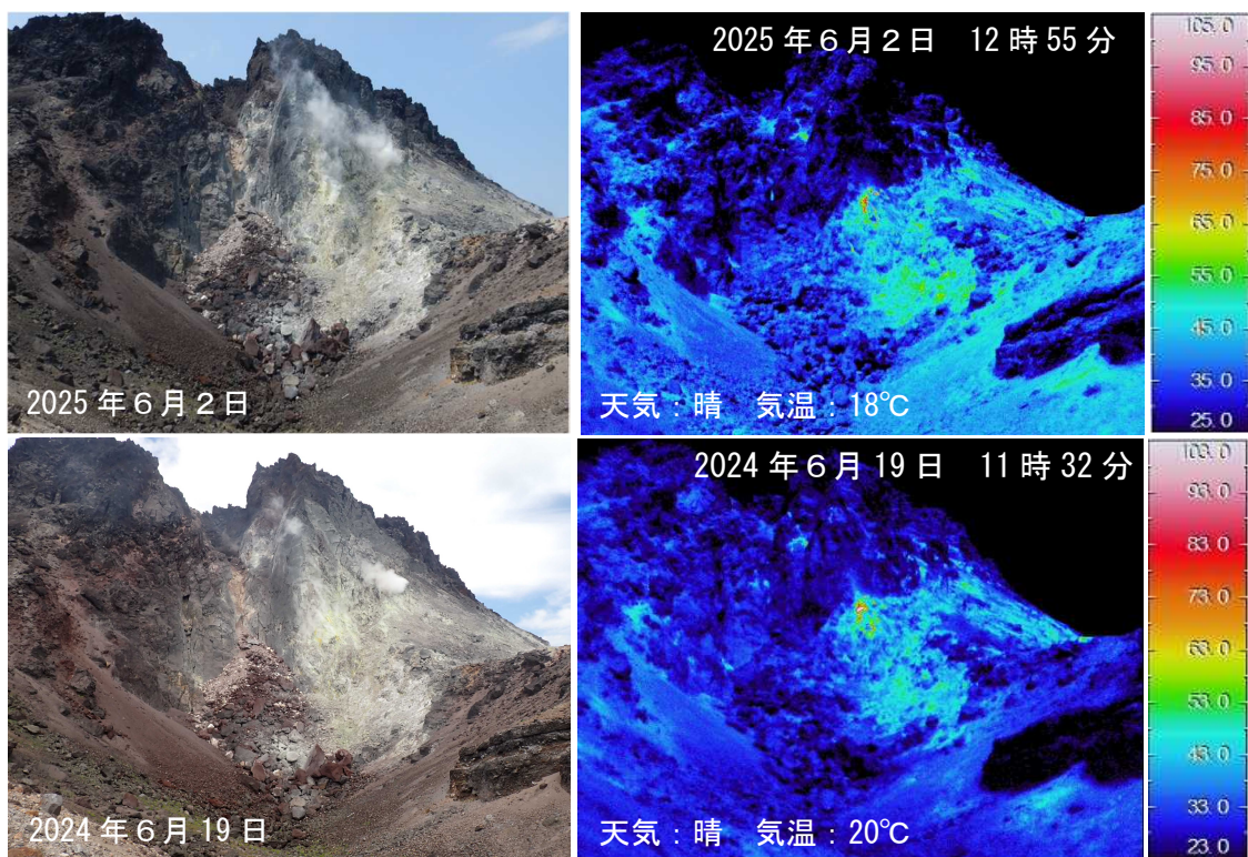
図5 樽前山 赤外熱映像装置によるH亀裂の地表面温度分布の比較
