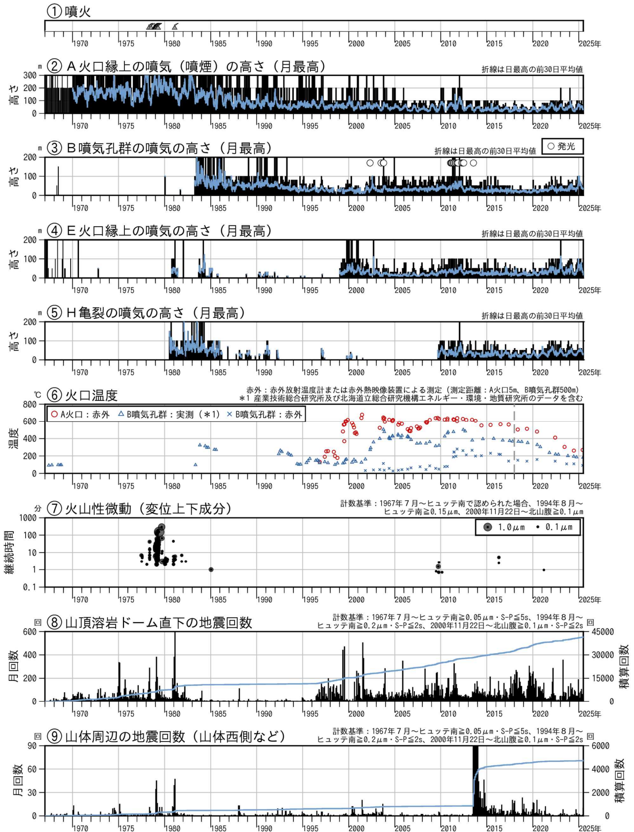
図1 樽前山 火山活動経過図（1967年1月～2025年6月）
