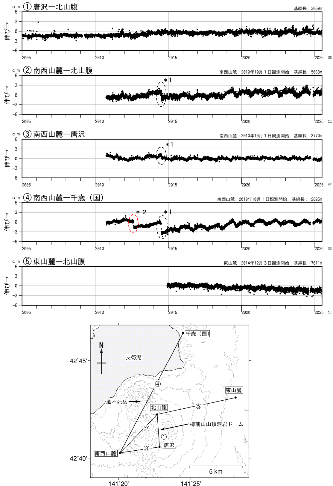
図8 樽前山 GNSS連続観測による基線長変化（2005年1月～2025年6月）及び観測点配置図
