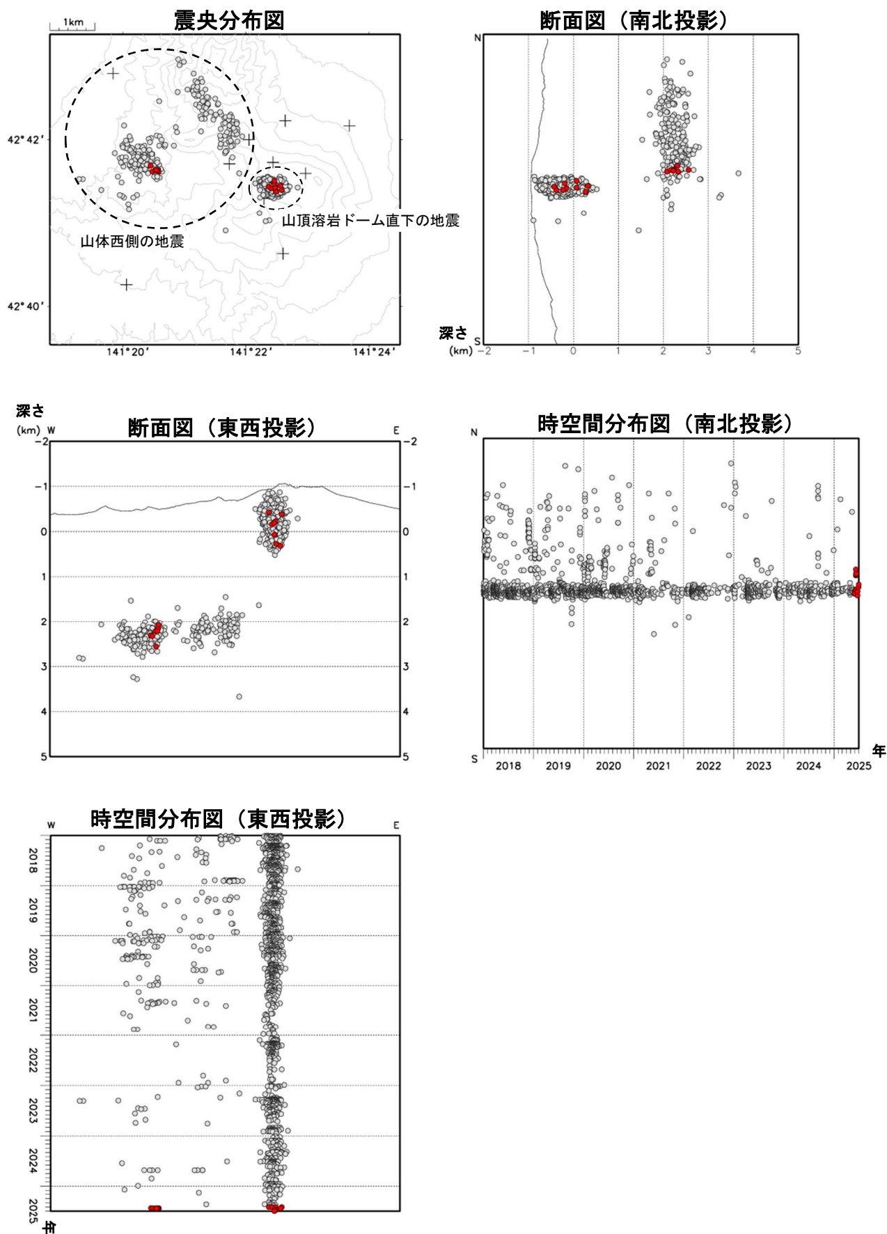
図7 樽前山 火山性地震の震源分布（2018年1月～2025年6月）
