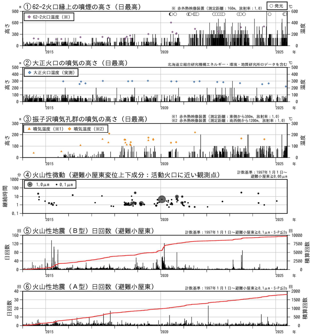
図2 十勝岳 火山活動経過図（2014年1月～2025年6月）
