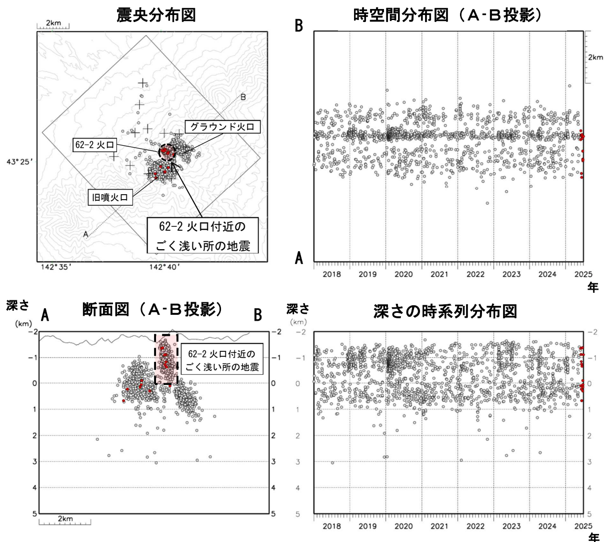
図4 十勝岳 火山性地震の震源分布（2018年1月～2025年6月）
