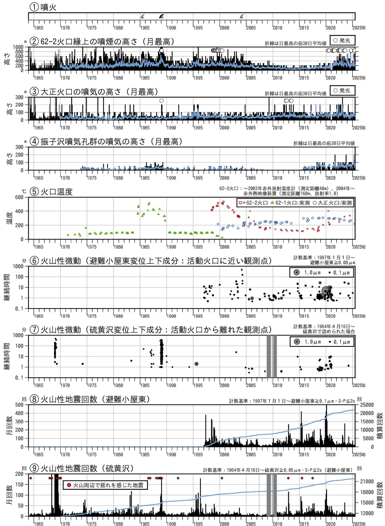
図1 十勝岳 火山活動経過図（1964年1月～2025年6月）
