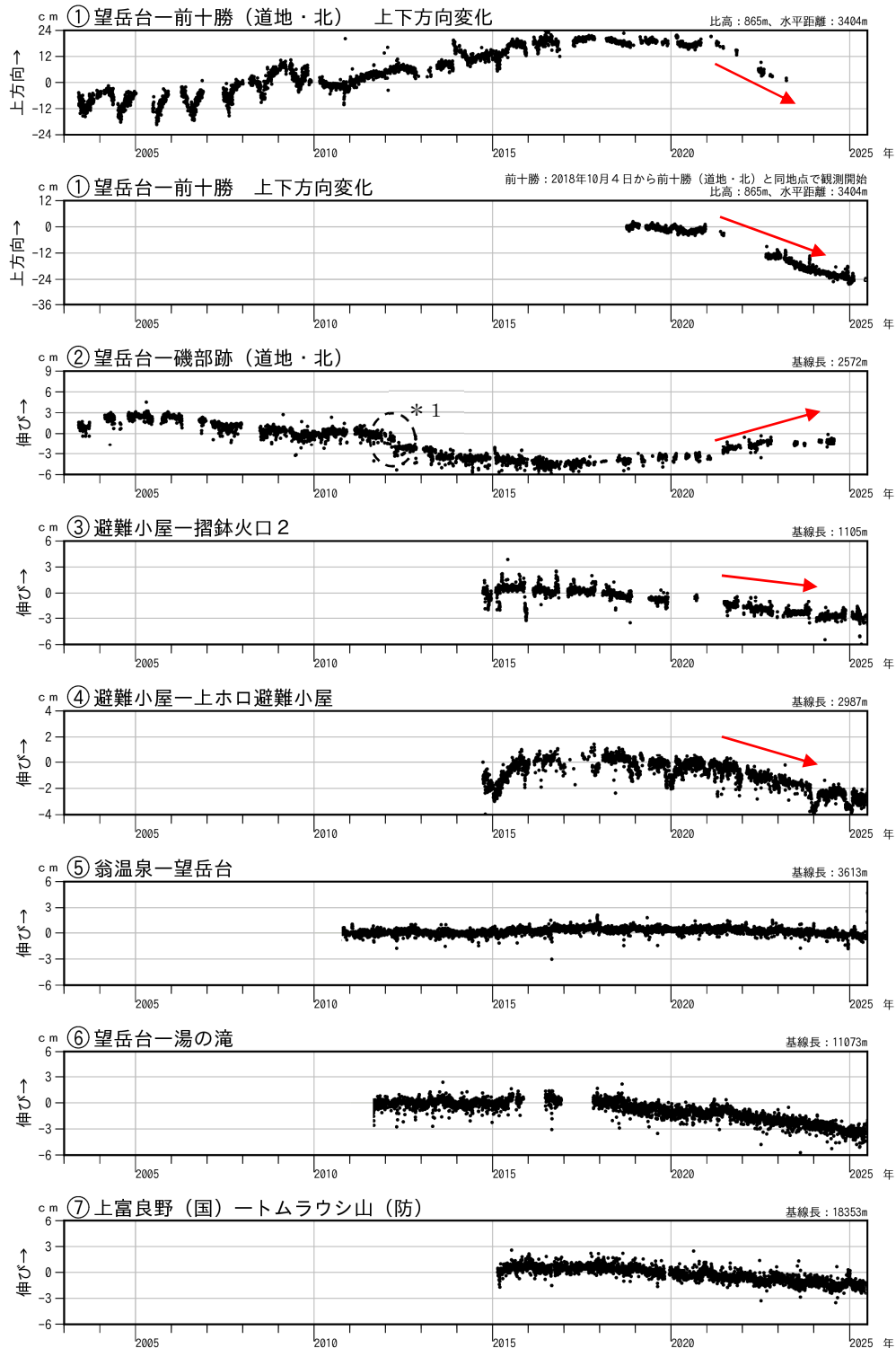
図5 十勝岳 GNSS連続観測による上下方向変化及び基線長変化（2003年5月～2025年6月）
