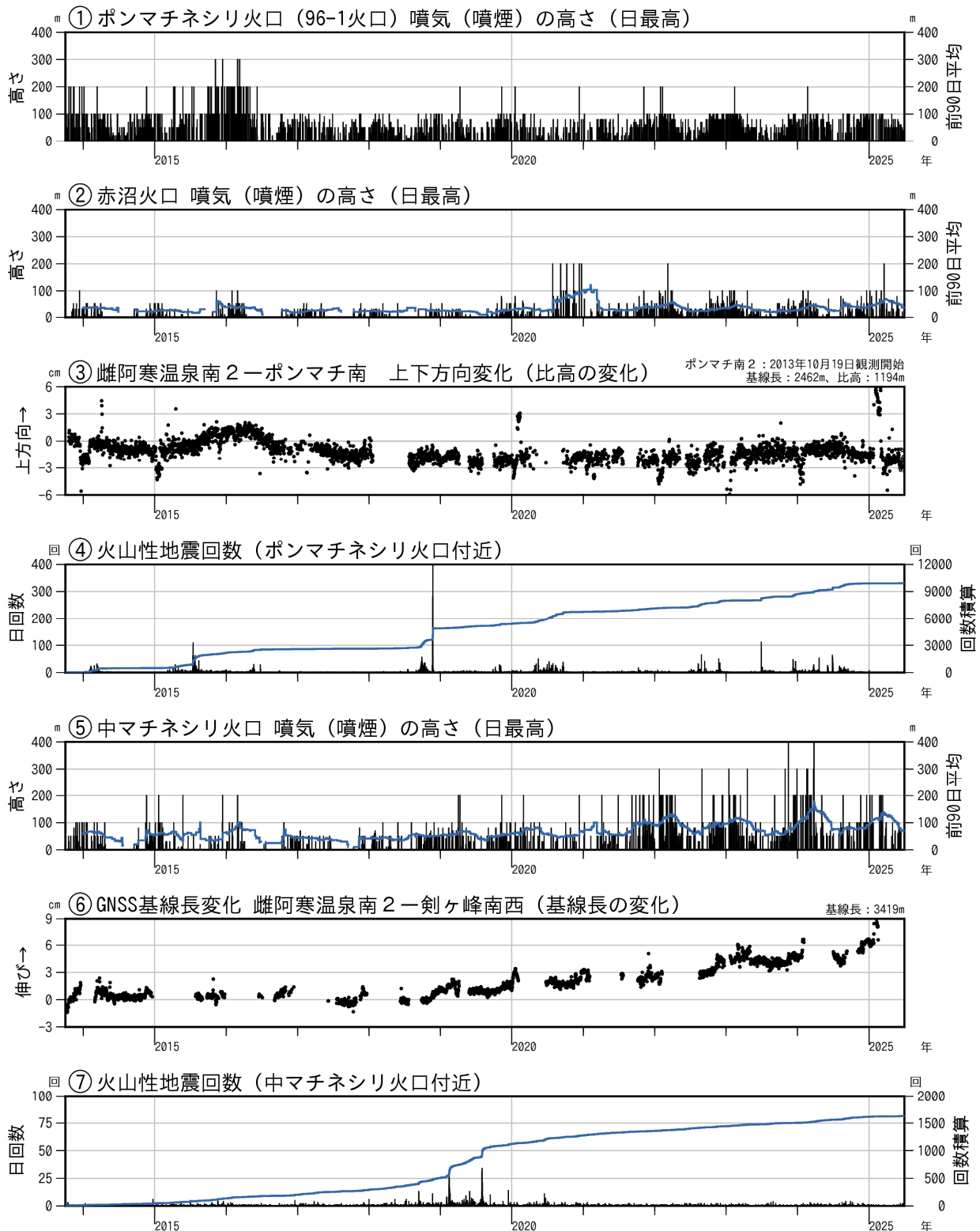
図5 雌阿寒岳 火口別の活動経過図（2013年10月～2025年6月）
