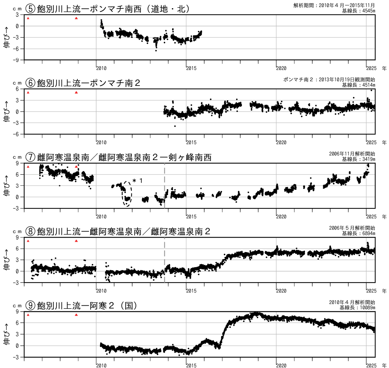
図8-2 雌阿寒岳 GNSS連続観測による基線長の変化（2006年4月～2025年6月）
