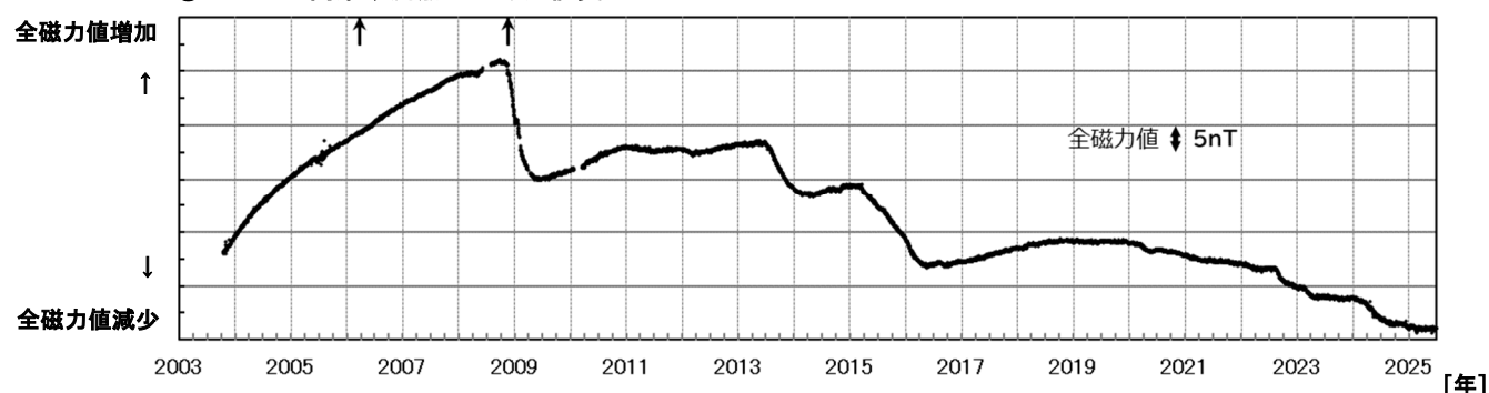
図6 雌阿寒岳 ポンマチネシリ96-1火口の噴気（噴煙）の長さと全磁力値の経過及び全磁力観測点配置図（2003年～2025年6月）
