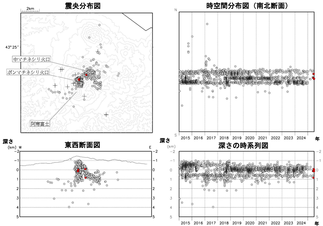
図7 雌阿寒岳 火山性地震の震源分布（2015年1月～2025年6月） ●：2015年1月～2025年5月の震源 ●：2025年6月の震源 ＋：地震観測点
