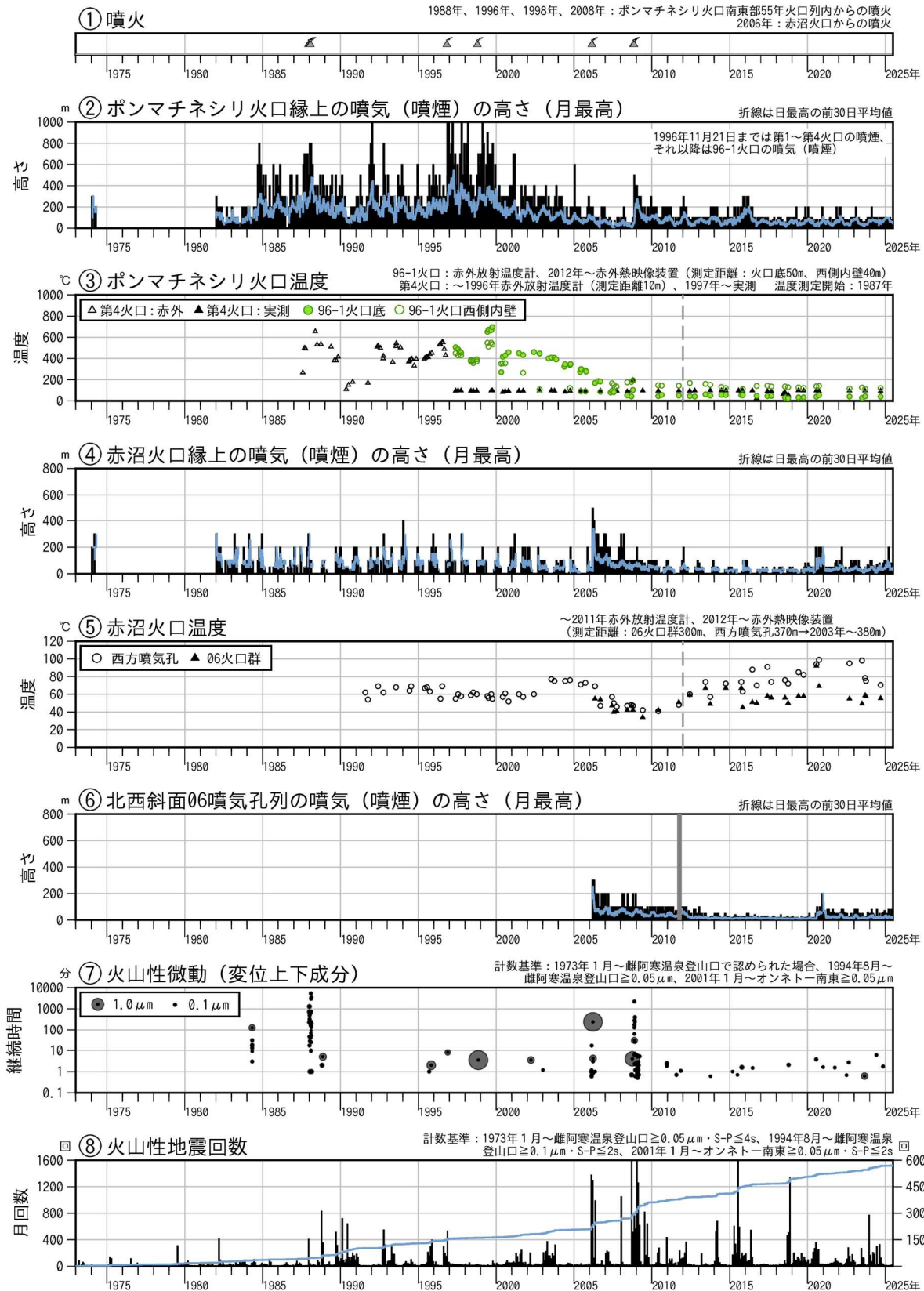
図4 雌阿寒岳 火山活動経過図（1973年1月～2025年6月）
