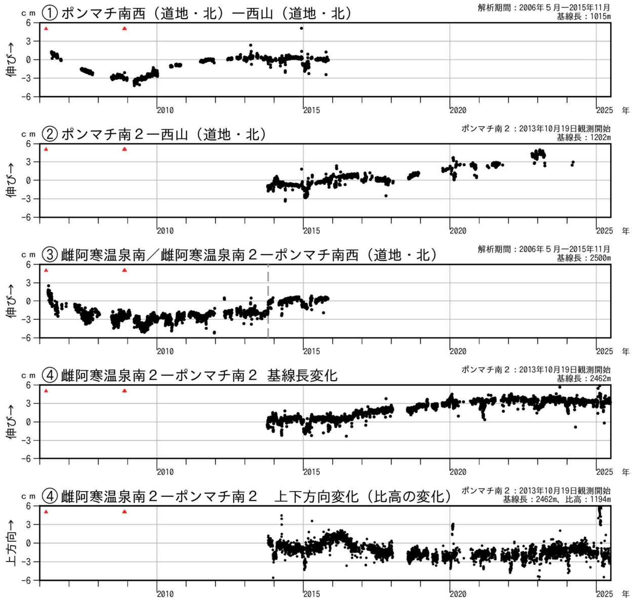
図8-1 雌阿寒岳 GNSS連続観測による基線長及び比高の変化（2006年4月～2025年6月）
