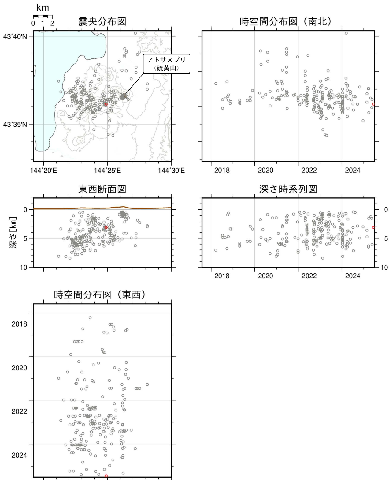
図3 アトサヌプリ 火山性地震の震源分布（2017年8月～2025年6月） ○：2017年8月～2025年5月の震源 ○：2025年6月の震源
