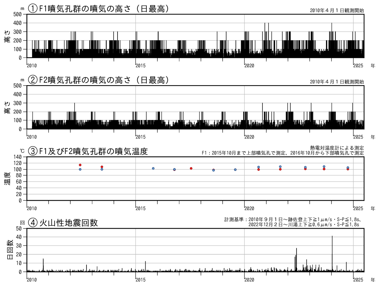
図1 アトサヌプリ 火山活動経過図（2010年4月～2025年6月）
