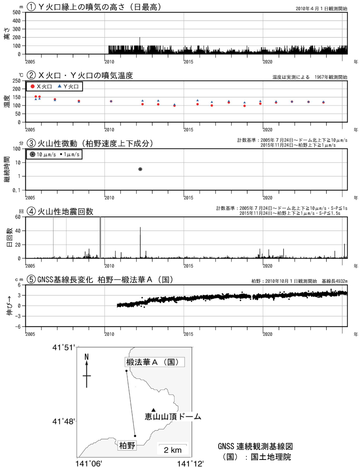
図2 恵山 火山活動経過図（2005年7月～2025年4月） ④の灰色部分は機器障害による欠測期間を示します。 ⑤のグラフは上図の基線に対応しています。 ⑤のグラフの空白部分は欠測を示します。
