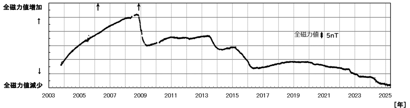
図5 雌阿寒岳 ポンマチネシリ96-1火口の噴気（噴煙）の長さや全磁力値の経過及び全磁力観測点配置図（2003年～2025年4月）
