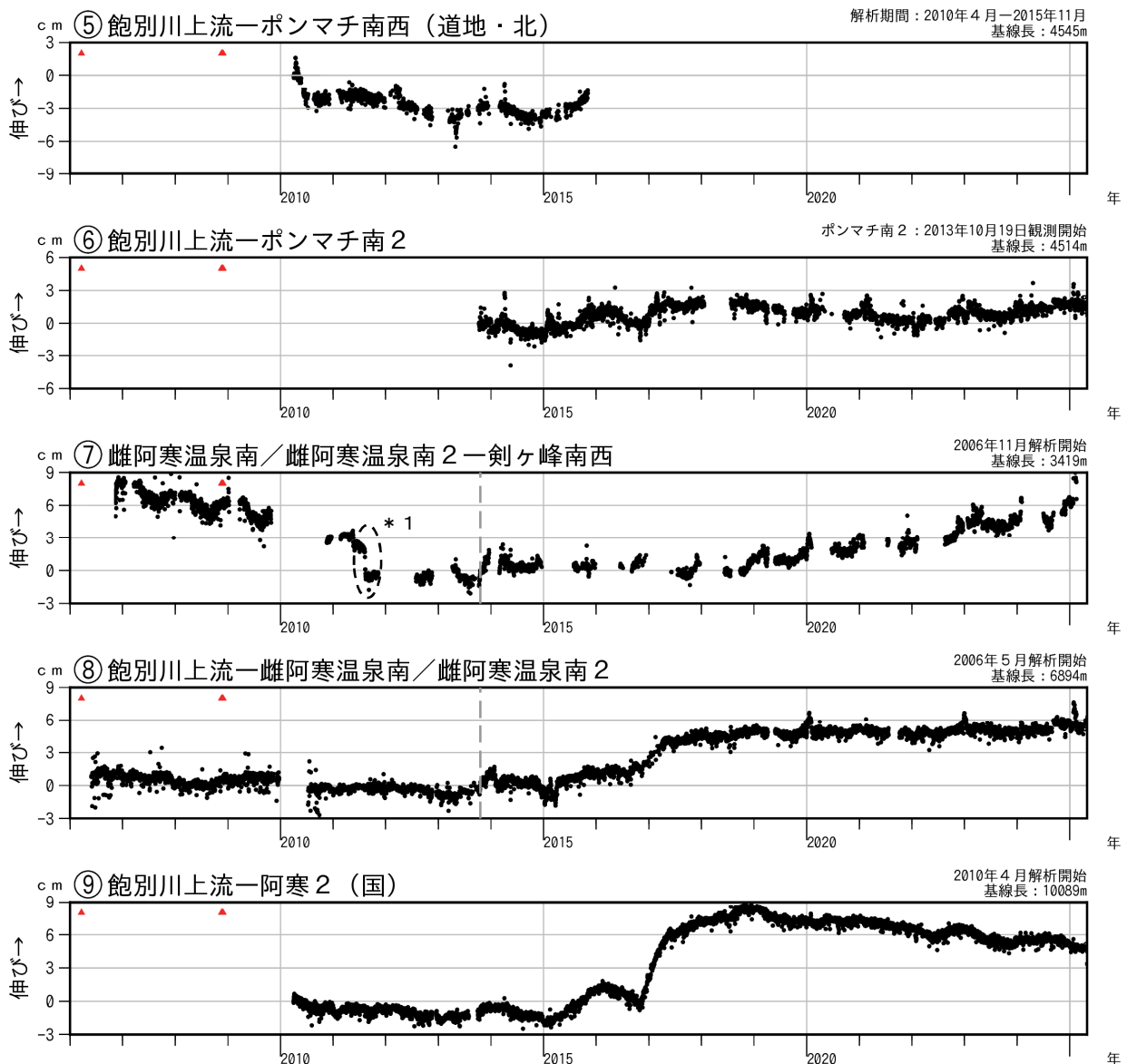
図7-2 雌阿寒岳 GNSS連続観測による基線長の変化（2006年4月～2025年4月）
