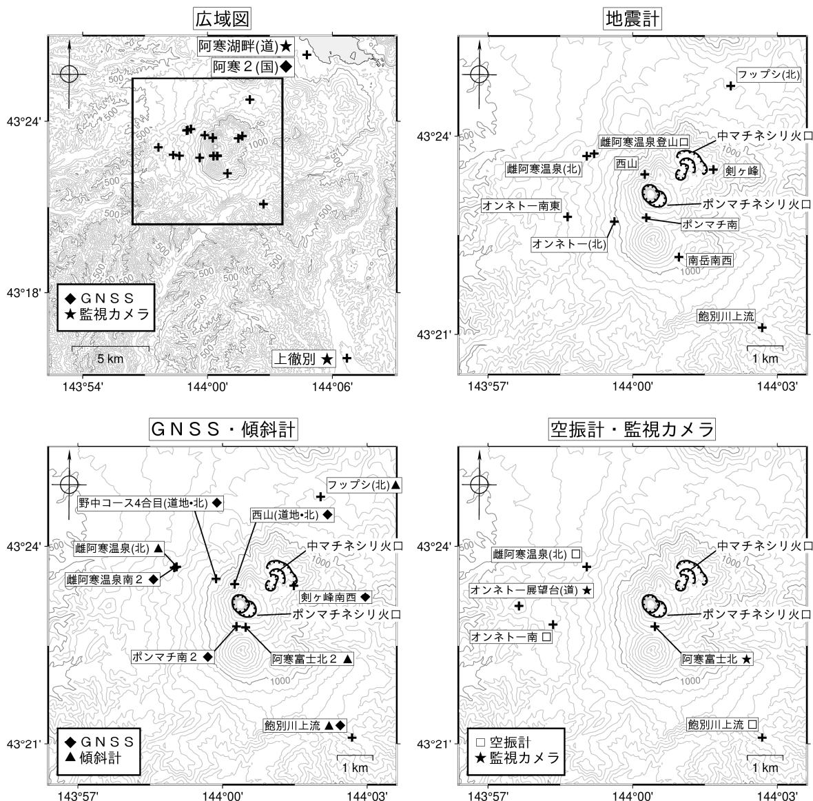
図9 雌阿寒岳 観測点配置図
