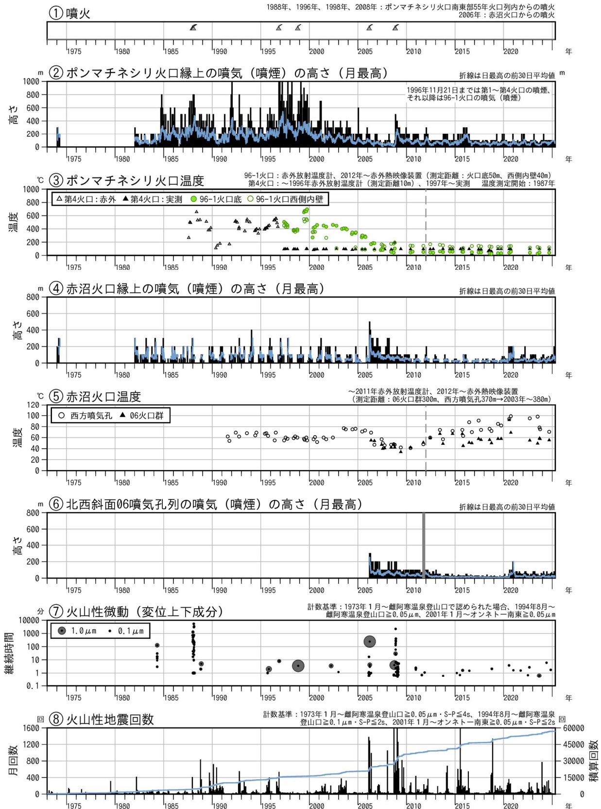
図4 雌阿寒岳 火山活動経過図（1973年1月～2025年4月）
