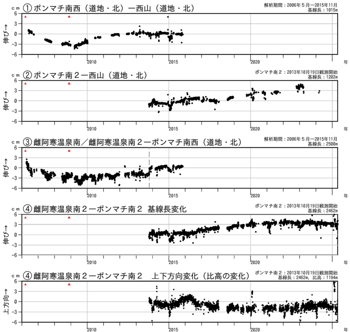
図7-1 雌阿寒岳 GNSS連続観測による基線長及び比高の変化（2006年4月～2025年4月）
