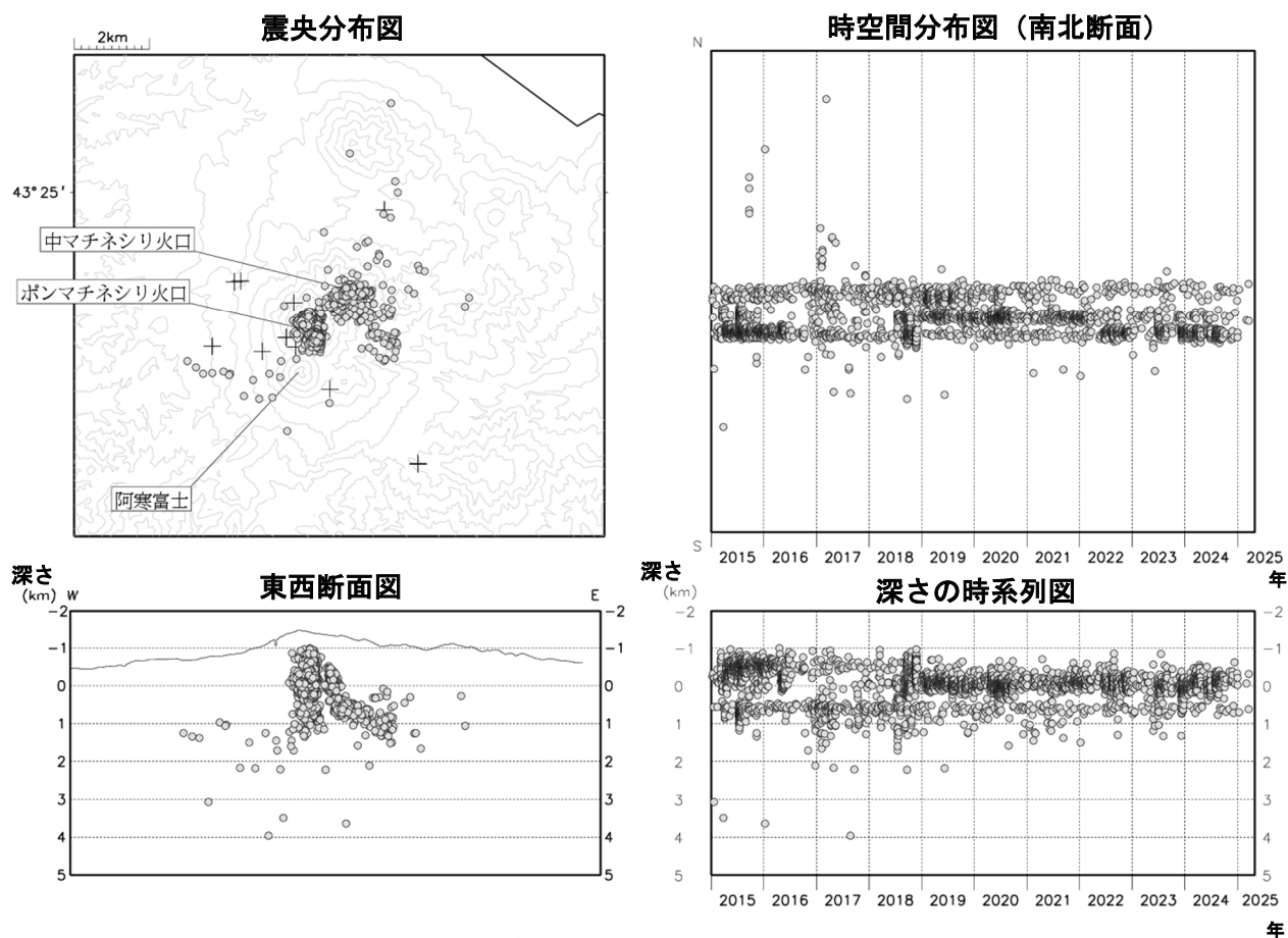
図6 雌阿寒岳 火山性地震の震源分布（2015年1月～2025年4月）
