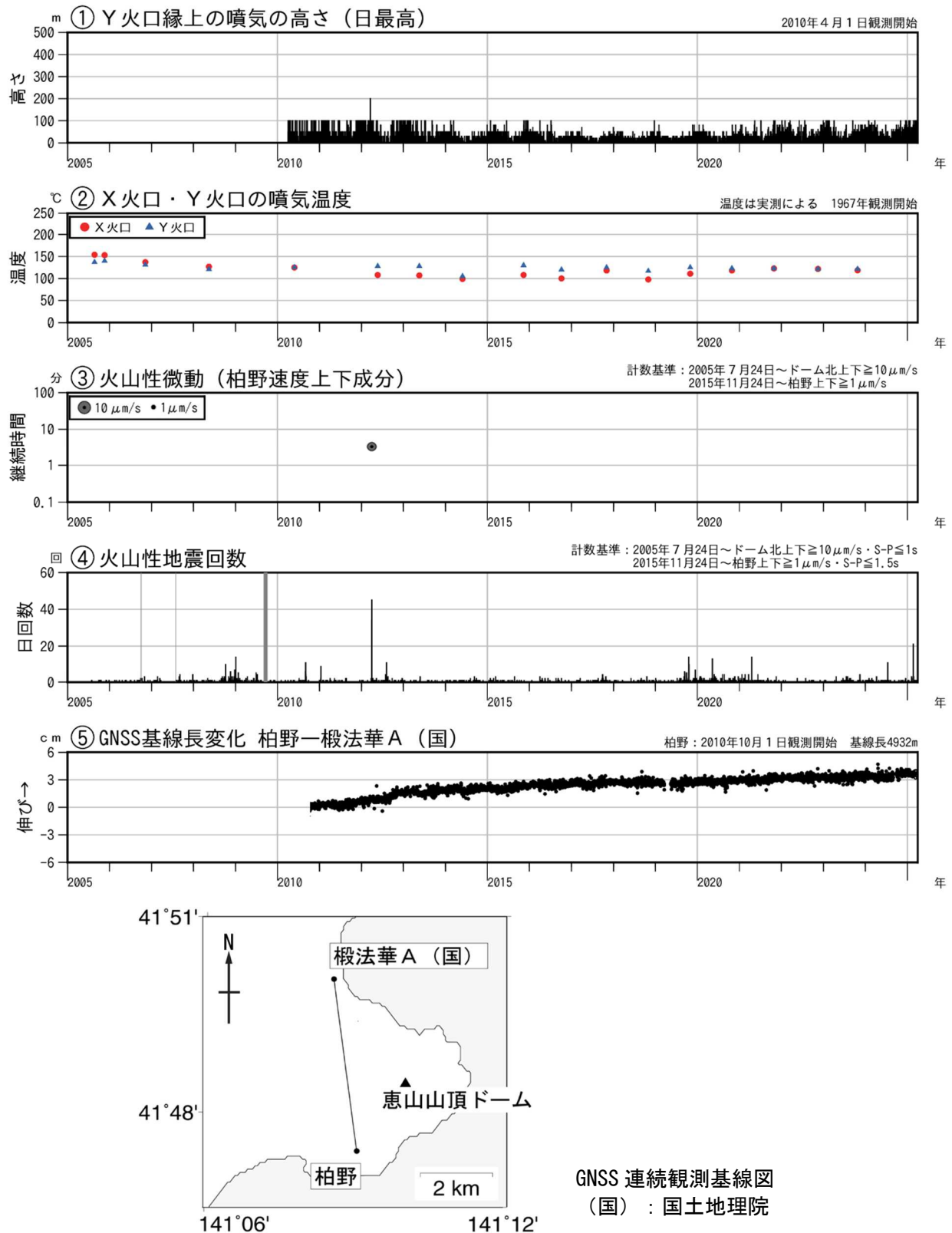
図 2 恵山 火山活動経過図（2005 年 7 月～2025 年 3 月） ④の灰色部分は機器障害による欠測期間を示します。 ⑤のグラフは上図の基線に対応しています。 ⑤のグラフの空白部分は欠測を示します。
