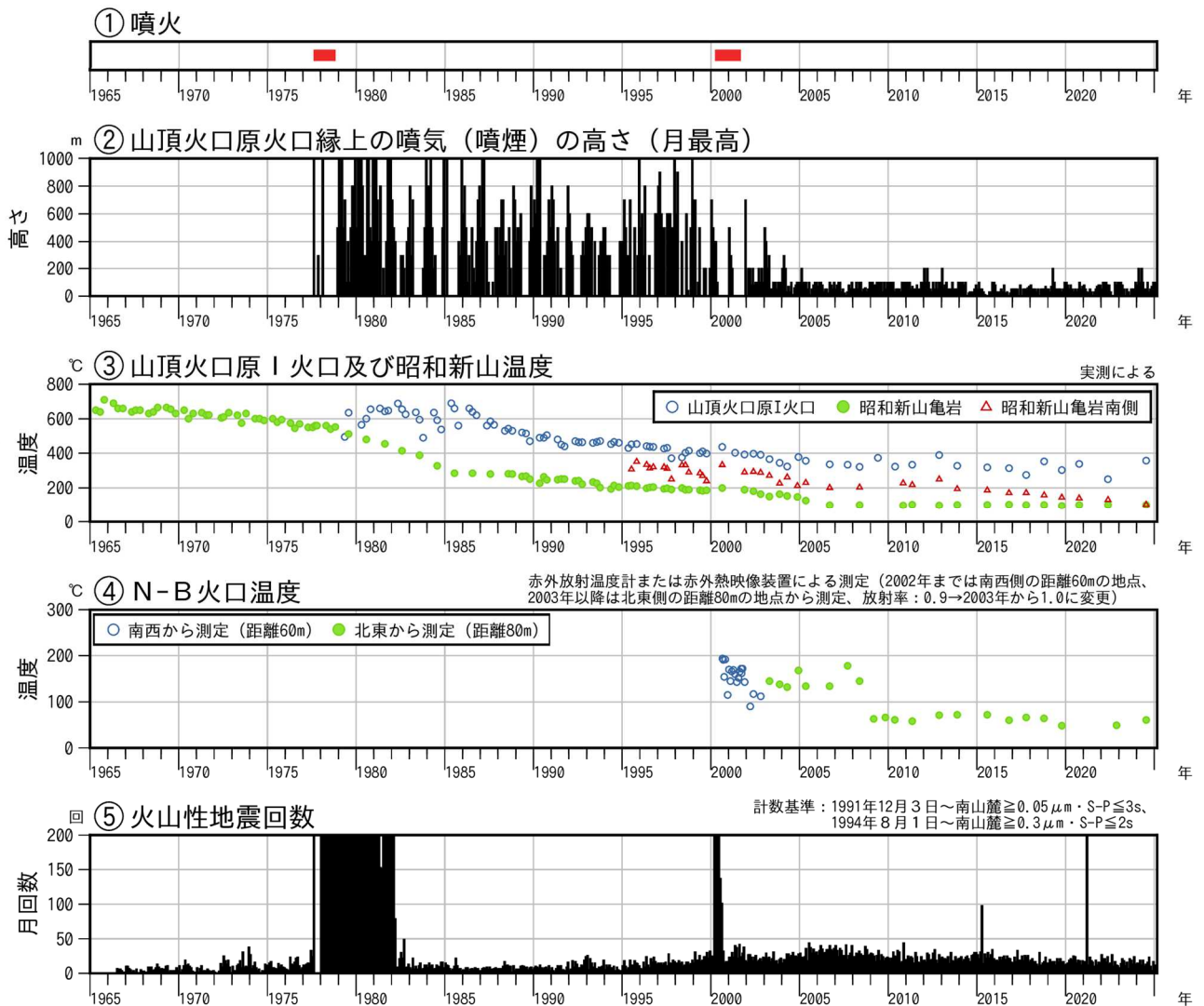
図1 有珠山 火山活動経過図（1965年1月～2025年2月）
