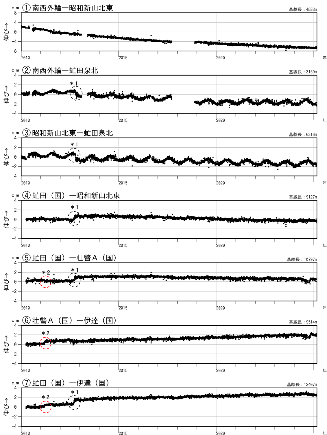
図4 有珠山 GNSS連続観測による基線長変化（2010年1月～2025年2月）
