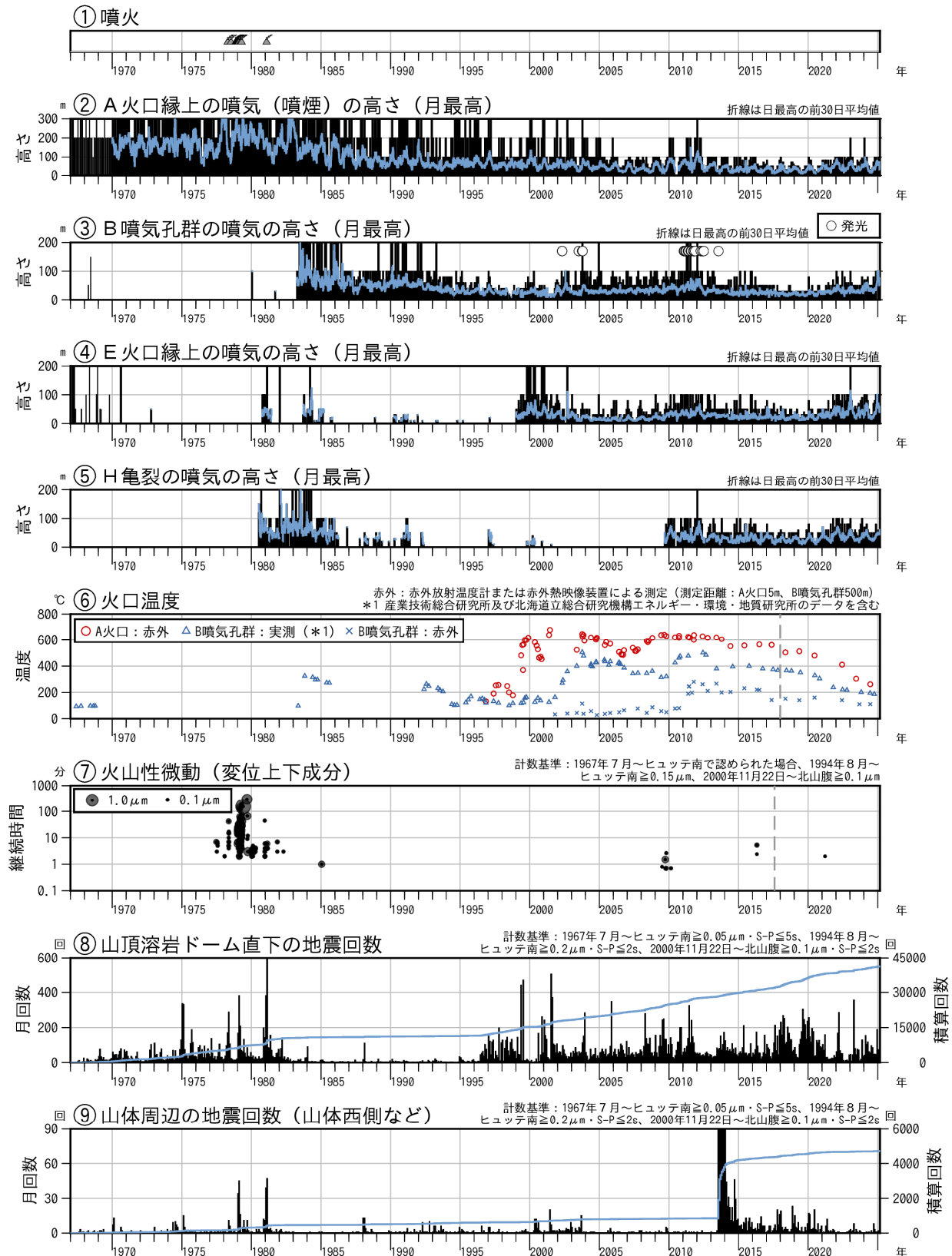
図2 樽前山 火山活動経過図（1967年1月～2025年2月）
