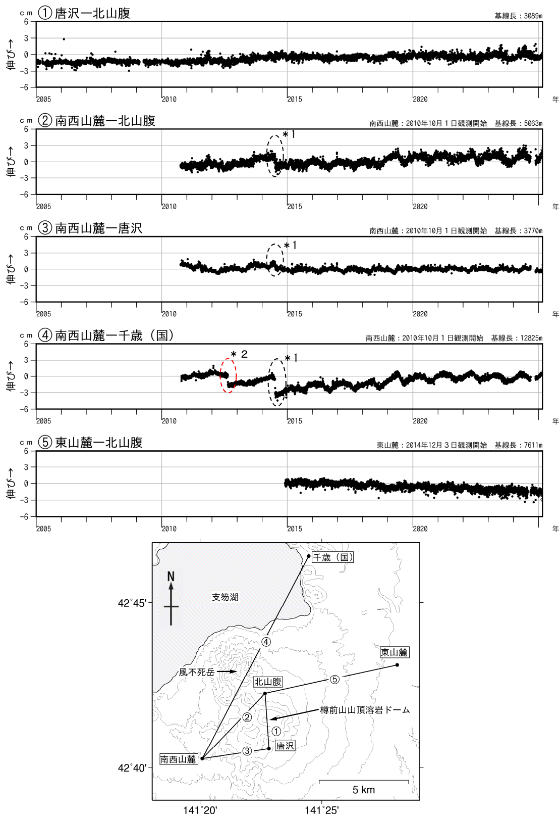
図4 樽前山 GNSS連続観測による基線長変化（2005年1月～2025年2月）及び観測点配置図
