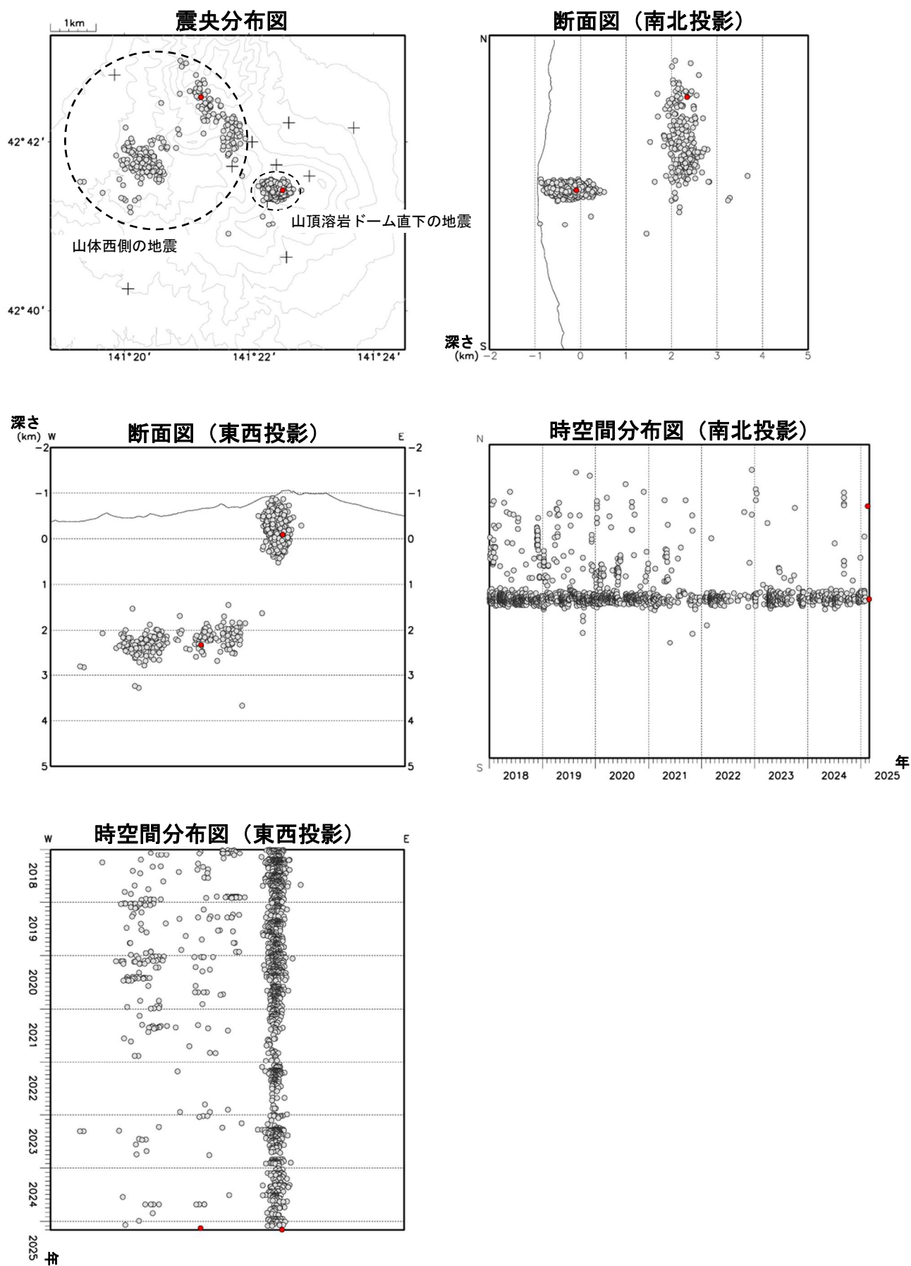
図3 樽前山 火山性地震の震源分布（2018年1月～2025年2月）
