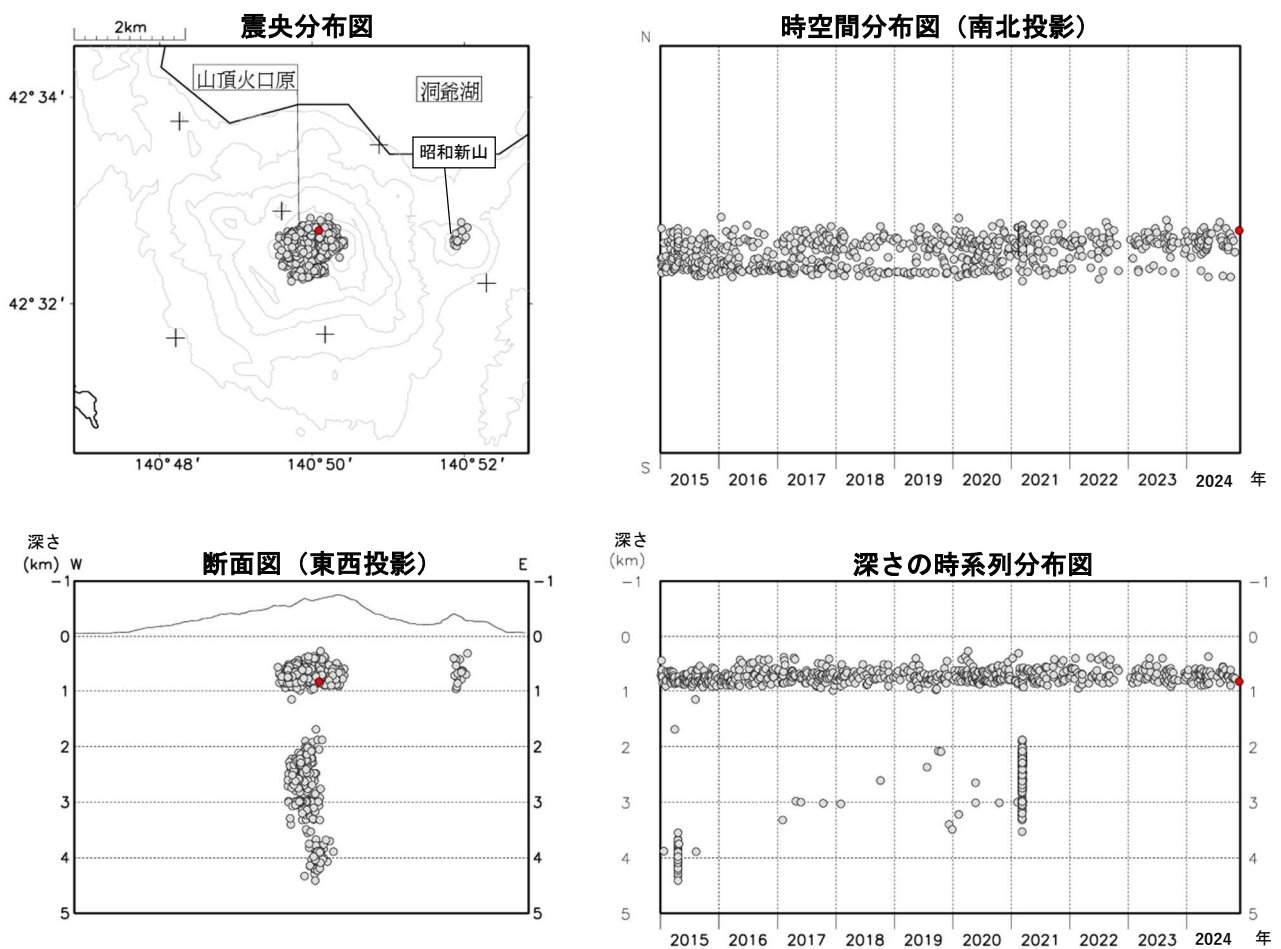
図3 有珠山 火山性地震の震源分布（2015年1月～2024年11月）
