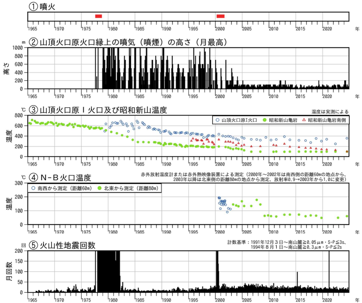
図1 有珠山 火山活動経過図（1965年1月～2024年11月）
