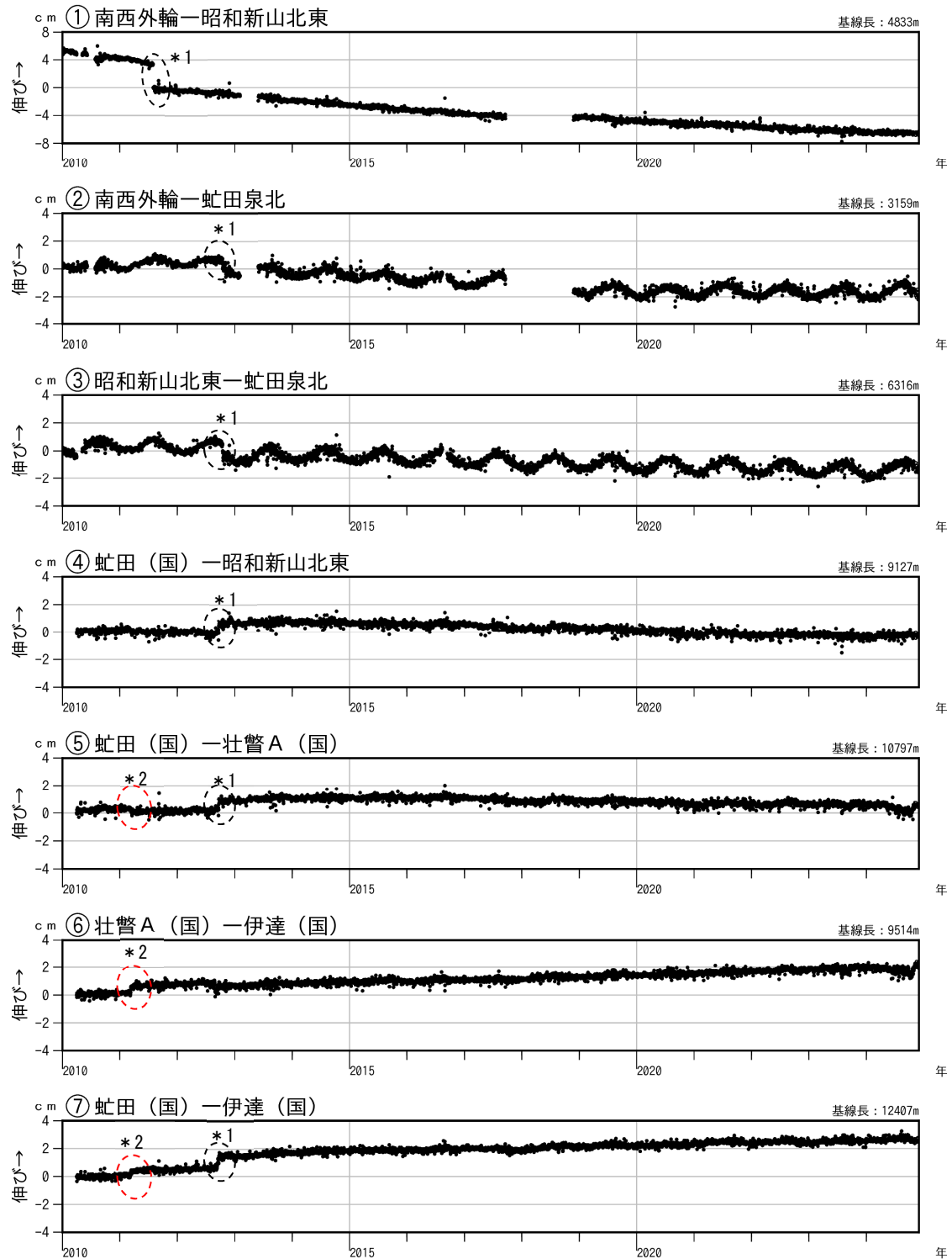
図4 有珠山 GNSS連続観測による基線長変化（2010年1月～2024年11月）
