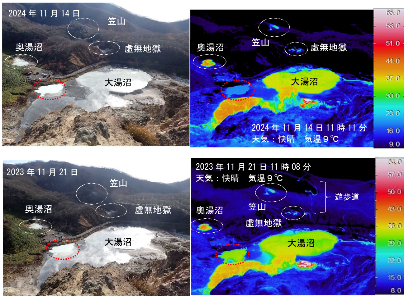
図6 倶多楽 笠山、虚無地獄、奥湯沼、大湯沼の地表面温度分布
