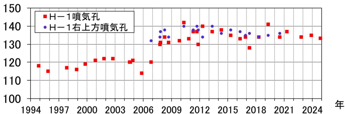
図5 倶多楽 日和山爆裂火口北西側噴気孔の噴気温度の推移（1994年～2024年） ・2007年以降、噴気温度は130°C以上の状態が継続しています。
