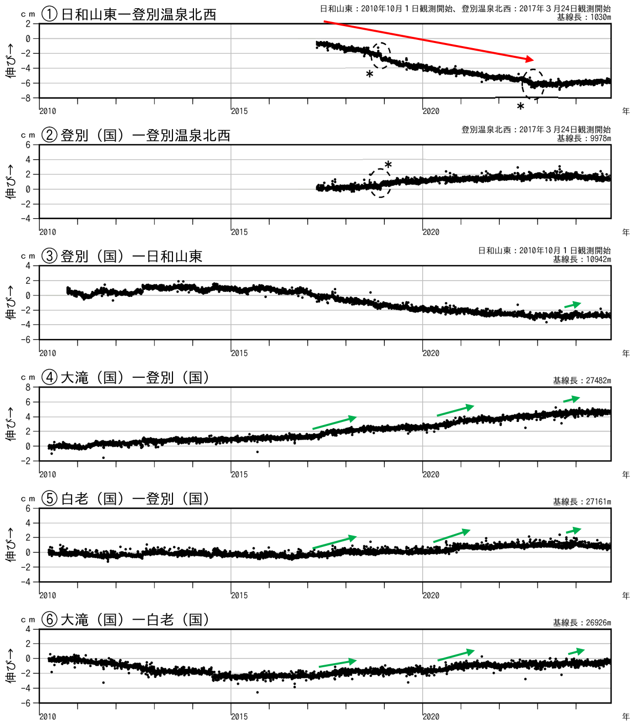
図7 倶多楽 GNSS連続観測による基線長変化（2010年4月～2024年11月）
