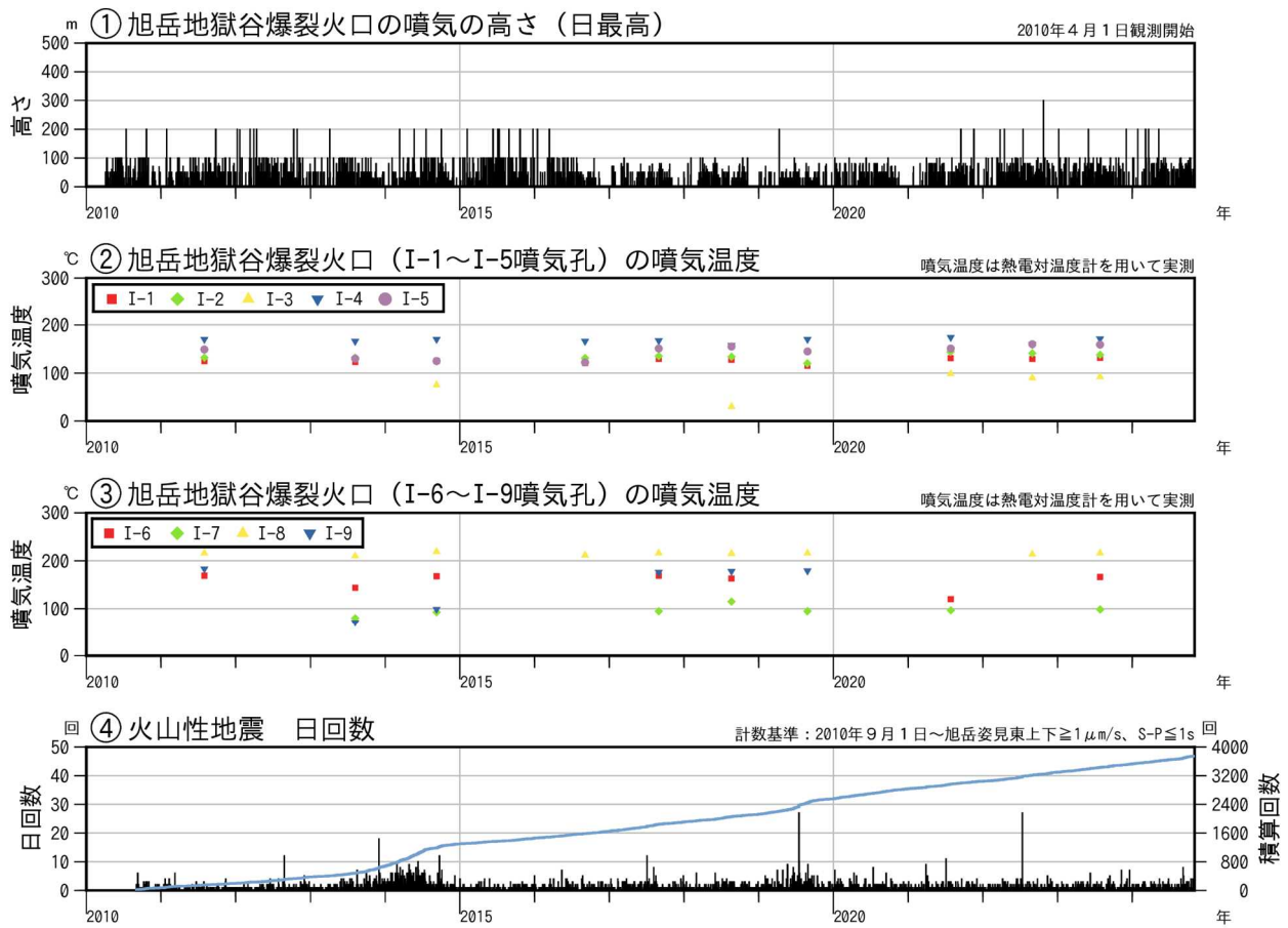
図2 大雪山 火山活動経過図（2010年4月～2024年10月）
