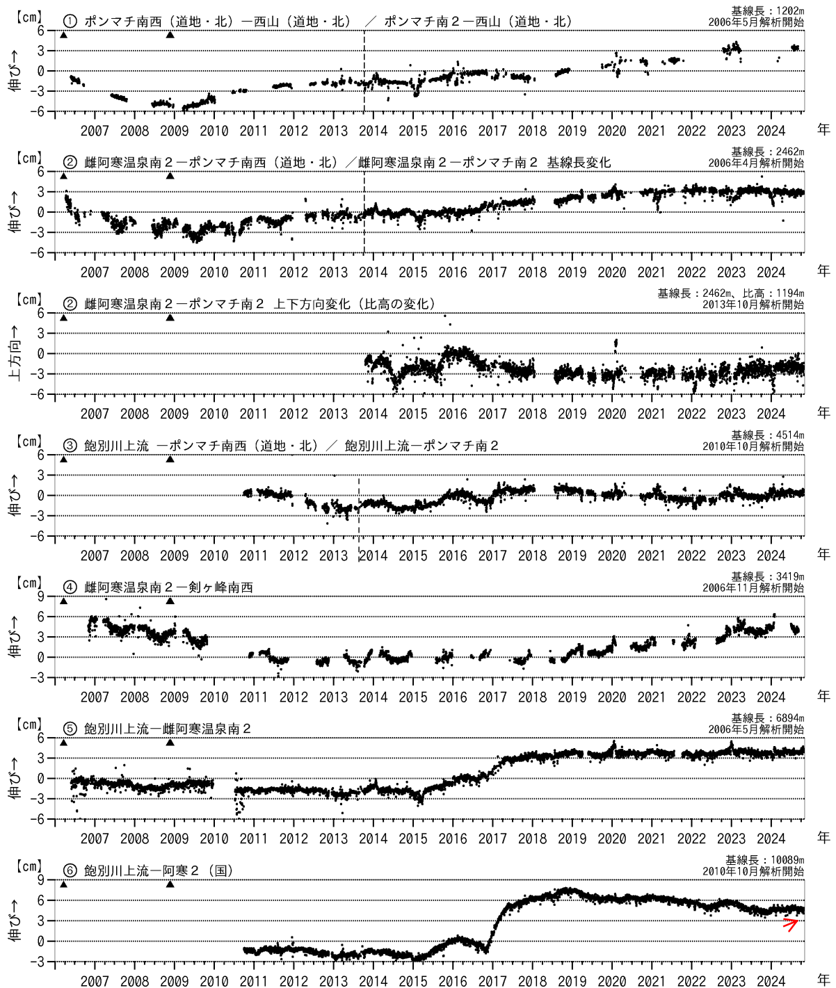
図8 雌阿寒岳 GNSS連続観測による基線長及び比高の変化（2006年4月～2024年10月）
