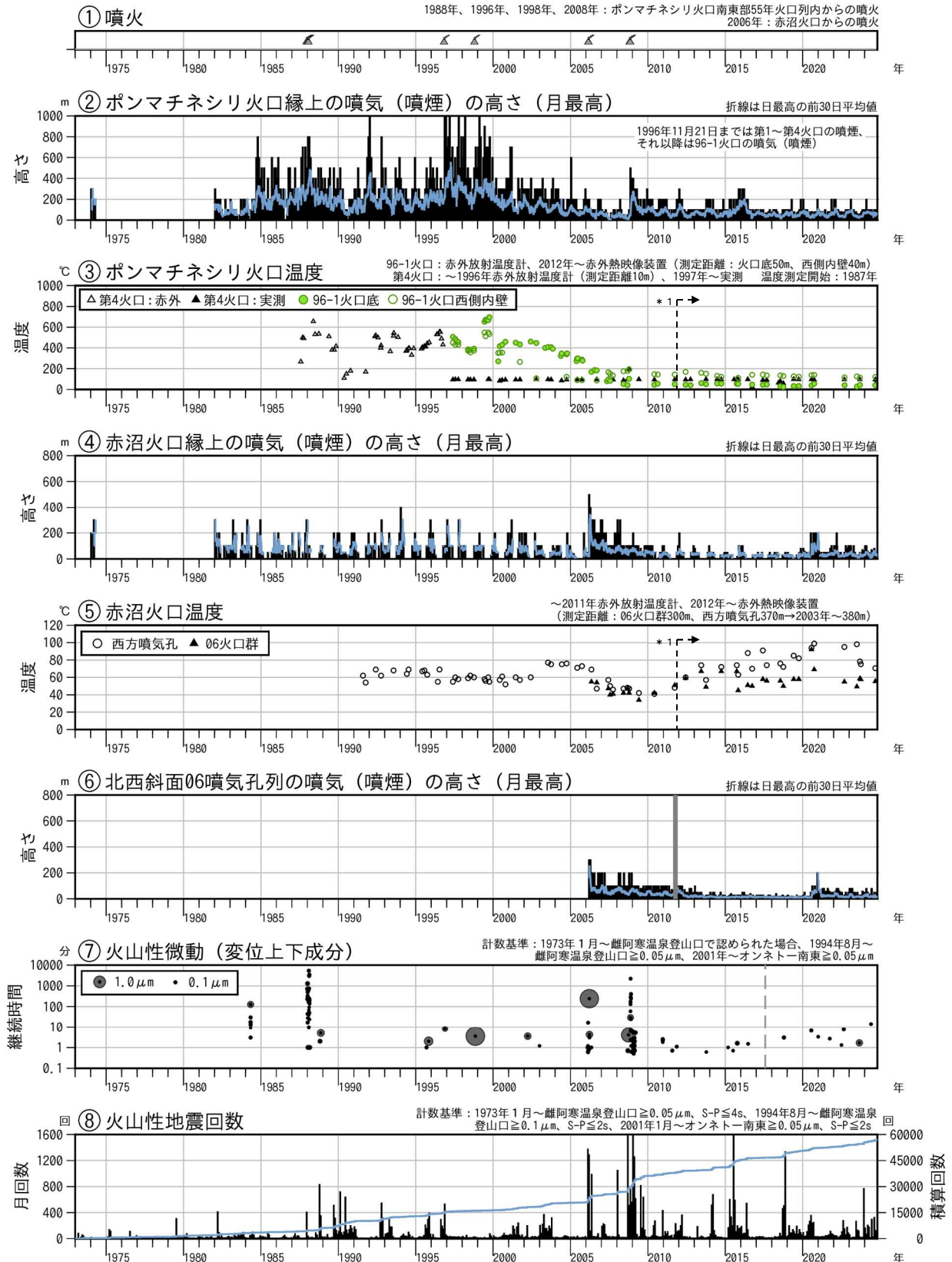
図2 雌阿寒岳 火山活動経過図（1973年1月～2024年10月）
