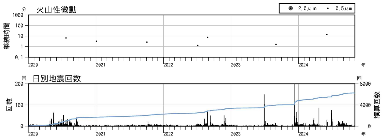
図6 雌阿寒岳 火山性微動の振幅、継続時間及び火山性地震の日別回数 (2020年1月～2024年10月)
