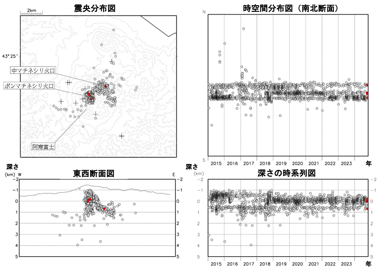
図7 雌阿寒岳 火山性地震の震源分布（2015年1月～2024年10月）
