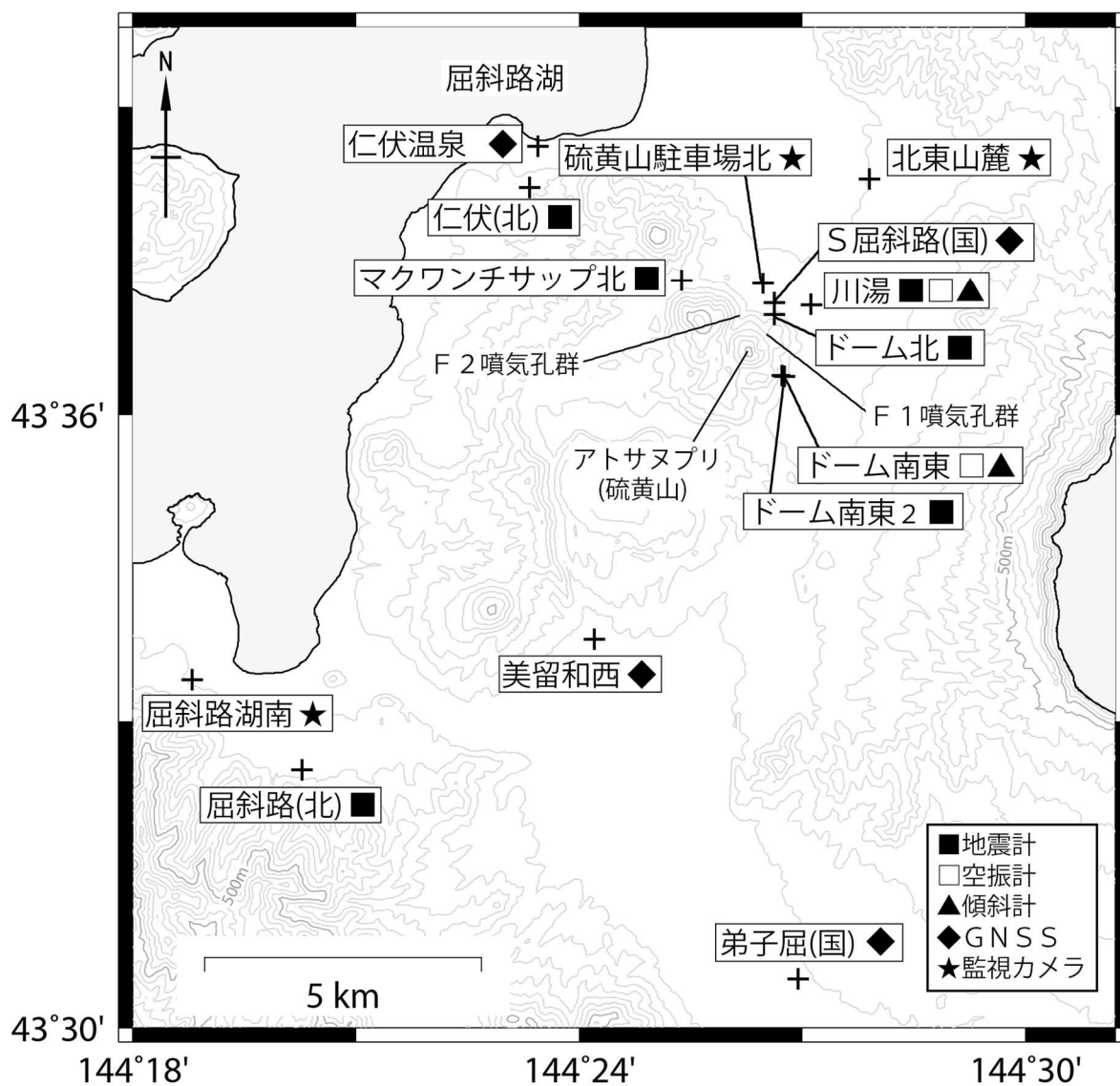
図9 アトサヌプリ 観測点配置図
