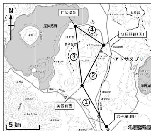
図8 アトサヌプリ GNSS連続観測による基線長変化（2010年10月～2024年10月）及び観測点配置図
