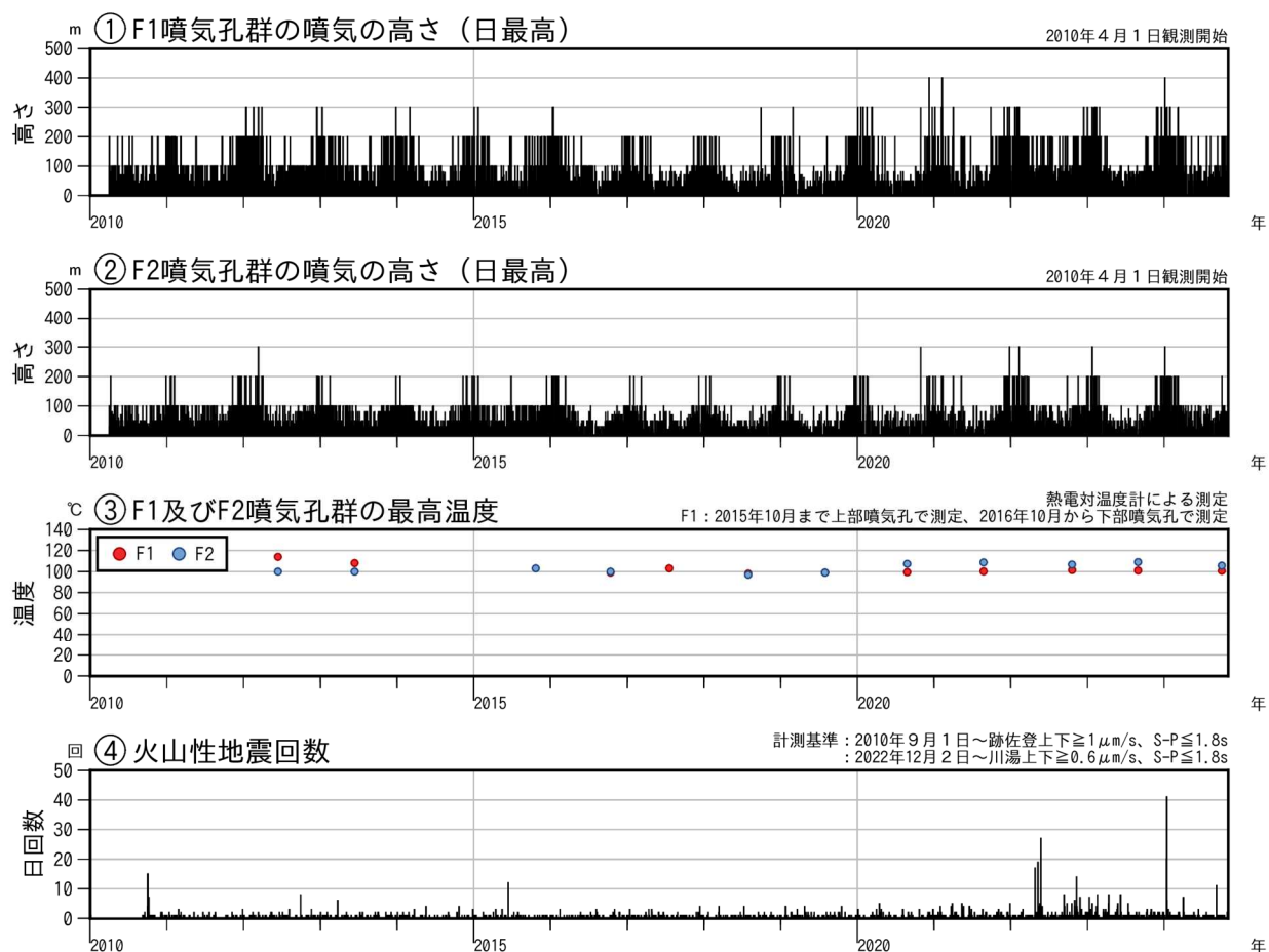
図1 アトサヌプリ 火山活動経過図（2010年4月～2024年10月）
