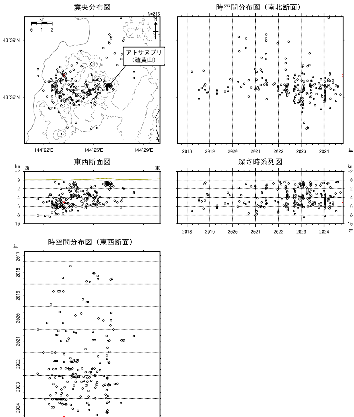
図7 アトサヌプリ 火山性地震の震源分布（2017年8月～2024年10月）
