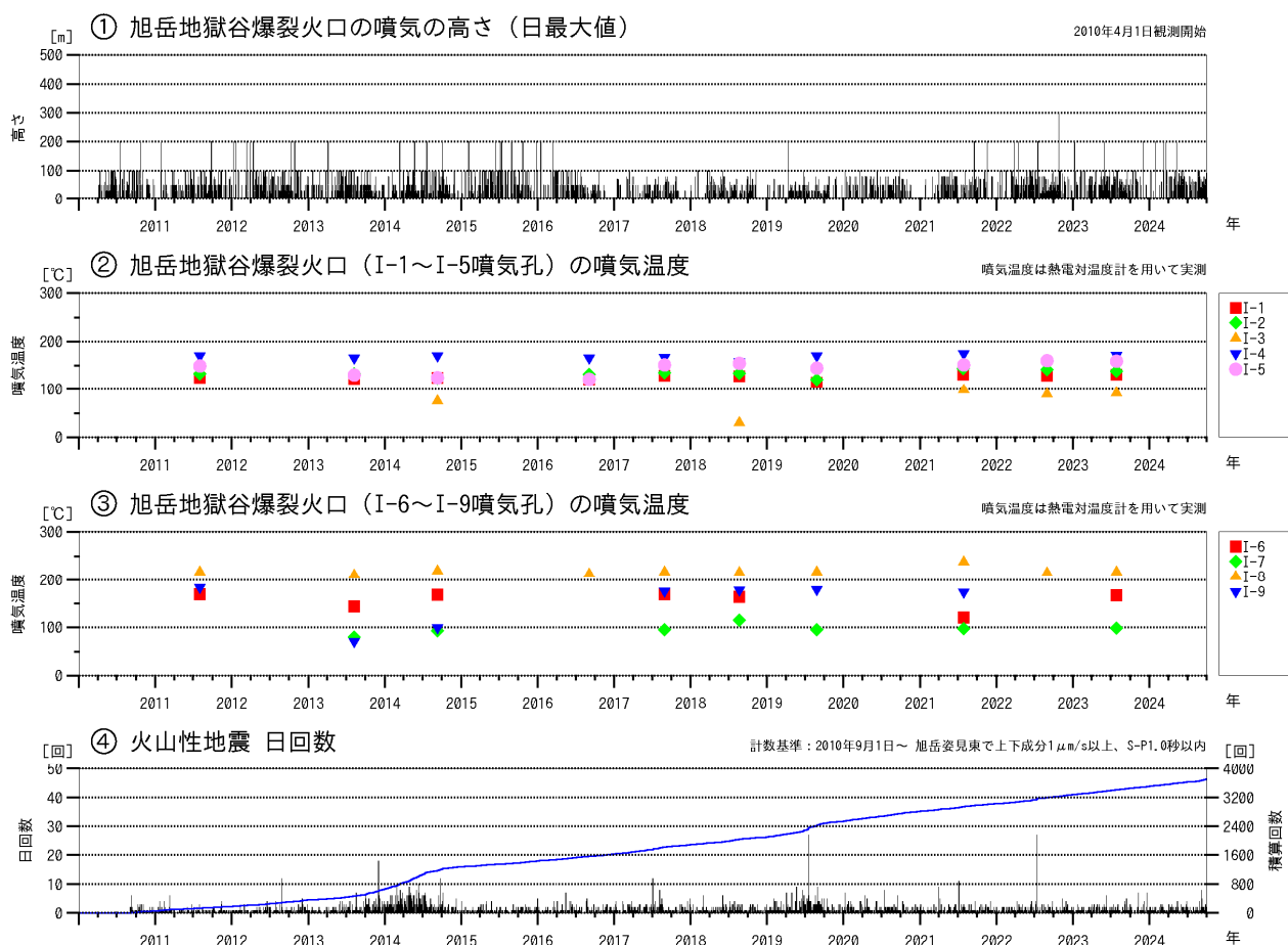
図2 大雪山 火山活動経過図（2010年4月～2024年9月）
