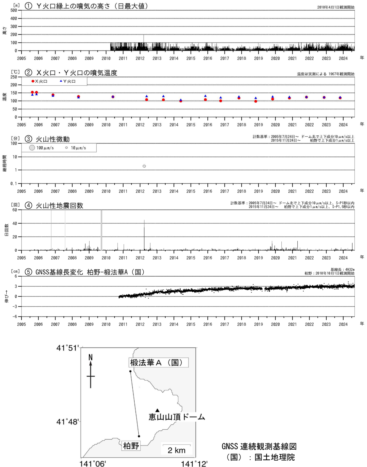
図2 恵山 火山活動経過図（2005年7月～2024年8月） ④の灰色部分は機器障害による欠測期間を示します。 ⑤のグラフは上図の基線に対応しています。 ⑤のグラフの空白部分は欠測を示します。
