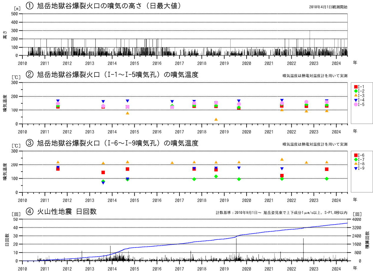
図2 大雪山 火山活動経過図（2010年4月～2024年6月）
