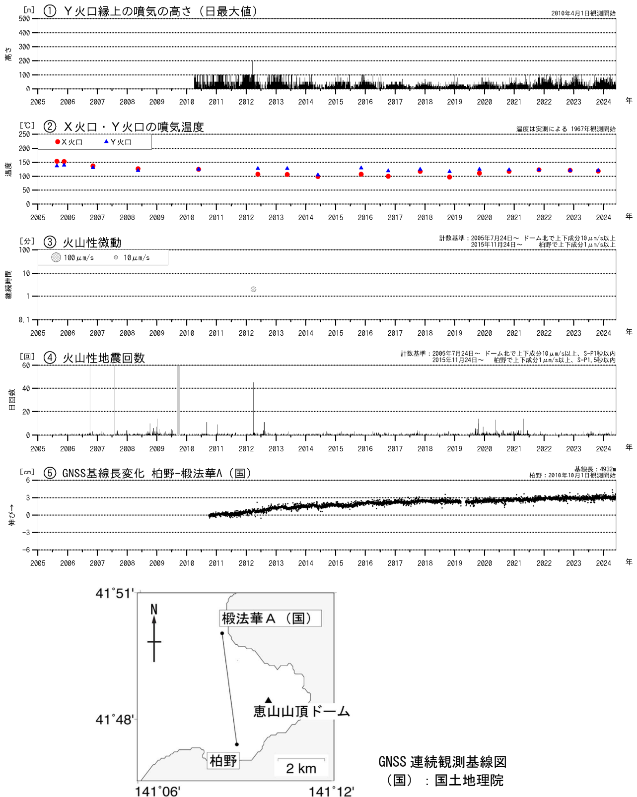
図2 恵山 火山活動経過図（2005年7月～2024年5月） ④の灰色部分は機器障害による欠測期間を示します。 ⑤のグラフは上図の基線に対応しています。 ⑤のグラフの空白部分は欠測を示します。
