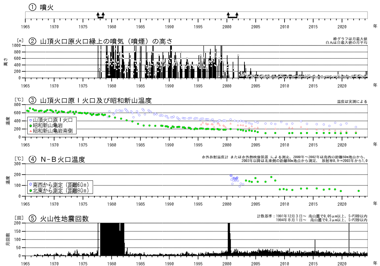
図1 有珠山 火山活動経過図（1965年1月～2024年5月）
