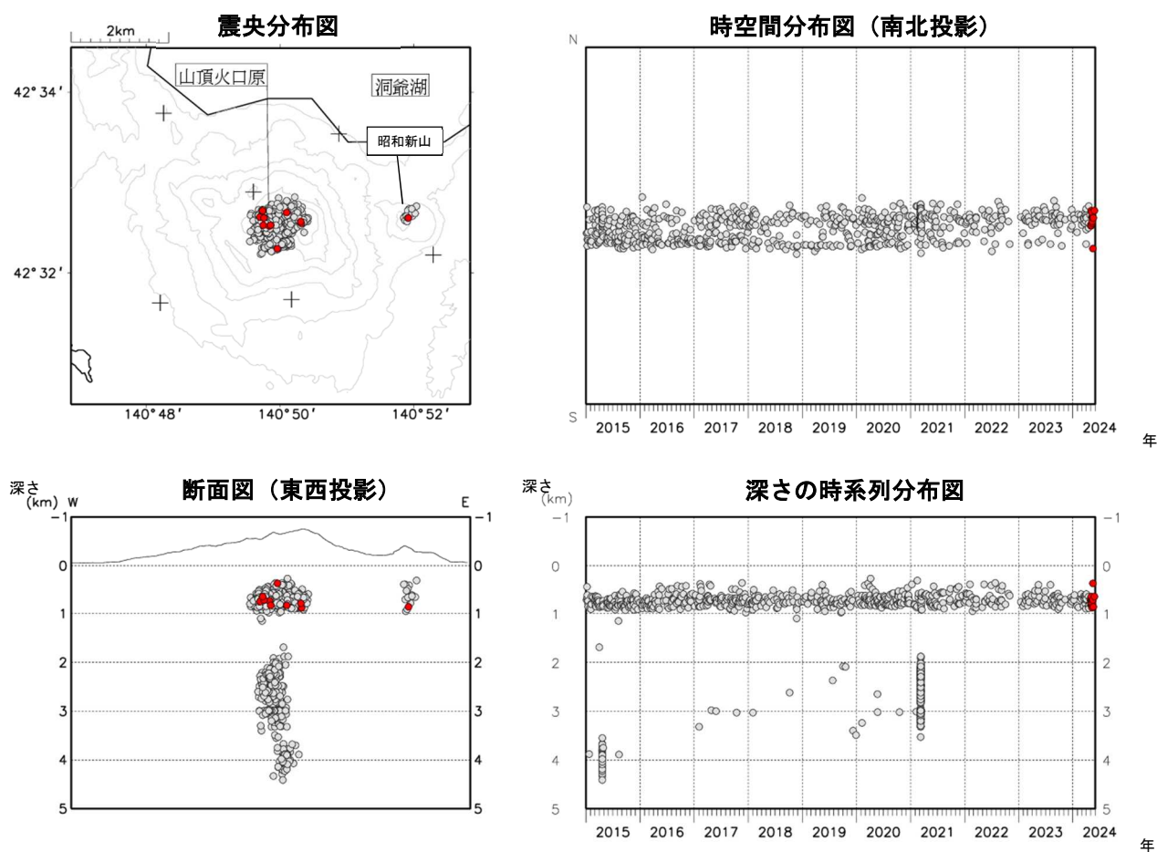
図3 有珠山 火山性地震の震源分布（2015年1月～2024年5月）
