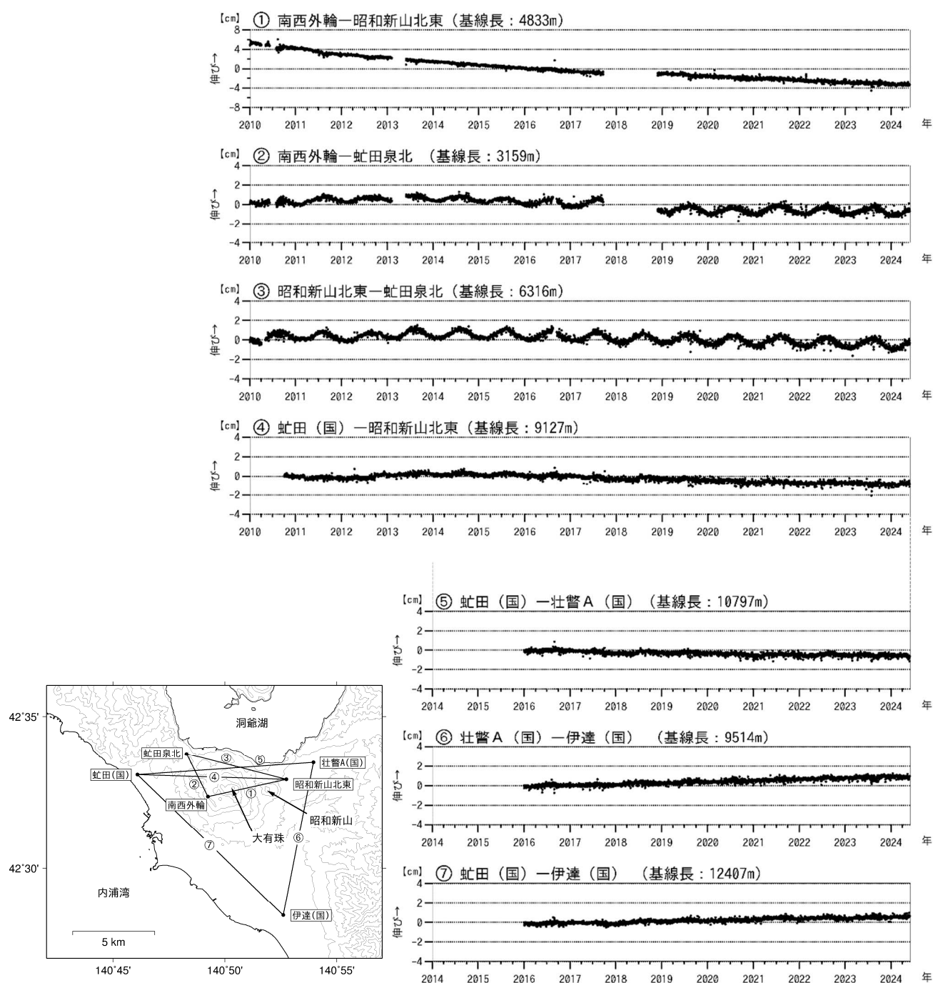
図4 有珠山 GNSS連続観測による基線長変化（2010年1月～2024年5月）及び観測点配置図 グラフ①～⑦は観測点配置図の基線①～⑦に対応しています。 グラフの空白部分は欠測を示します。
