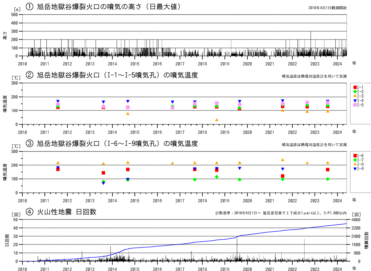
図2 大雪山 火山活動経過図（2010年4月～2024年5月）
