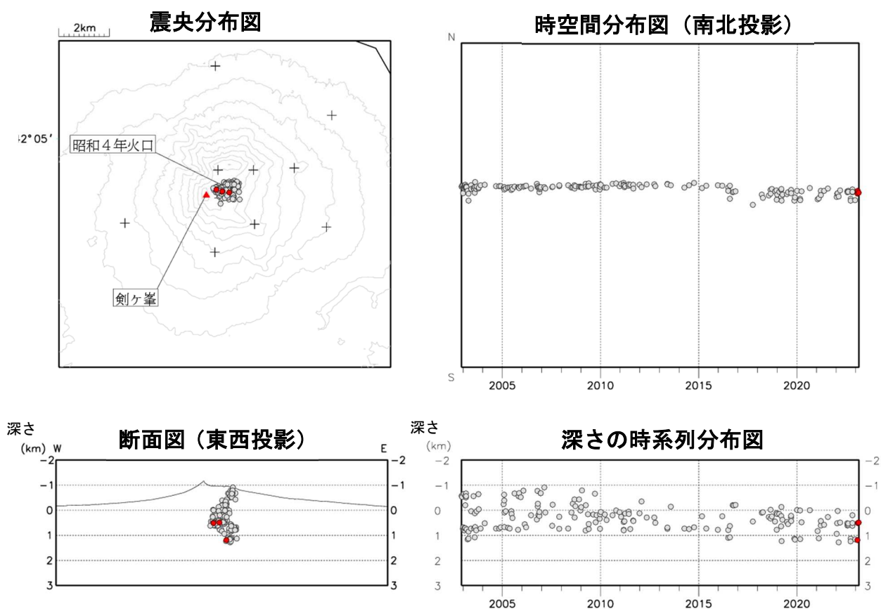
図4 北海道駒ヶ岳 火山性地震の震源分布（2002年12月～2023年2月）
