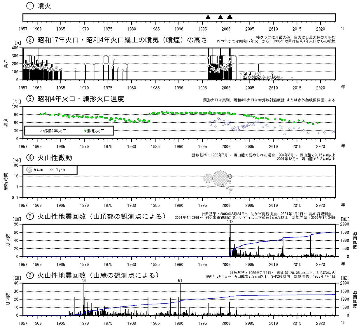
図1 北海道駒ヶ岳 火山活動経過図（1957年1月～2023年2月）
