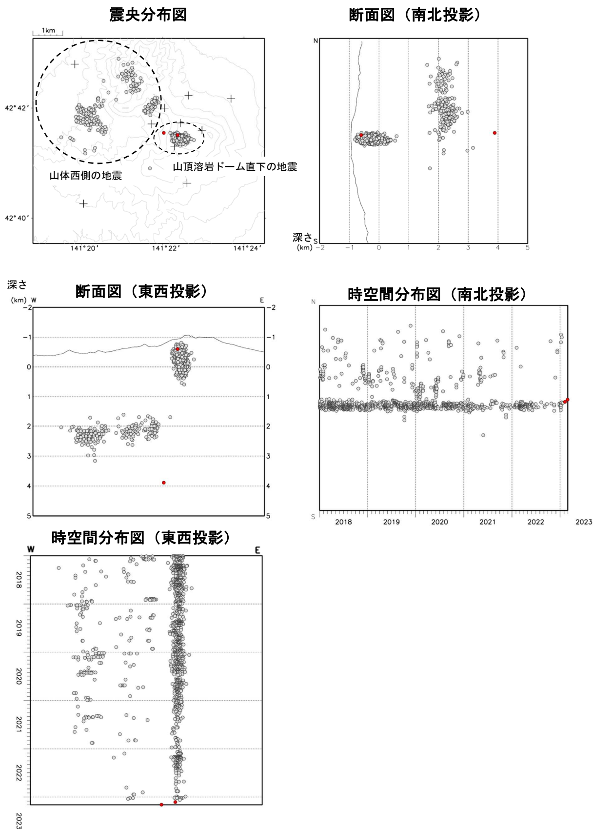
図3 樽前山 火山性地震の震源分布（2018年1月～2023年2月） ○：2018年1月～2023年1月の震源 ●：2023年2月の震源 ＋：地震観測点
