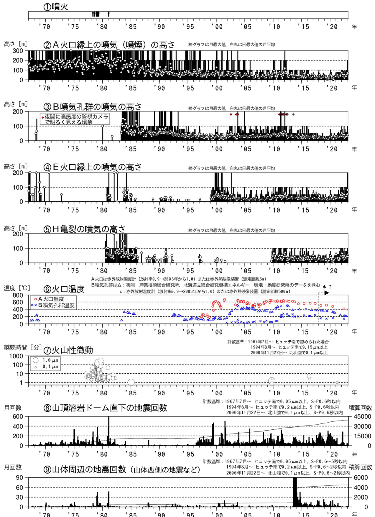
図2 樽前山 火山活動経過図(1967年1月～2023年2月)
