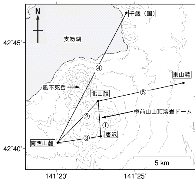
図4 樽前山 GNSS連続観測による基線長変化（2005年1月～2023年2月）及び観測点配置図
