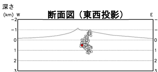
図4 北海道駒ヶ岳 火山性地震の震源分布（2002年12月～2022年11月）
