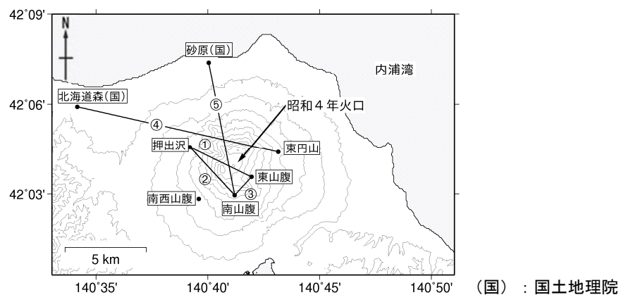
図5 北海道駒ヶ岳 GNSS連続観測による基線長変化（2001年4月～2022年11月）及び観測点配置図 グラフ①～⑤は観測点配置図の基線①～⑤に対応しています。 グラフの空白部分は欠測を示します。
