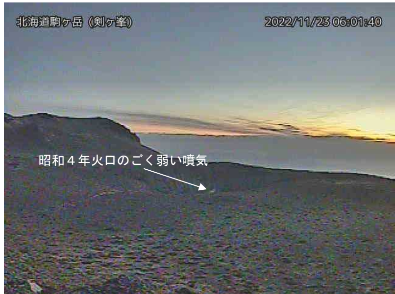
図3 北海道駒ヶ岳 西南西側から見た火口周辺の状況 (剣ヶ峯監視カメラによる)
