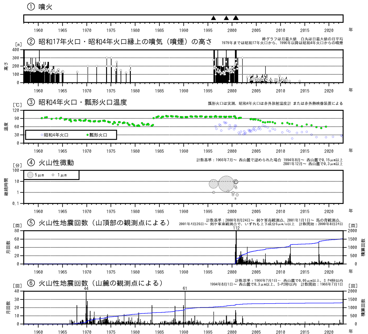
図1 北海道駒ヶ岳 火山活動経過図（1957年1月～2022年11月）
