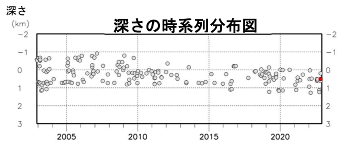
図4 北海道駒ヶ岳 火山性地震の震源分布（2002年12月～2022年11月）
