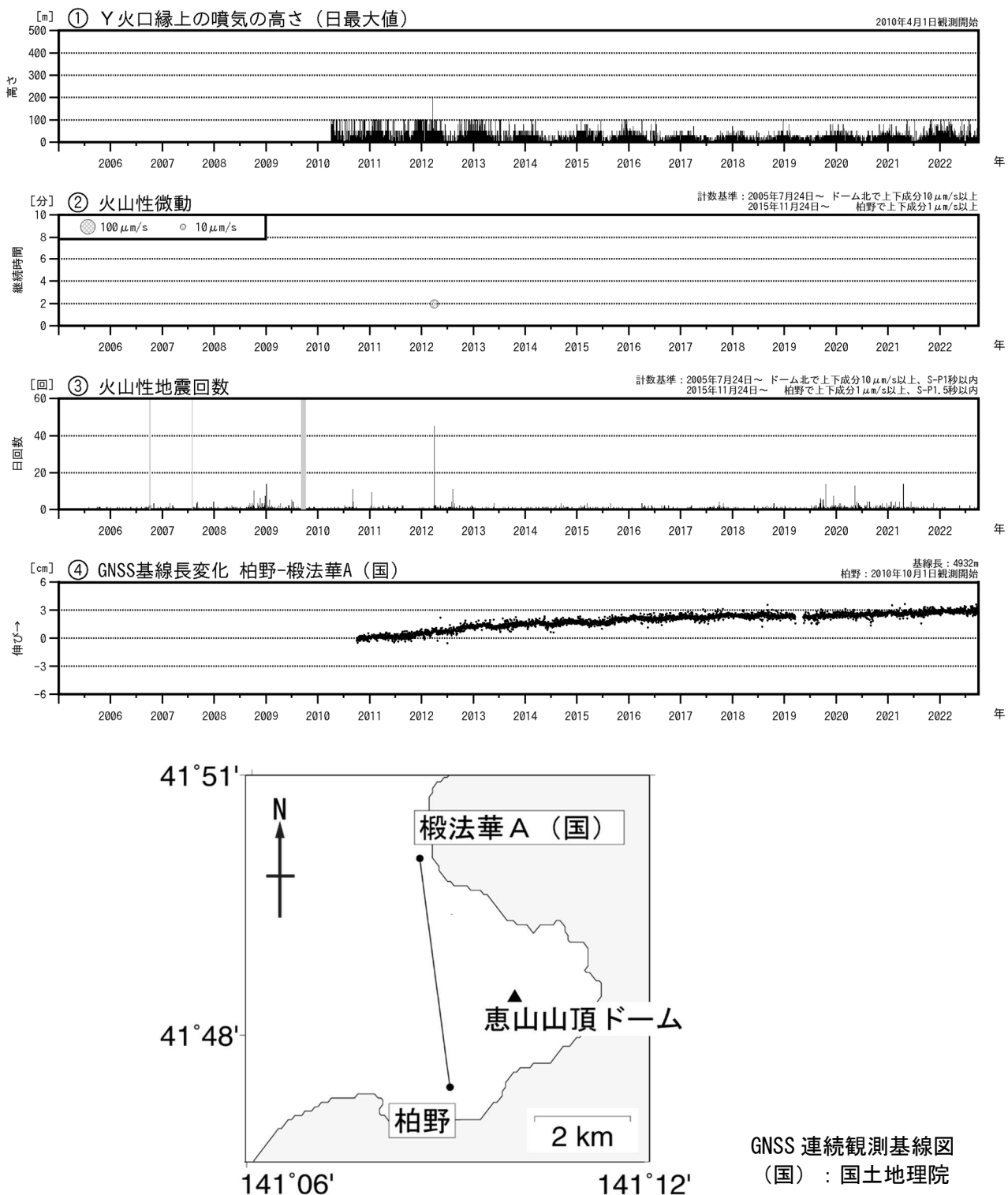
図2 恵山 火山活動経過図（2005年7月～2022年9月） ③の灰色部分は機器障害による欠測期間を示します。 ④のグラフは上図の基線に対応しています。 ④のグラフの空白部分は欠測を示します。
