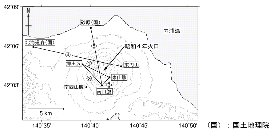
図5 北海道駒ヶ岳 GNSS連続観測による基線長変化（2001年4月～2022年9月）及び観測点配置図 グラフ①～⑤は観測点配置図の基線①～⑤に対応しています。 グラフの空白部分は欠測を示します。
