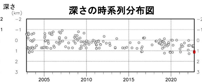
図4 北海道駒ヶ岳 火山性地震の震源分布（2002年12月～2022年9月）
