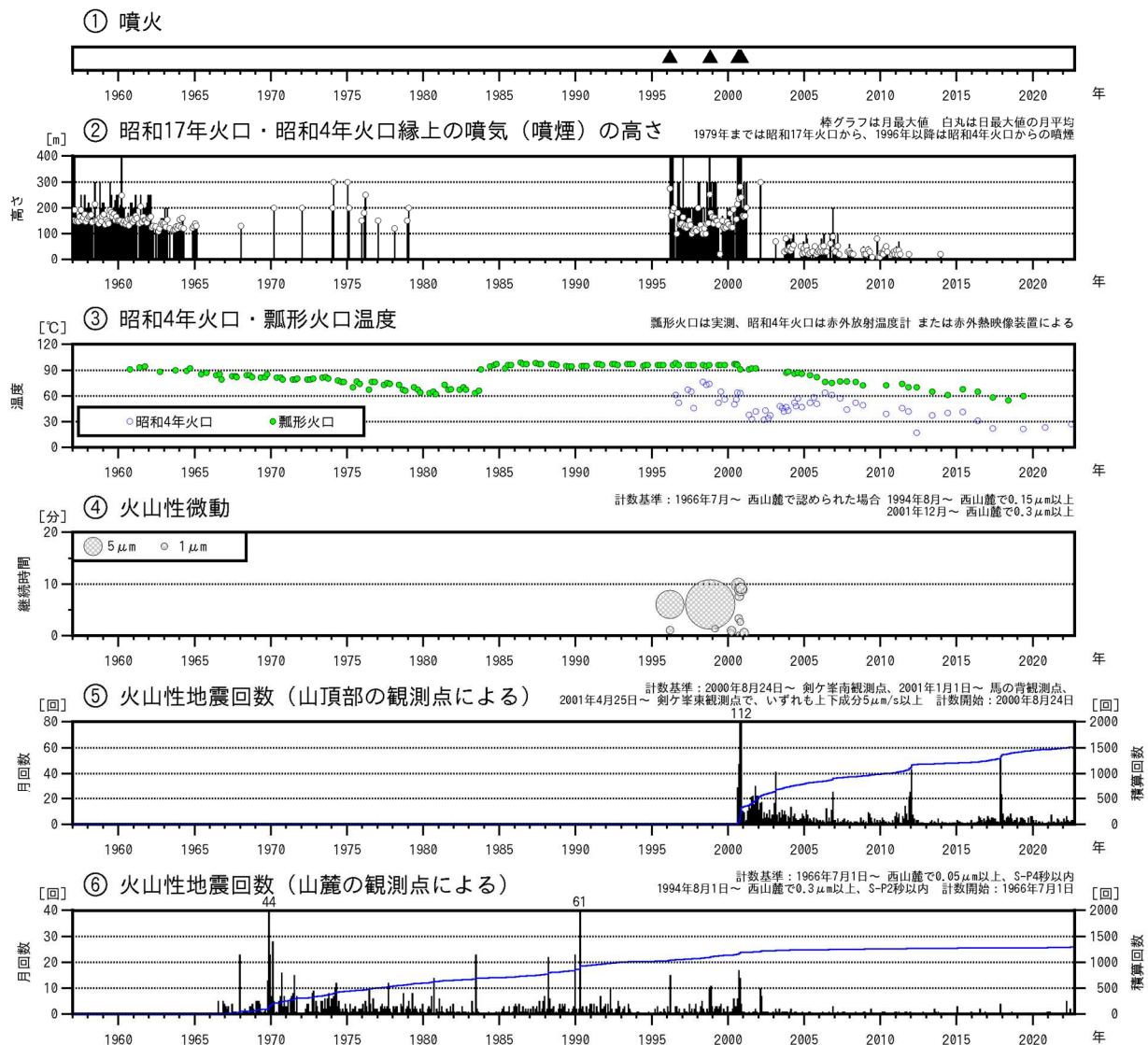
図1 北海道駒ヶ岳 火山活動経過図（1957年1月～2022年9月）
