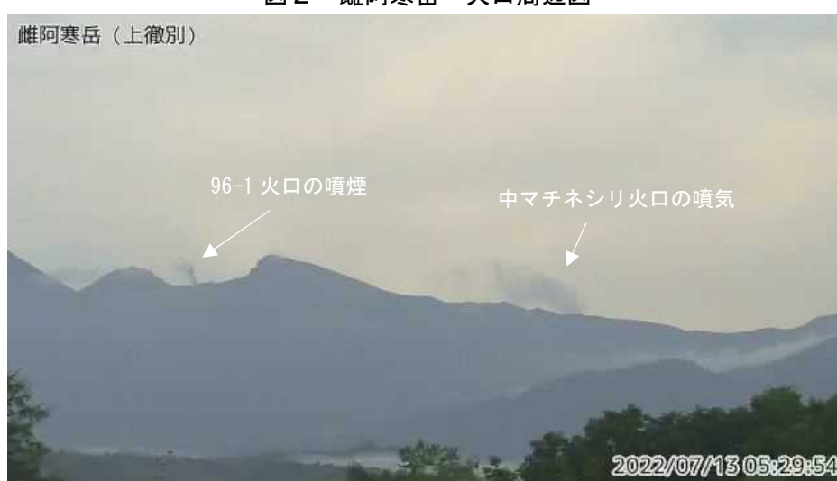
図3 雌阿寒岳 南東側から見た赤沼火口、96-1 火口及び中マチネシリ火口の状況 (上徹別監視カメラによる)
