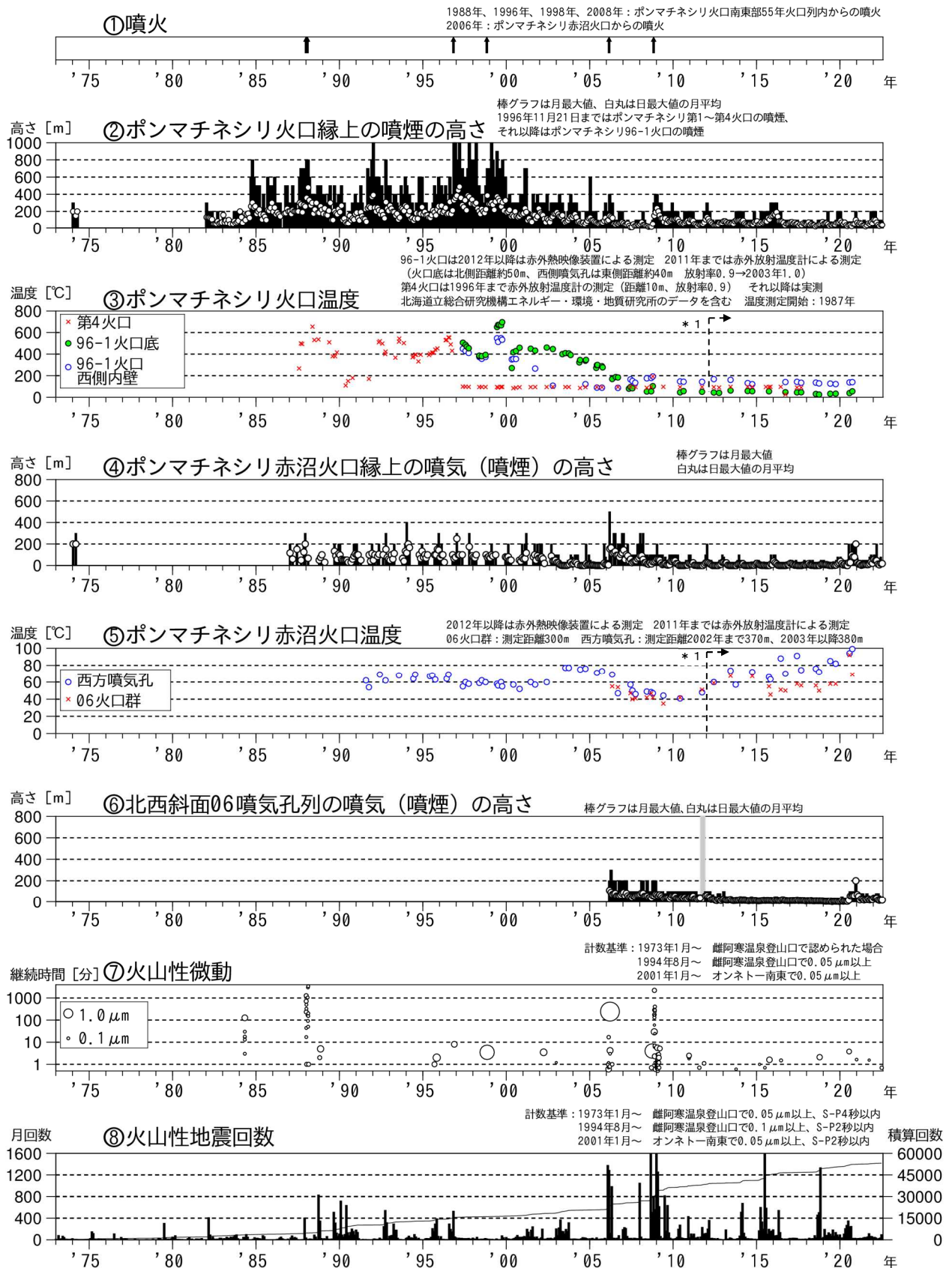
図1 雌阿寒岳 火山活動経過図（1973年1月～2022年7月）
