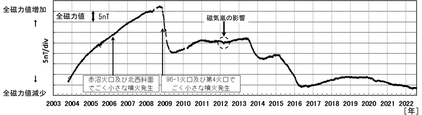
図5 雌阿寒岳 ポンマチネシリ96-1火口の噴煙の長さ と全磁力値の経過及び全磁力観測点配置図 (2003年～2022年7月)
