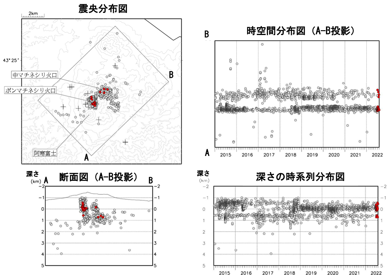
図6 雌阿寒岳 火山性地震の震源分布（2015年1月～2022年7月） ●印：2015年1月～2022年6月の震源 ●印：2022年7月の震源 ＋印：地震観測点
