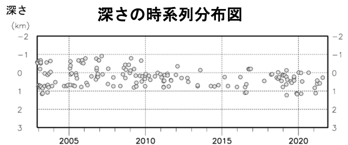
図4 北海道駒ヶ岳 火山性地震の震源分布（2002年12月～2021年11月）
