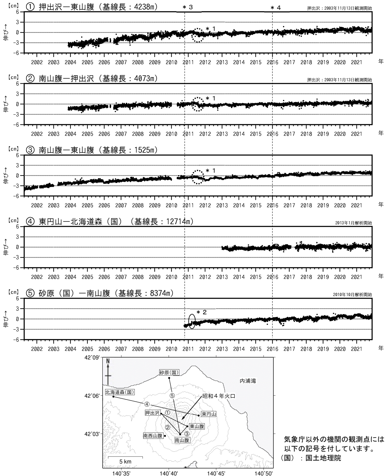
図5 北海道駒ヶ岳 GNSS連続観測による基線長変化（2001年4月～2021年11月）及び観測点配置図
