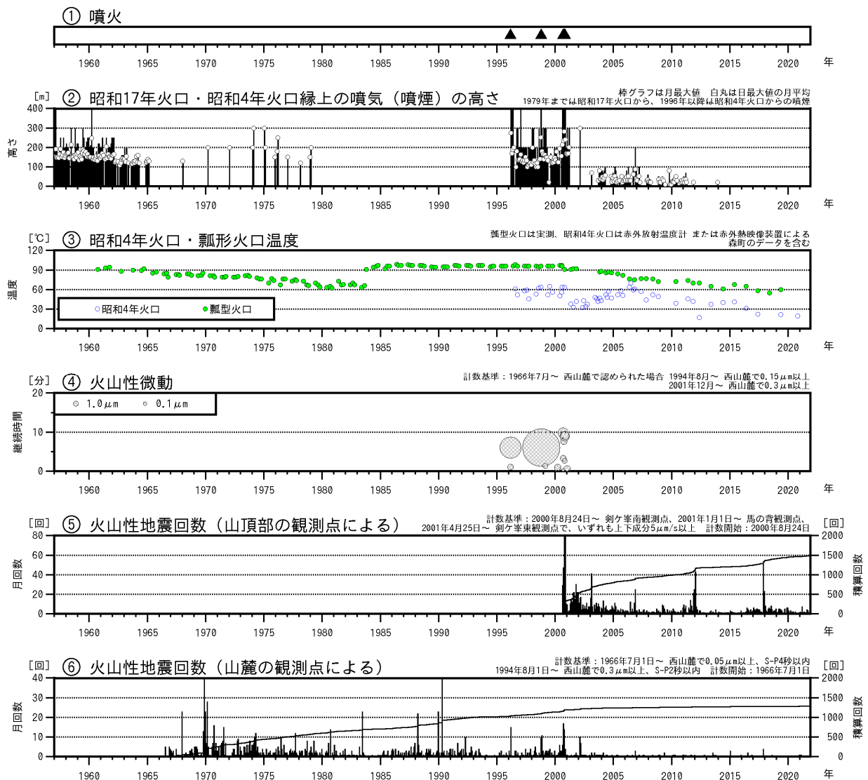
図1 北海道駒ヶ岳 火山活動経過図（1957年1月～2021年11月）
