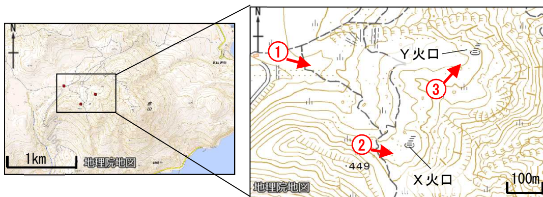
図5 恵山 写真及び赤外熱映像の撮影方向（赤矢印）
