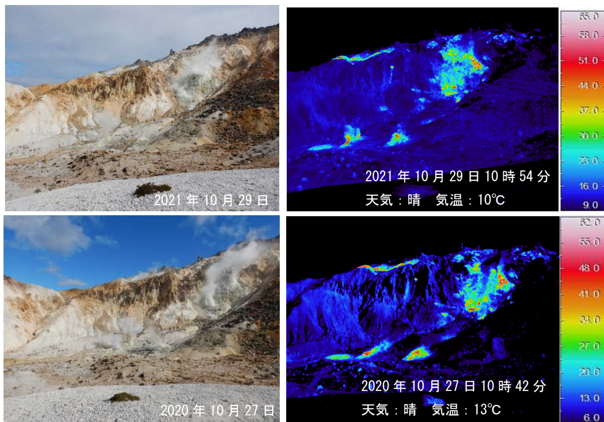
図8 恵山 赤外熱映像装置によるY火口内の地表面温度分布
