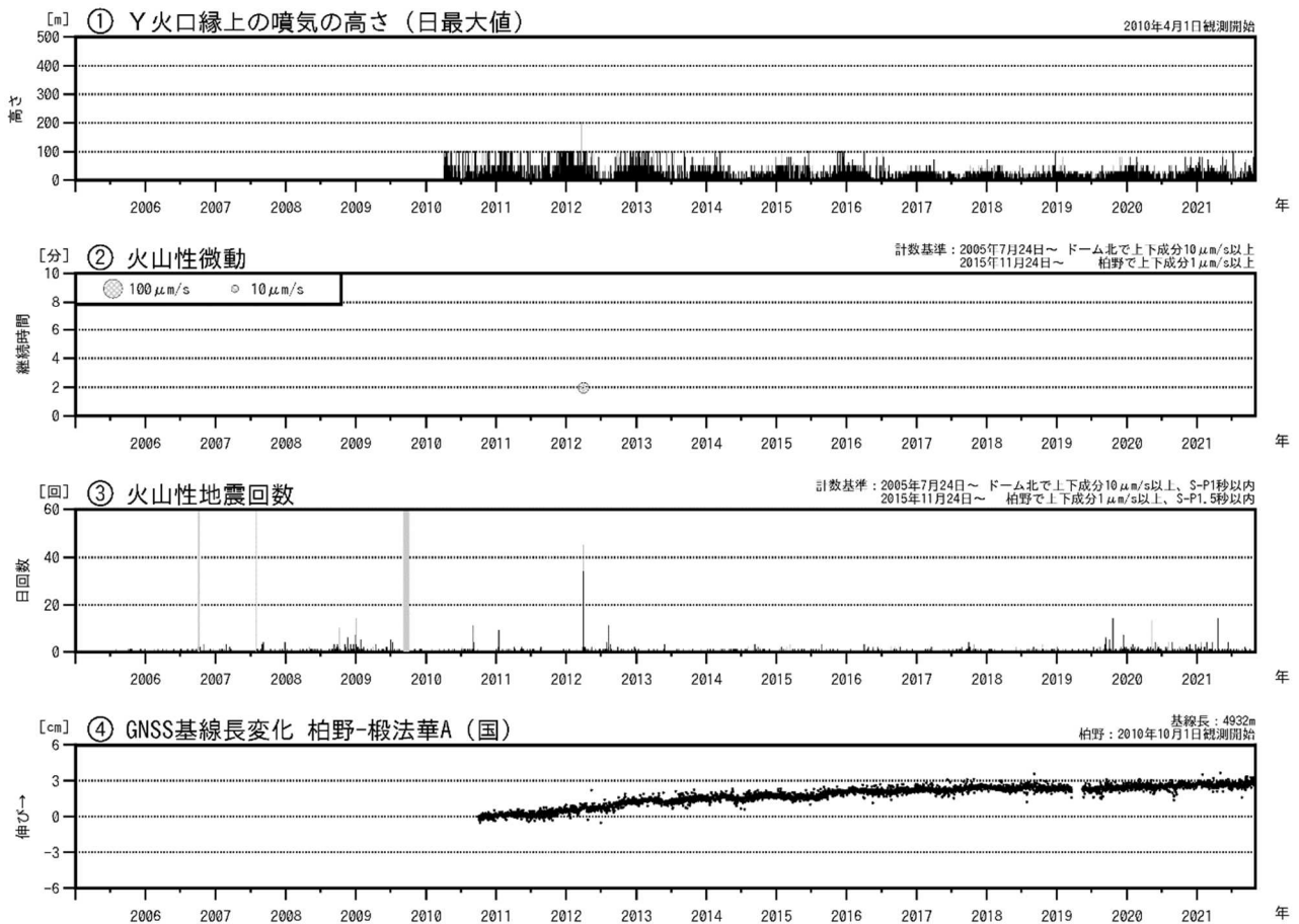
図2 恵山 火山活動経過図（2005年7月～2021年10月）
