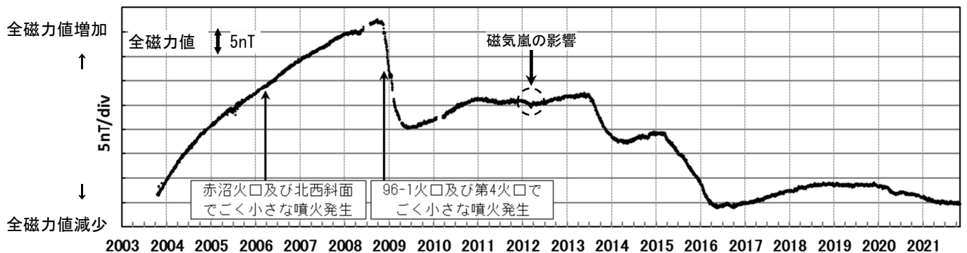
図6 雌阿寒岳 ポンマチネシリ96-1火口の噴煙の長さ（2003年～2021年10月）と全磁力の比較及び全磁力観測点配置図
