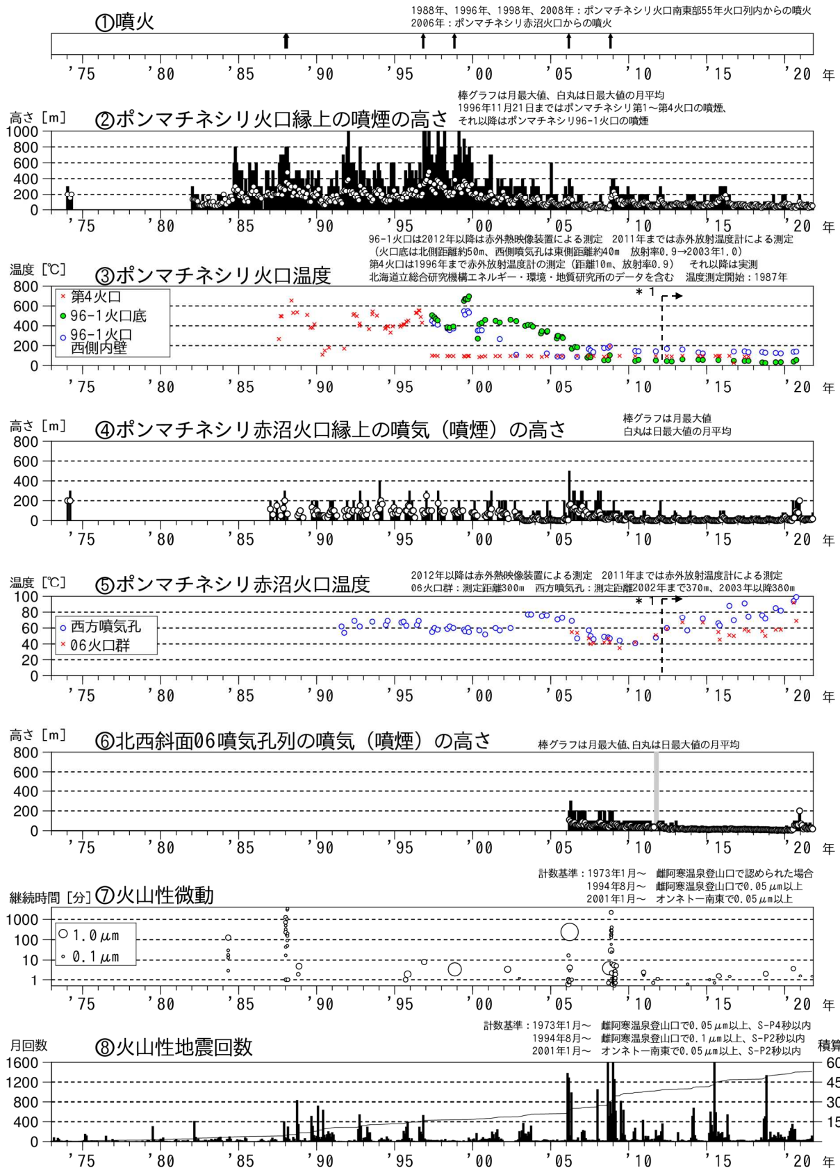
図1 雌阿寒岳 火山活動経過図（1973年1月～2021年10月）
