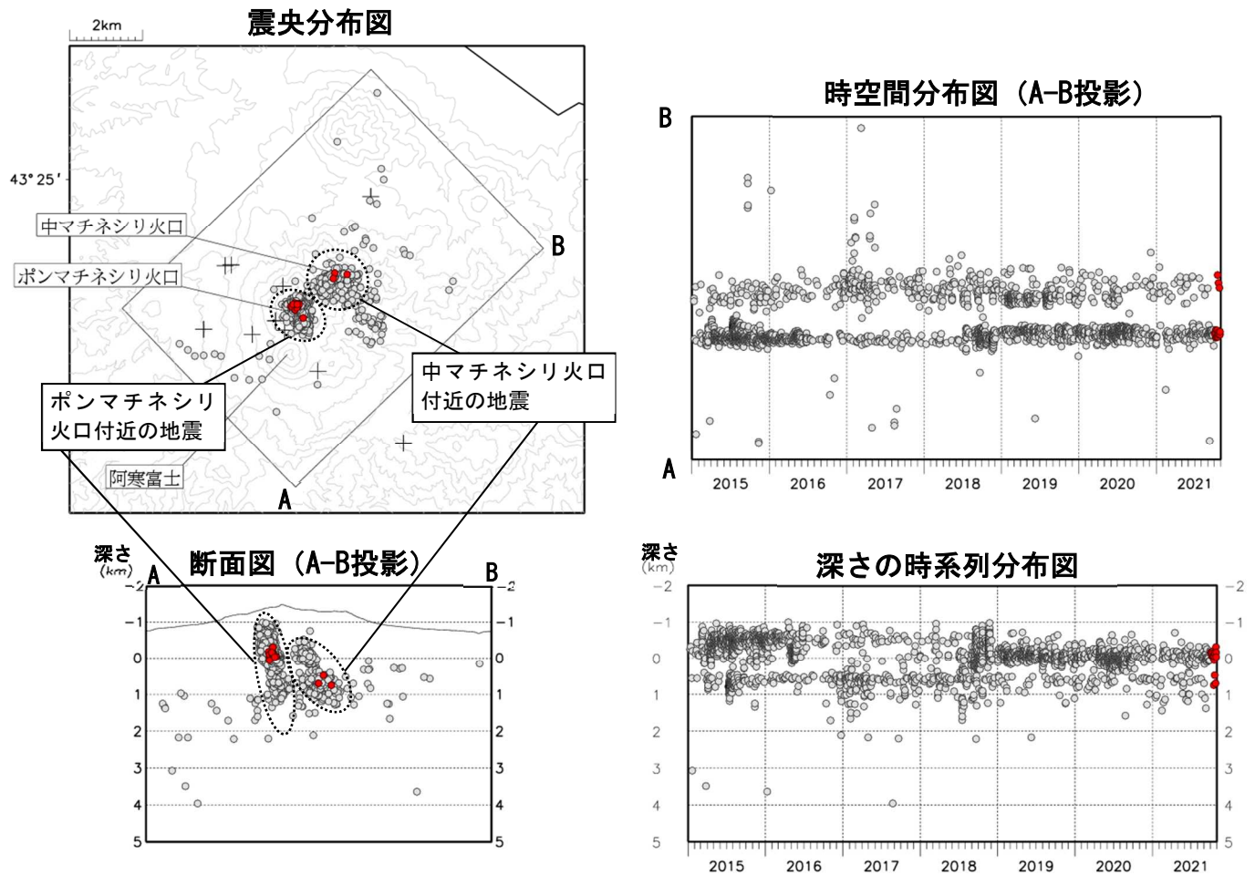
図7 雌阿寒岳 火山性地震の震源分布（2015年1月～2021年10月）
