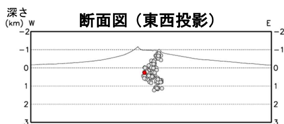
図4 北海道駒ヶ岳 火山性地震の震源分布（2002年12月～2021年8月）
