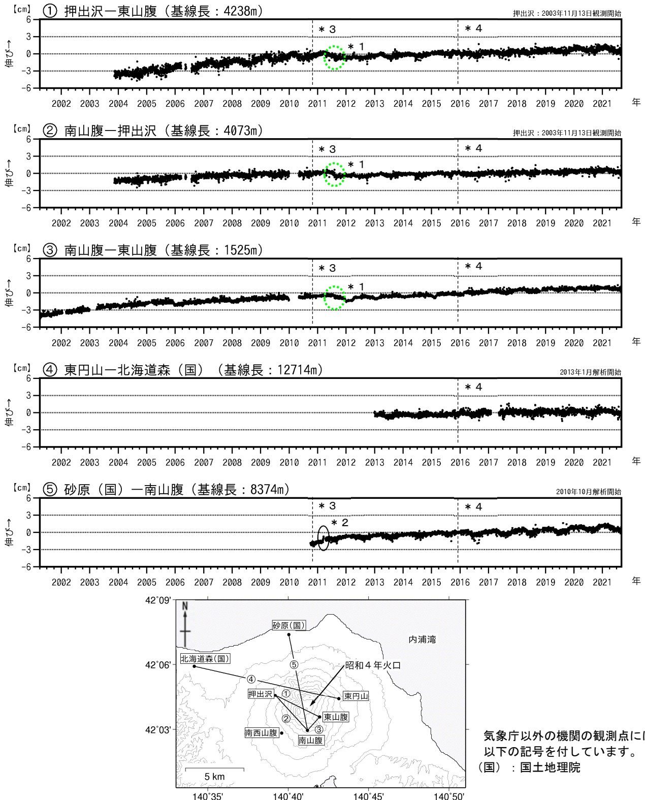
図5 北海道駒ヶ岳 GNSS連続観測による基線長変化（2001年4月～2021年8月）及び観測点配置図
