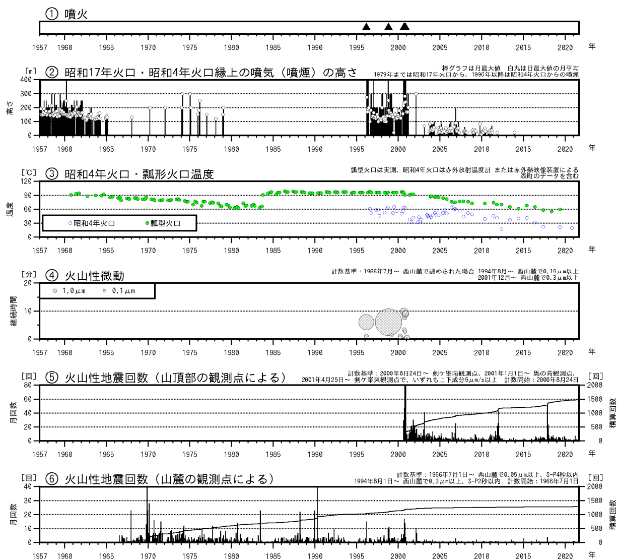
図1 北海道駒ヶ岳 火山活動経過図（1957年1月～2021年8月）
