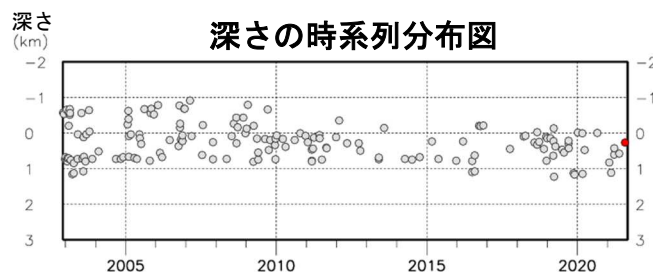
図4 北海道駒ヶ岳 火山性地震の震源分布（2002年12月～2021年8月）
