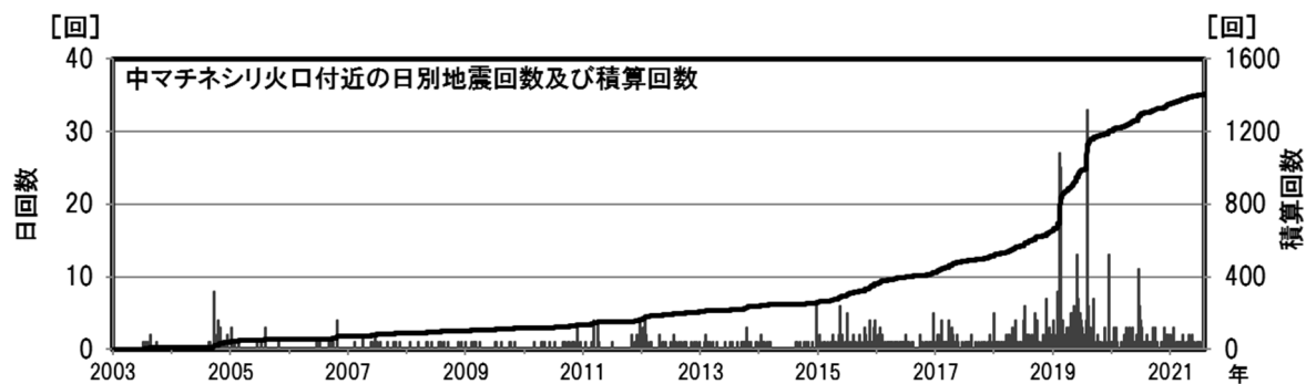
図8 雌阿寒岳 中マチネシリ火口付近の日別地震回数（2003年～2021年7月）
