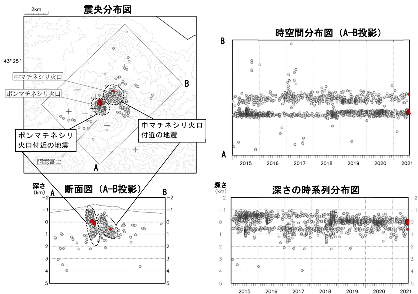
図9 雌阿寒岳 火山性地震の震源分布（2015年1月～2021年7月）
