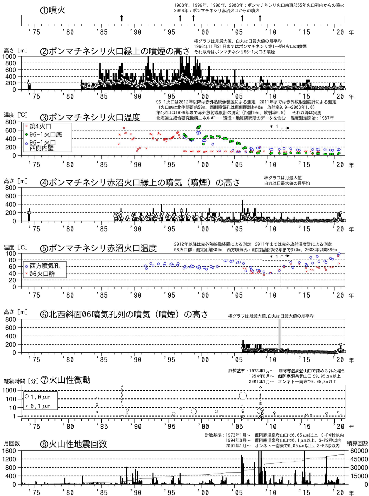
図1 雌阿寒岳 火山活動経過図（1973年1月～2021年7月）
