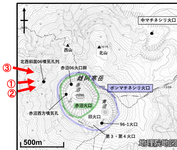
図2 雌阿寒岳 火口周辺図および写真の撮影方向（矢印）
