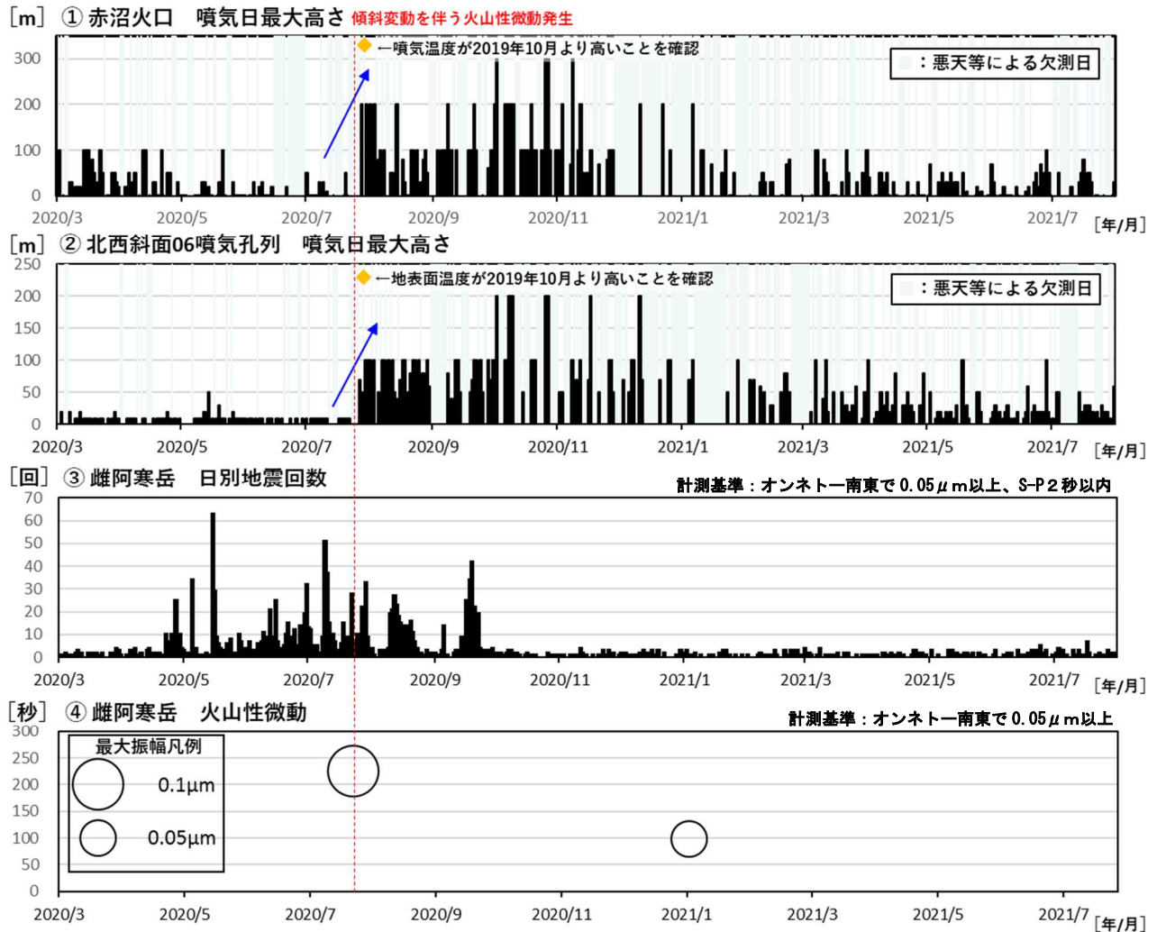
図6 雌阿寒岳 2020年7月以降の噴気活動及び地震活動等の活動経過（2020年3月～2021年7月） ・2020年7月22日の火山性微動発生後に活発化が確認された赤沼火口及び北西斜面06噴気孔列の噴気活動（①、②の青矢印）は、2020年12月以降低下傾向が続いています。
