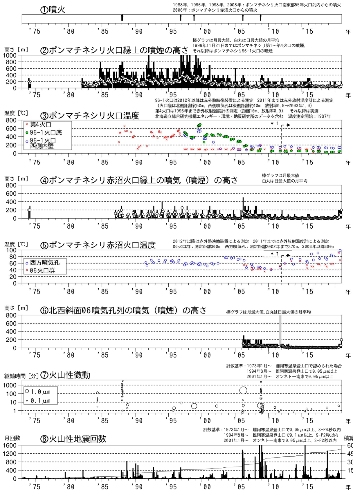
図1 雌阿寒岳 火山活動経過図（1973年1月～2020年12月）
