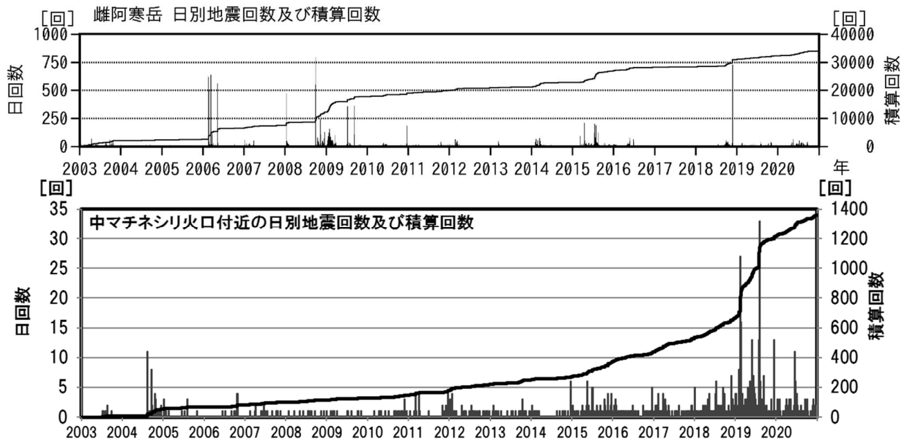
図6 雌阿寒岳 中マチネシリ火口付近の日別地震回数（2003年～2020年12月）
