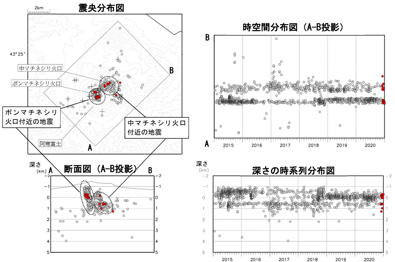
図7 雌阿寒岳 火山性地震の震源分布（2015年1月～2020年12月）
