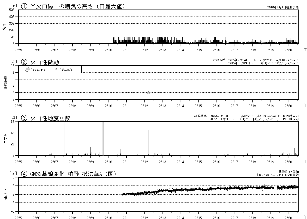
図2 恵山 火山活動経過図（2005年7月～2020年7月）
