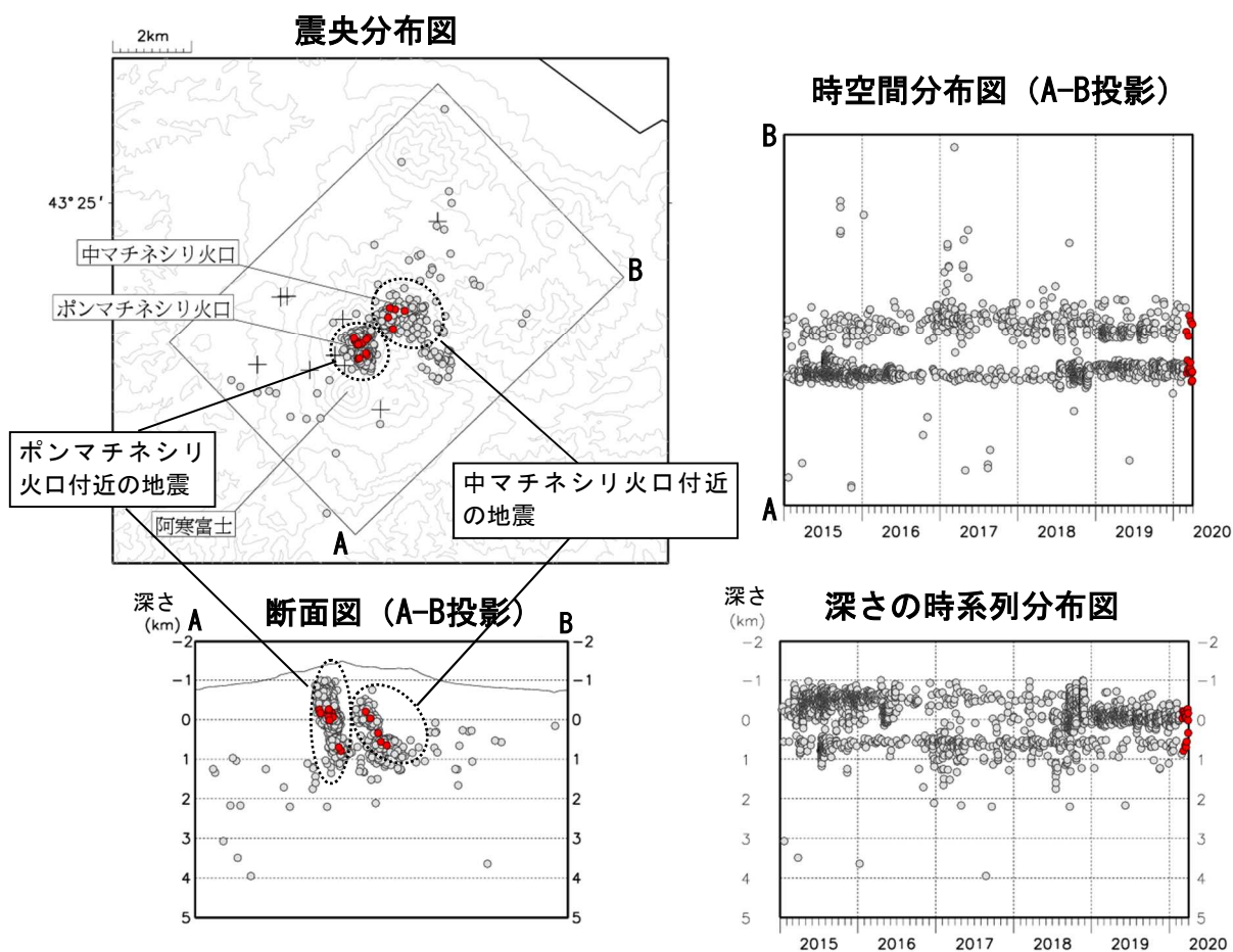
図6 雌阿寒岳 火山性地震の震源分布（2015年1月～2020年3月）
