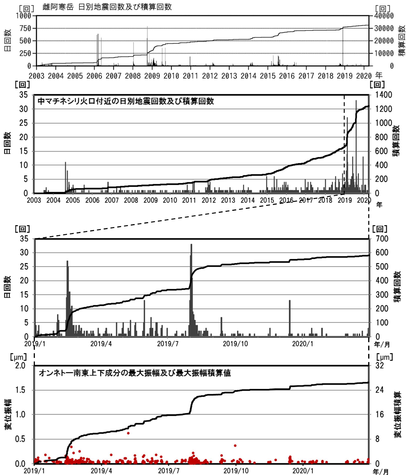
図5 雌阿寒岳 中マチネシリ火口付近の地震の日回数及び最大振幅
