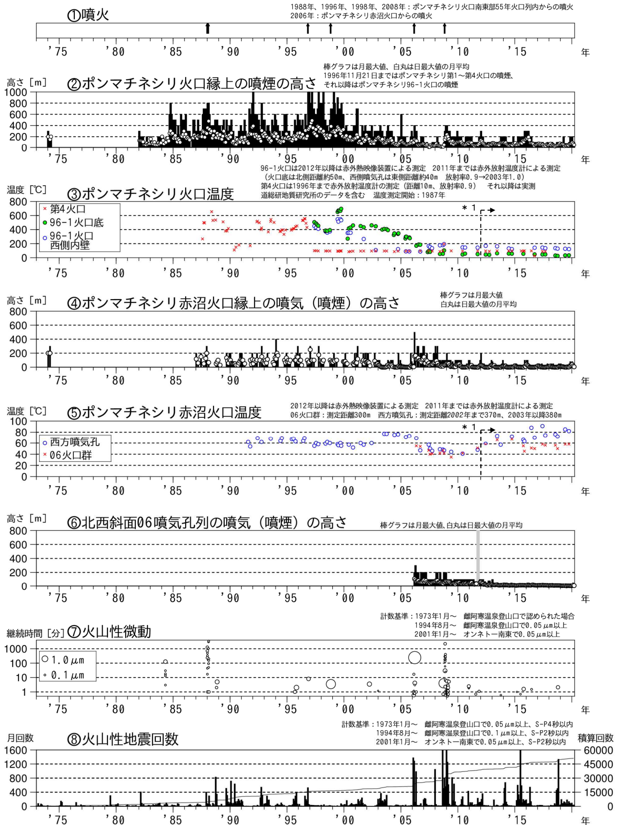
図1 雌阿寒岳 火山活動経過図（1973年1月～2020年3月）
