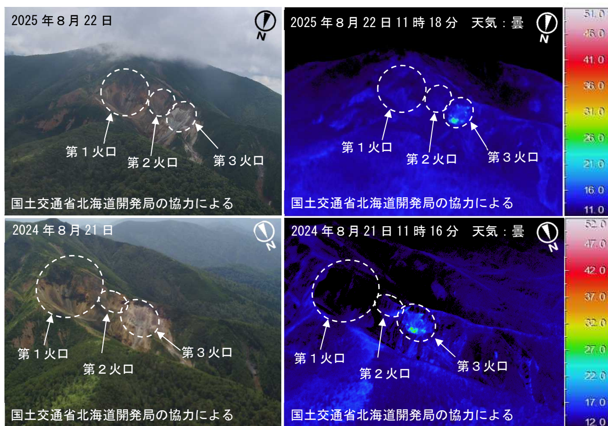
図3 丸山 赤外熱映像装置による第1火口～第3火口の地表面温度分布 北側上空（上段：図1の②、下段：図1の③）から撮影 ・前回の観測（2024年8月）と比べて、第3火口の地熱域（点線で囲まれた領域）の地表面温度分布に特段の変化はありませんでした。
