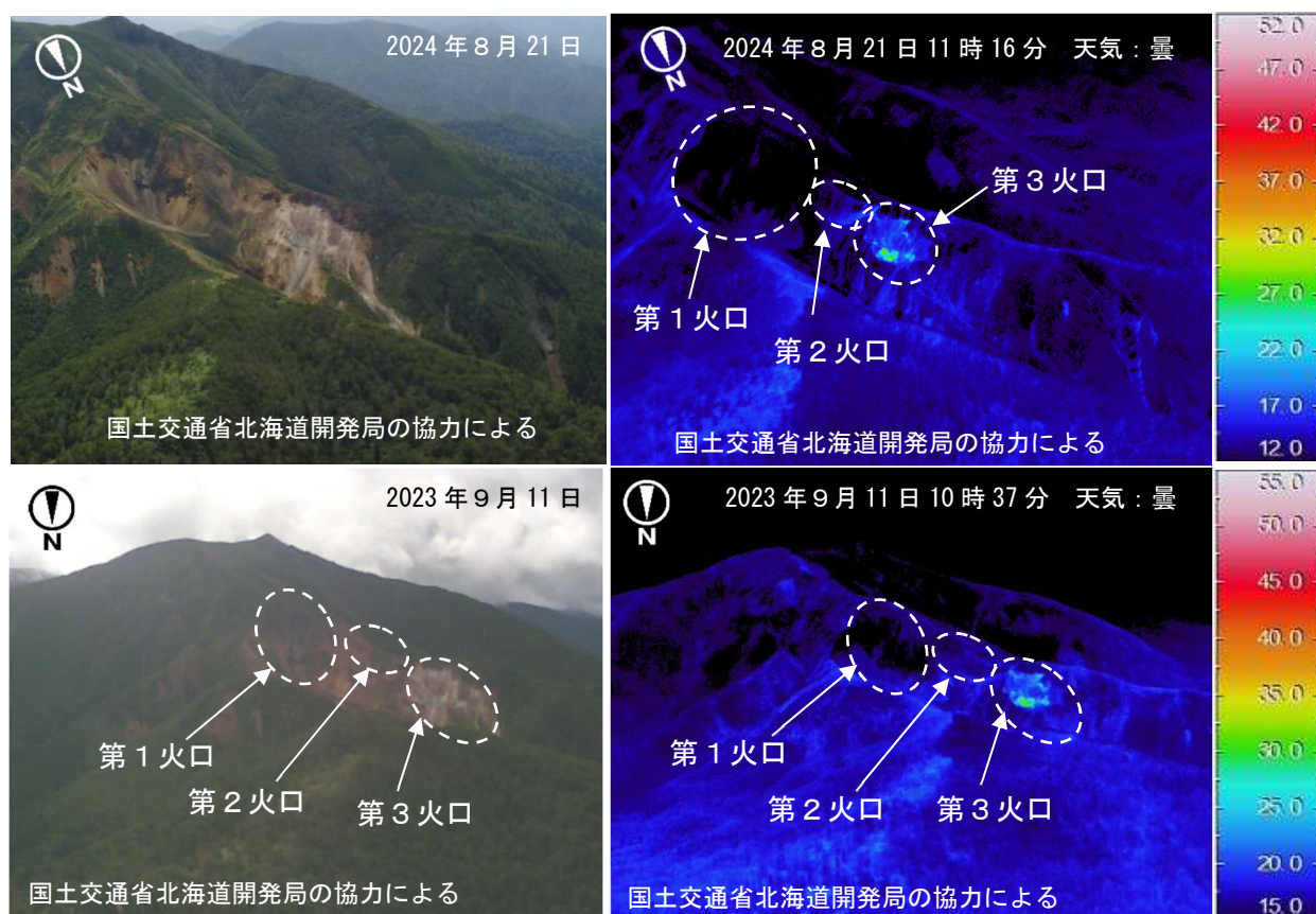
図3 丸山 赤外熱映像装置による第1火口～第3火口の地表面温度分布 上段：北東側上空（図1の①）から撮影 下段：北側上空（図1の②）から撮影 ・第3火口の地熱域（点線で囲まれた領域）の地表面温度分布は、前回の観測（2023年9月）と比べて特段の変化はありませんでした。
