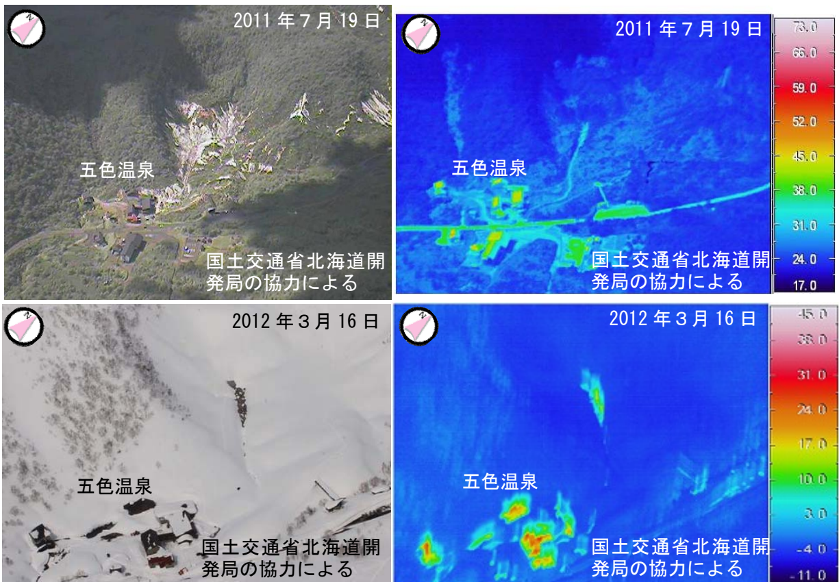
図3 ニセコ 五色温泉付近の地表面温度分布 1) 南東側上空（図1-②の矢印方向）から撮影
