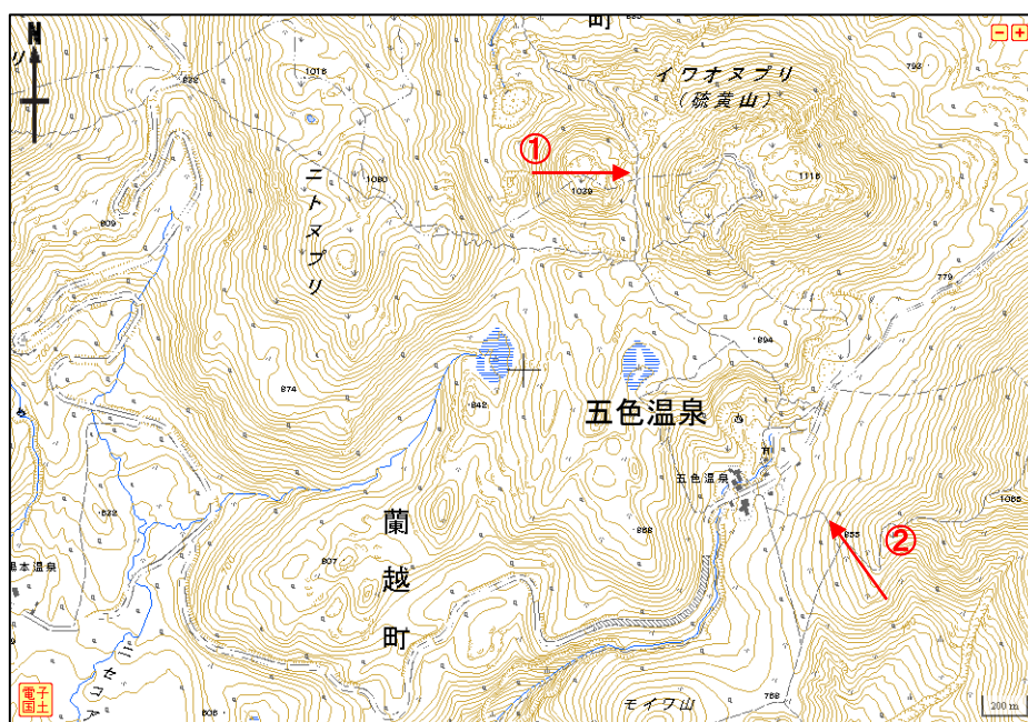
図 1 ニセコ 周辺図と赤外熱映像 1) 及び写真の撮影方向
