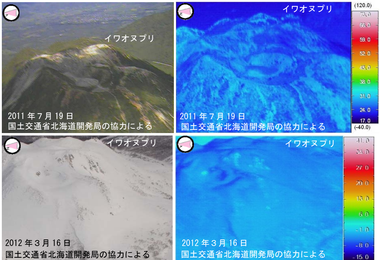
図2 ニセコ イワオヌプリ山頂の地表面温度分布 1) 西側上空（図1-①の矢印方向）から撮影
