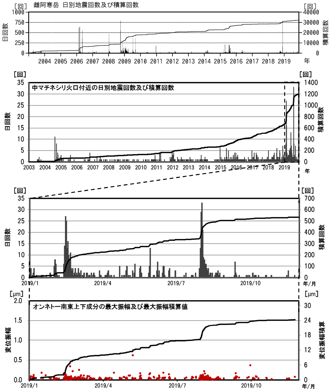
図5 雌阿寒岳 中マチネシリ火口付近の地震の日回数及び最大振幅（2003年1月～2019年11月）
