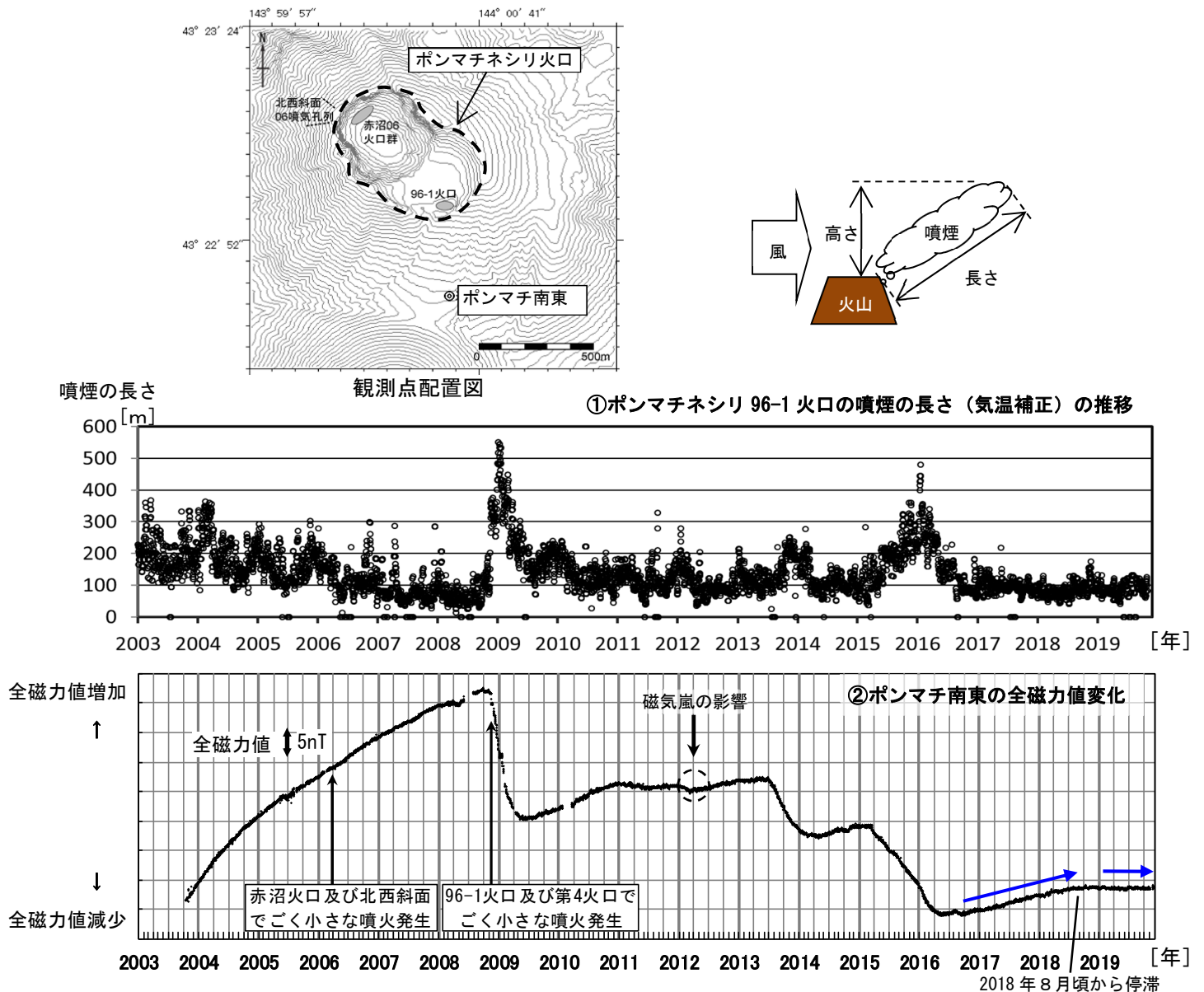
図4 雌阿寒岳 ポンマチネシリ96-1火口の噴煙の長さ（気温補正）の推移及び全磁力観測点配置図
