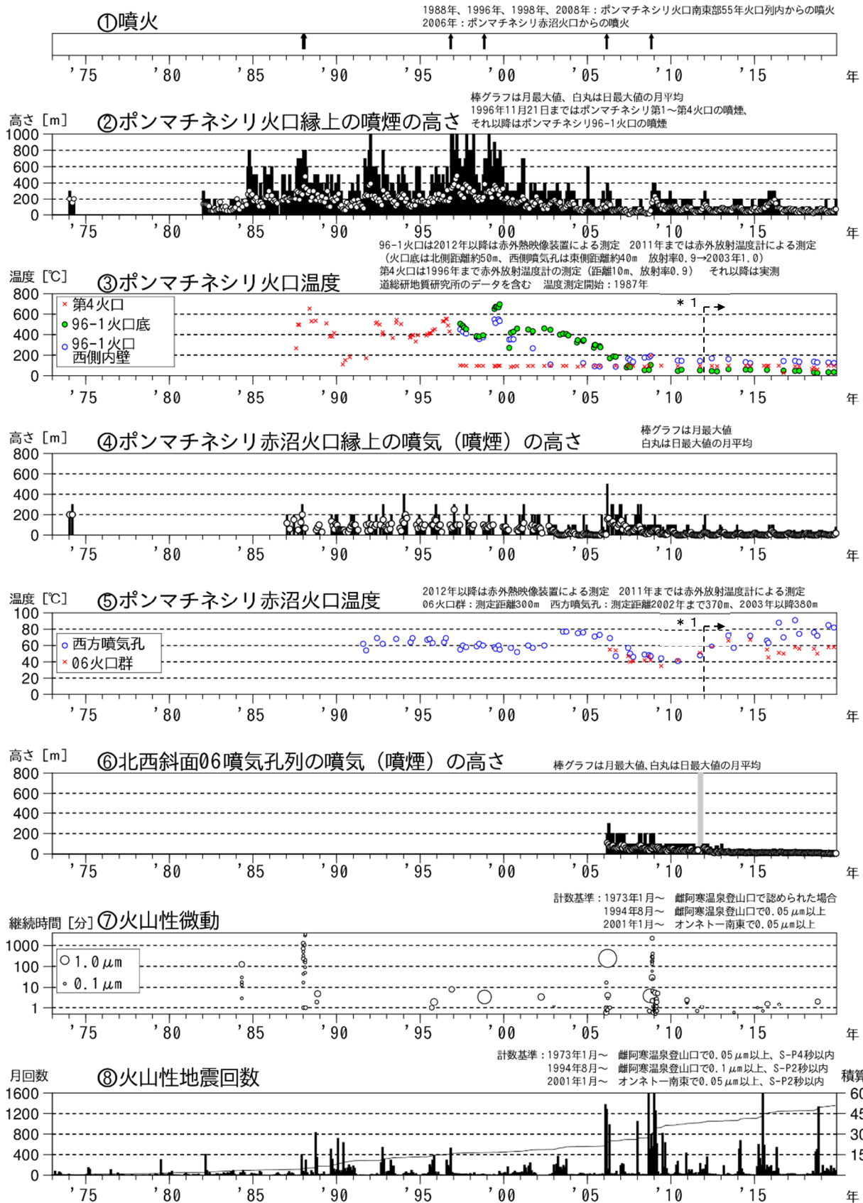
図1 雌阿寒岳 火山活動経過図（1973年1月～2019年11月）
