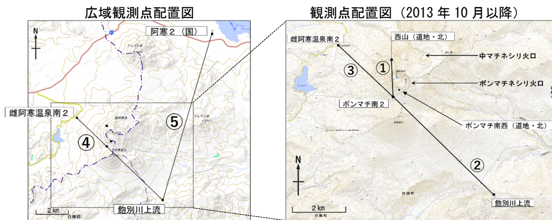
図 7 雌阿寒岳 GNSS連続観測による基線長変化（2006年 4 月～2019年11月）及び観測点配置図
