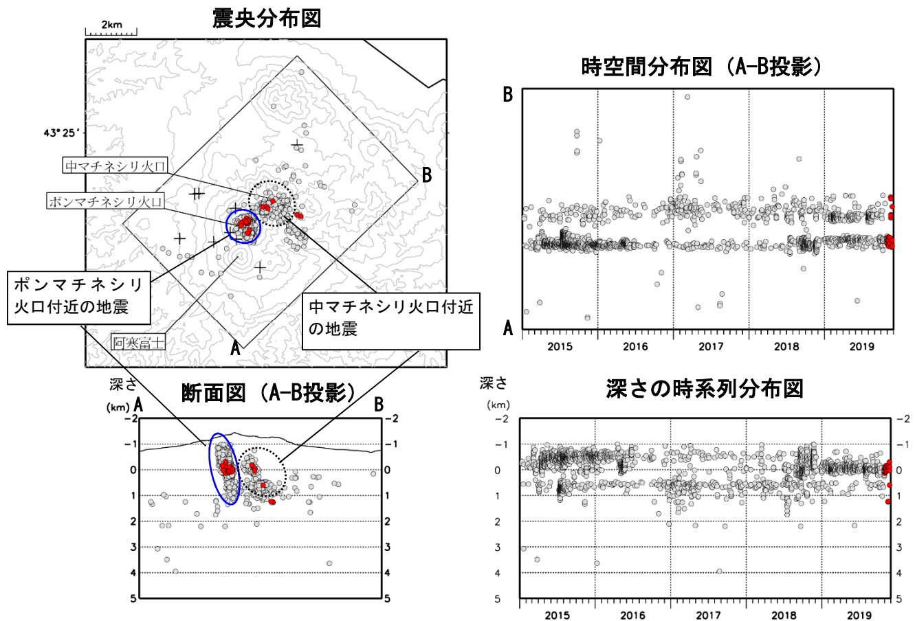
図6 雌阿寒岳 火山性地震の震源分布（2015年1月～2019年11月）
