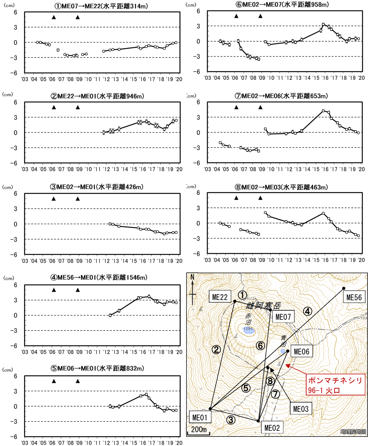
図8 雌阿寒岳 GNSS繰り返し観測によるポンマチネシリ火口付近の水平距離変化及び観測点配置 (2003年7月～2019年10月)
