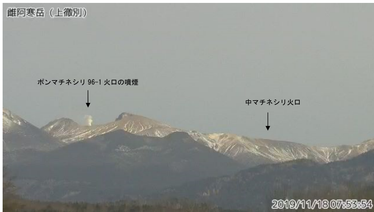
図3 雌阿寒岳 南東側から見た山体の状況 かみてしべつ (11月18日、上徹別監視カメラによる)
